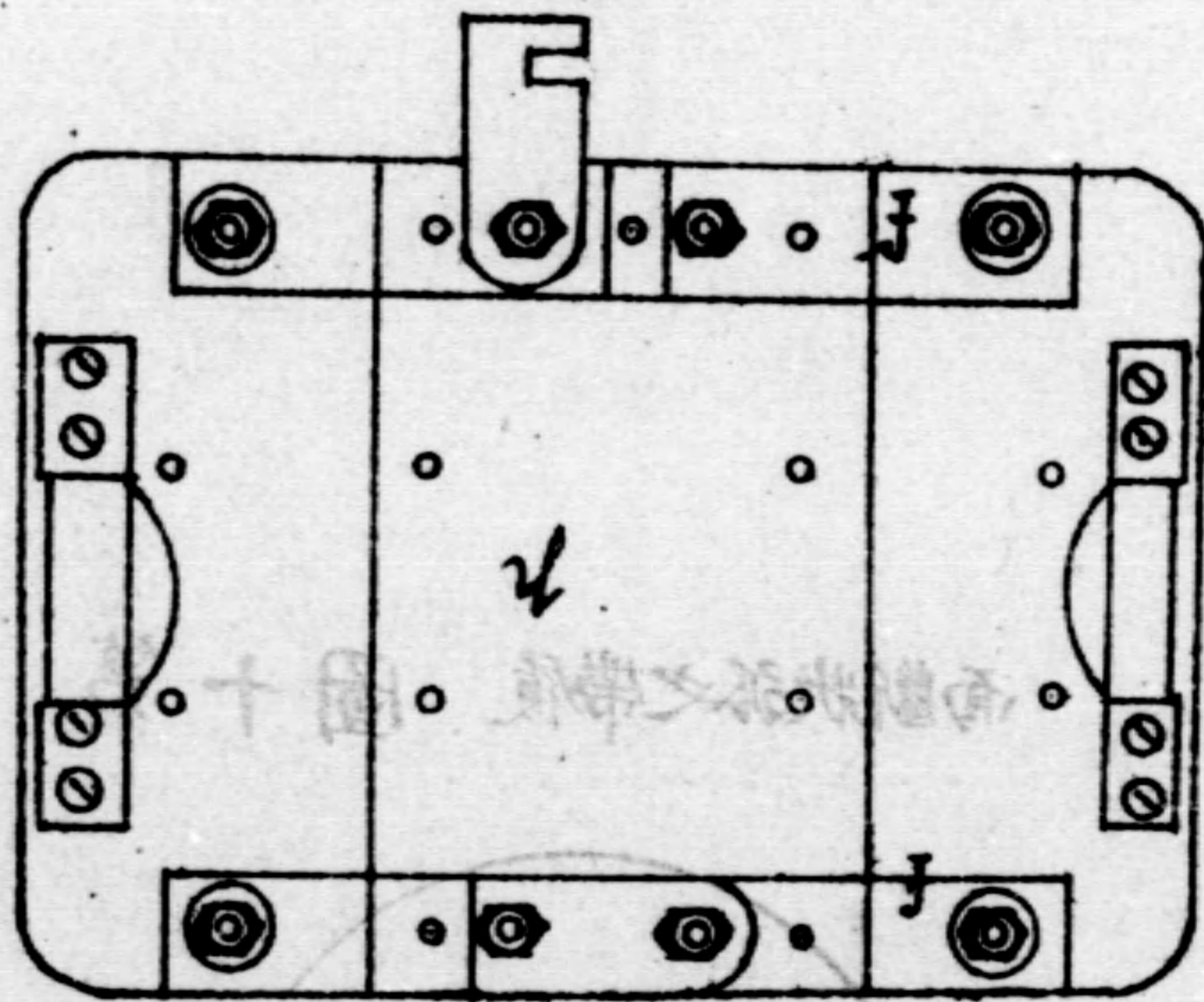
第 七 圖 履 鋏 (平 面)
