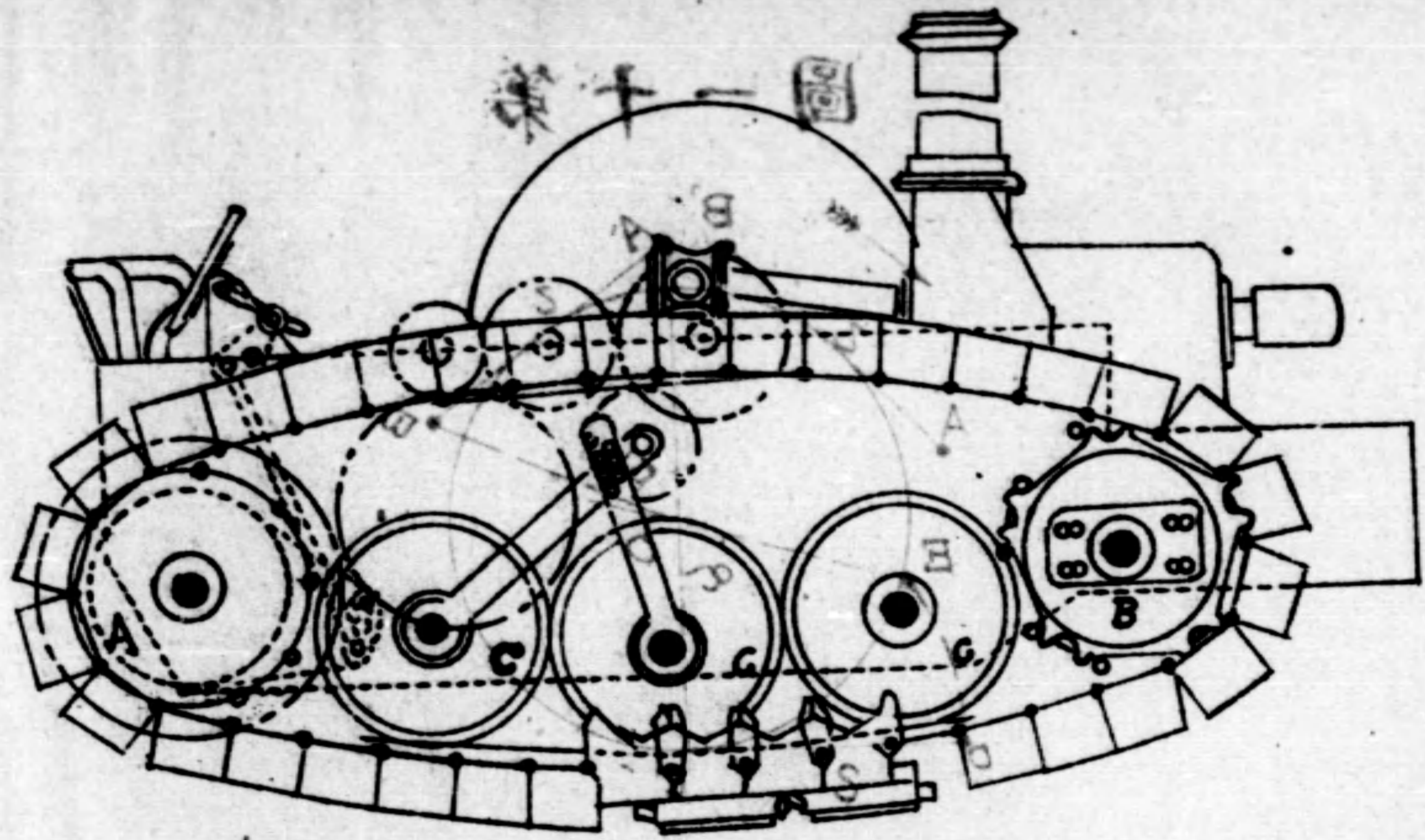
機引牽「皮斯龍屋」圖一十二第
