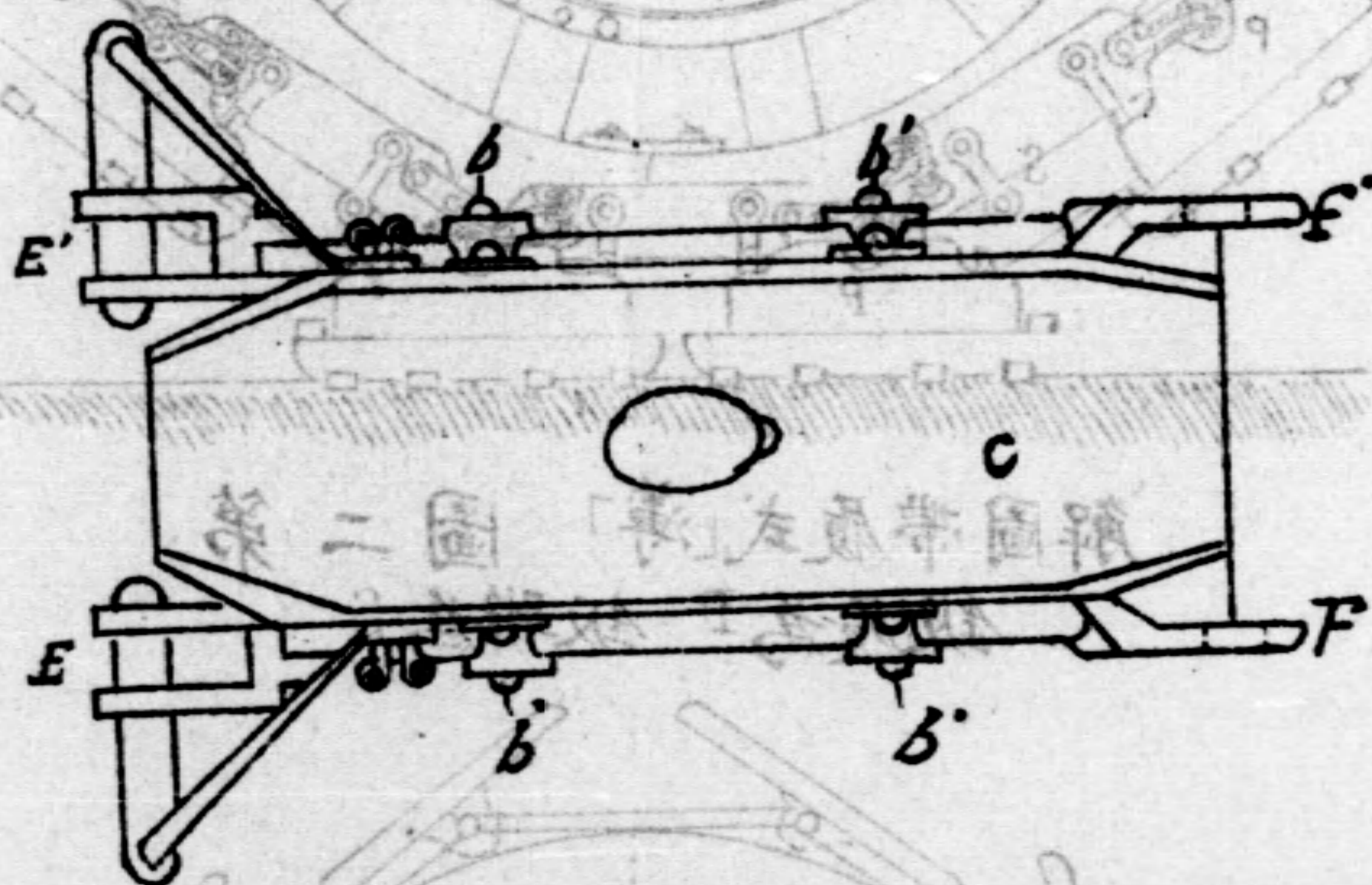
(面平)鉸聯 圖四第
