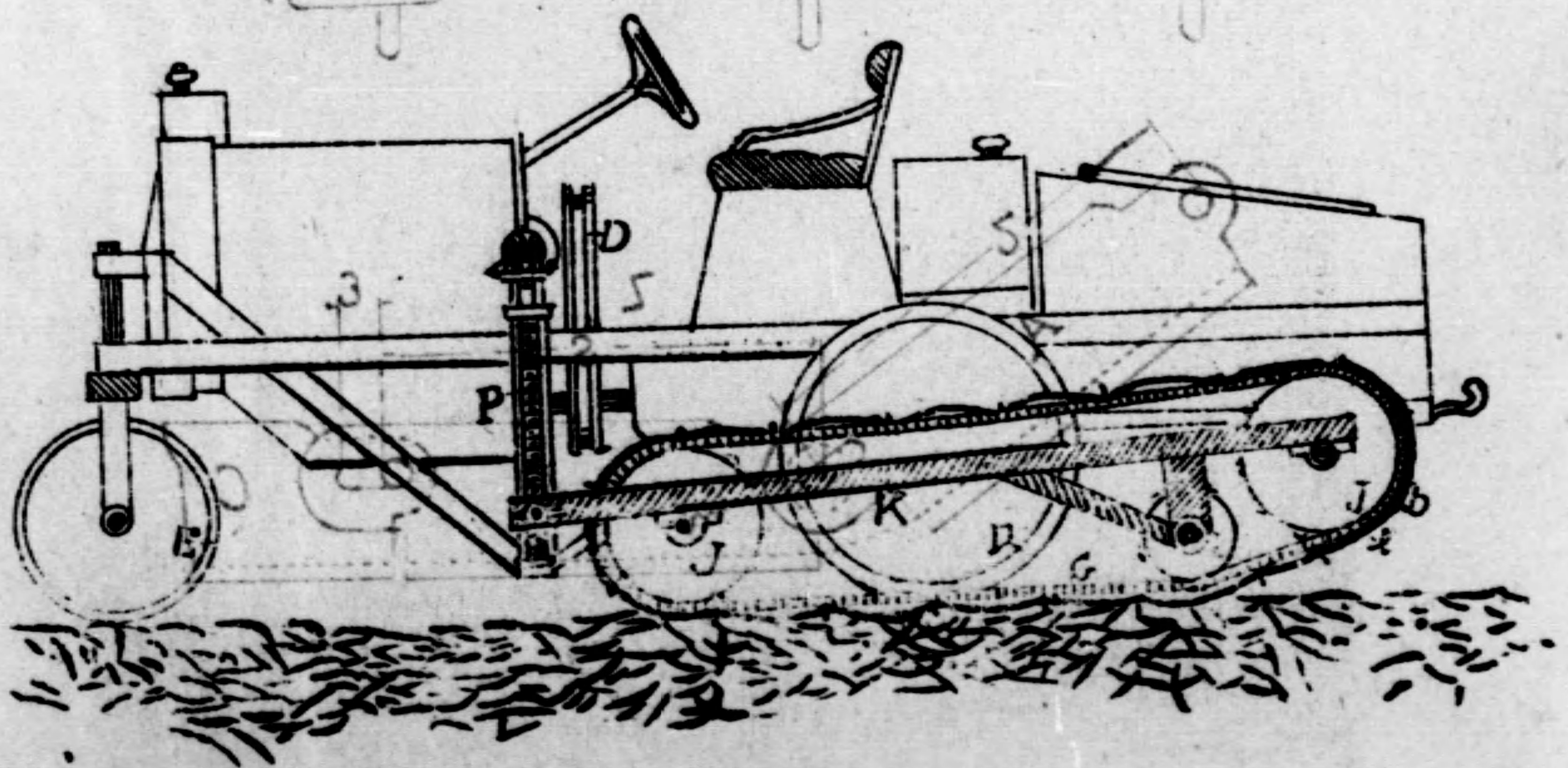
機引牽「安路」圖三十二第
