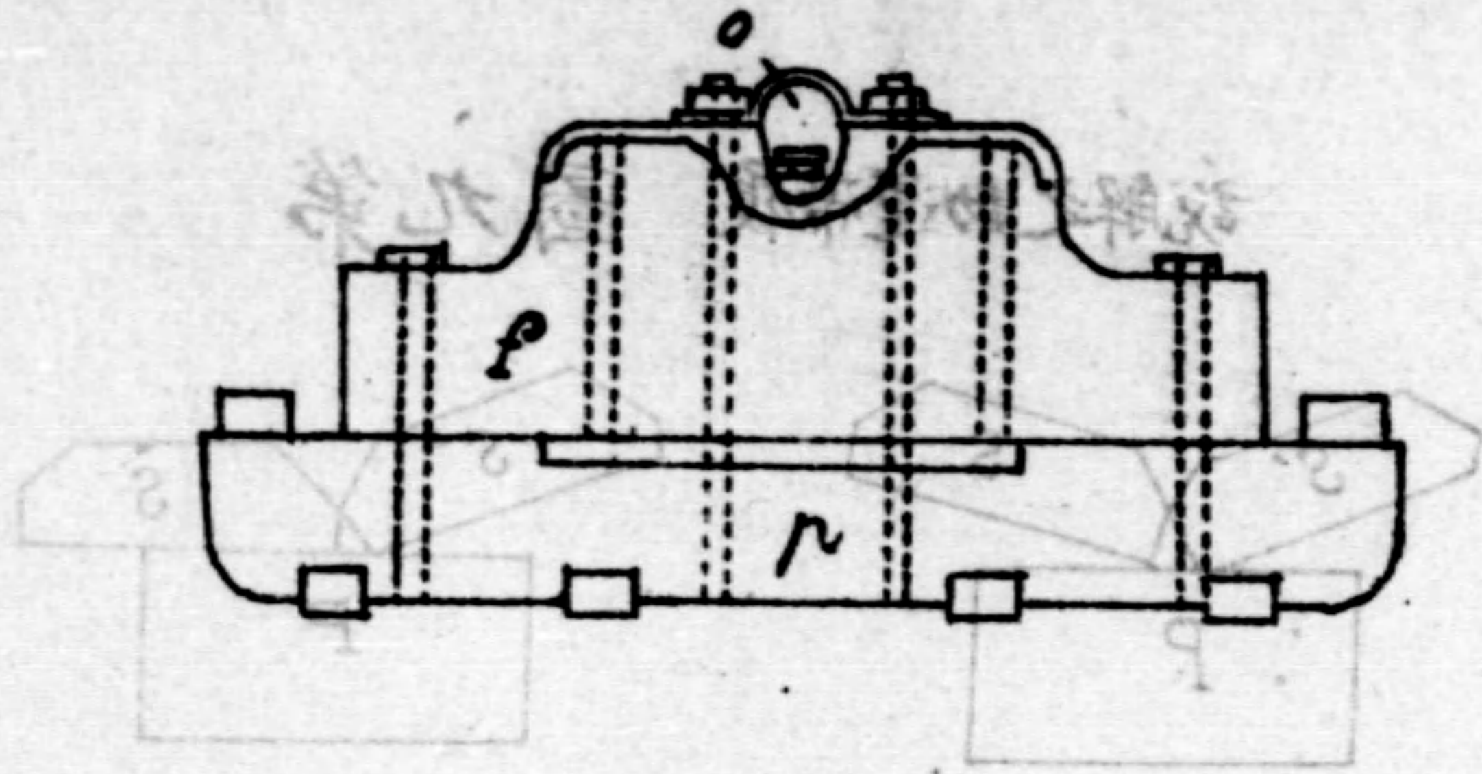
第 六 圖 履 鋏 (側 面)
