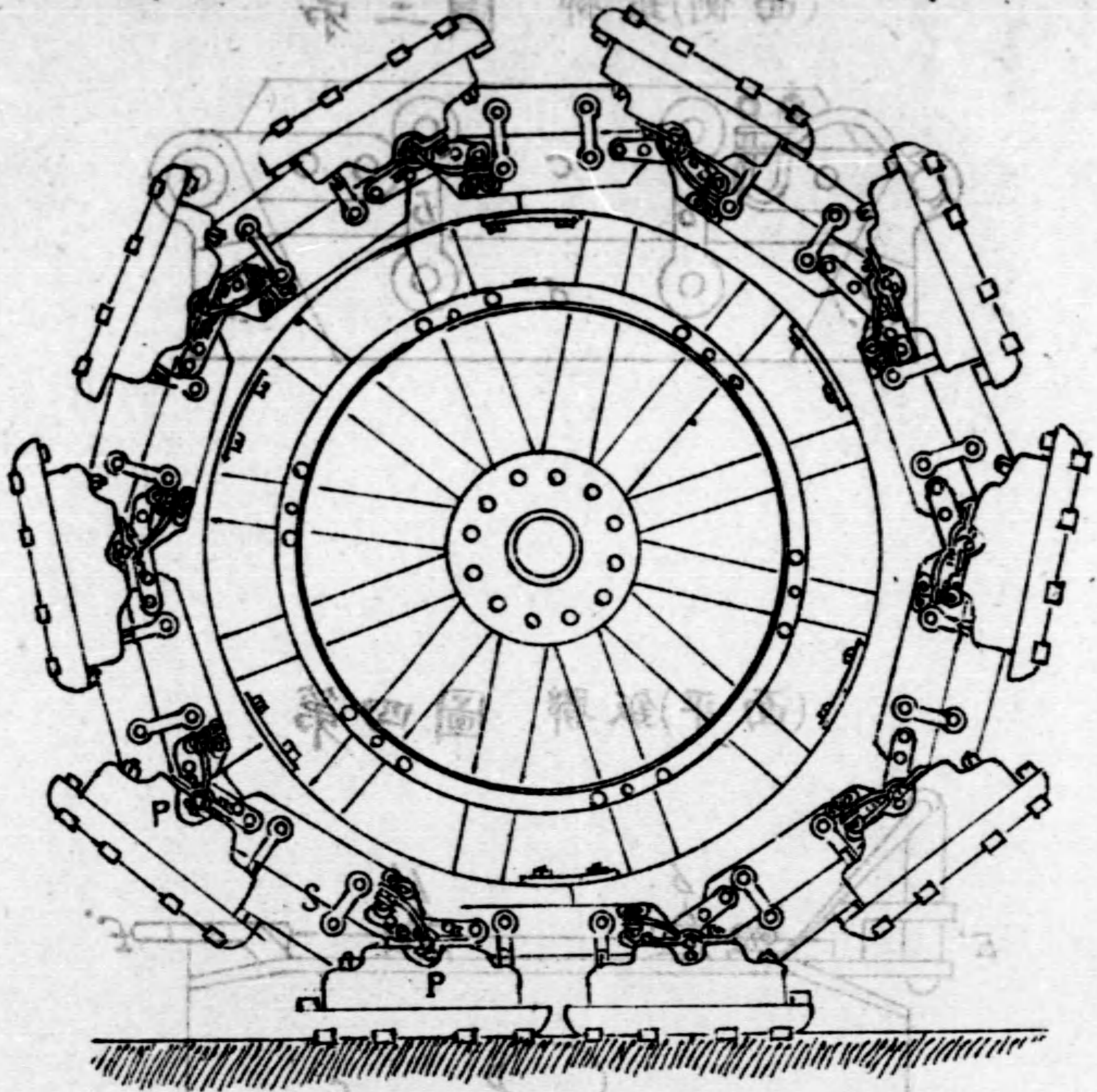
第二圖 薄式履帶圖解
