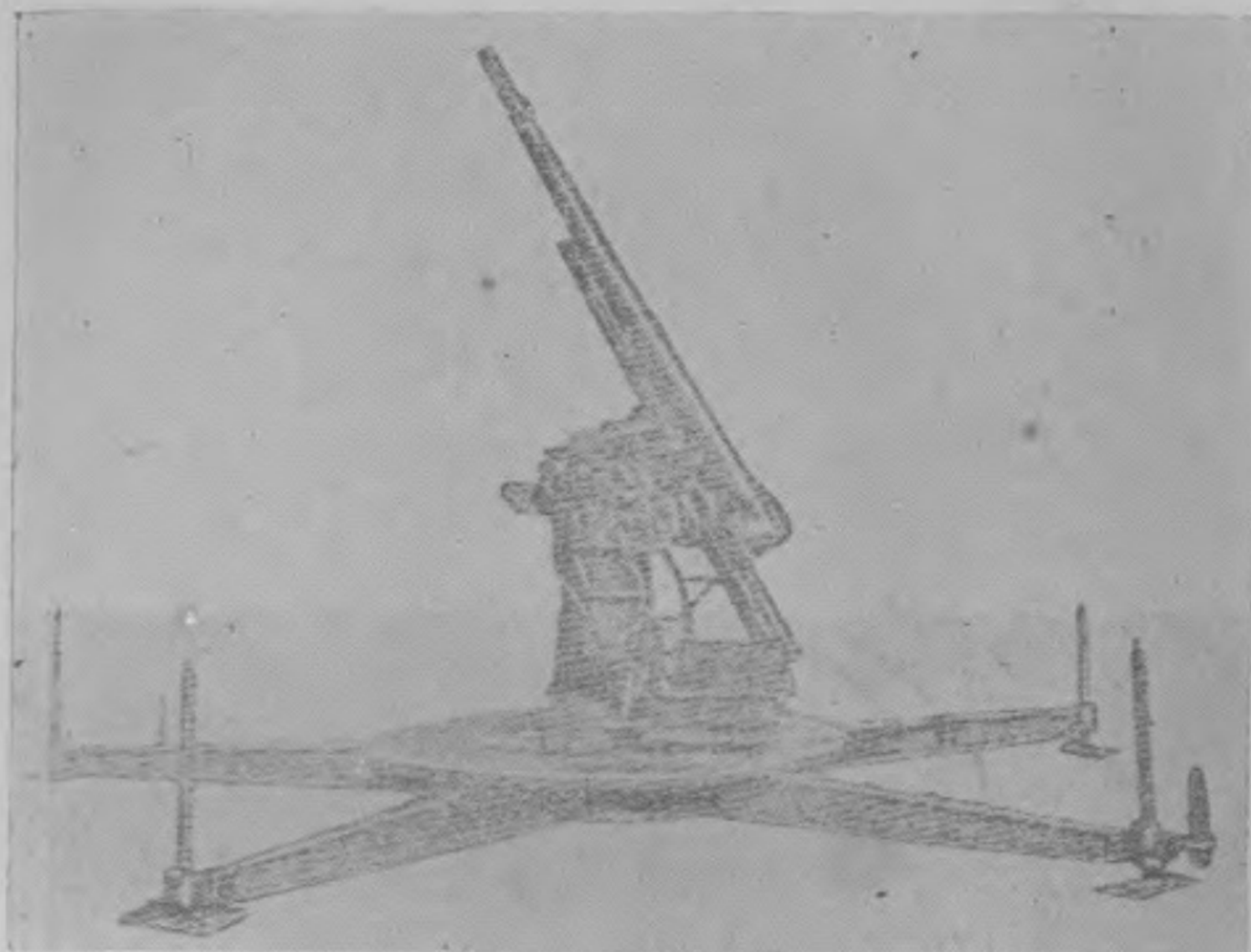
防空高射砲
