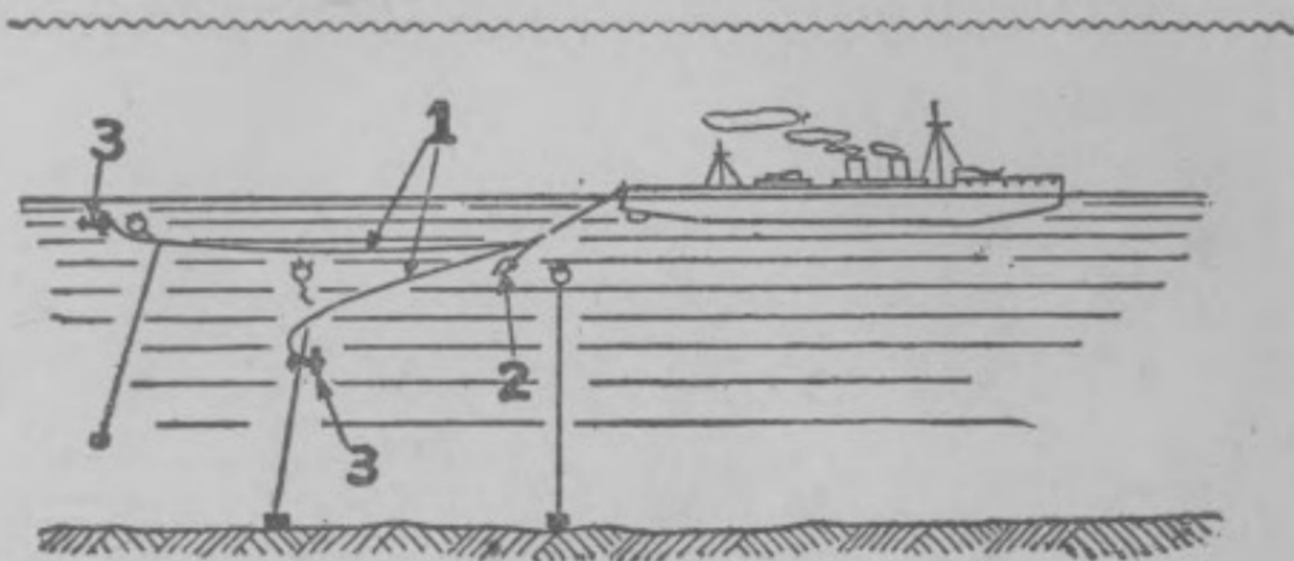
對艦掃海的狀態(1.掃海索, 2.浮標, 3.沈降器)
