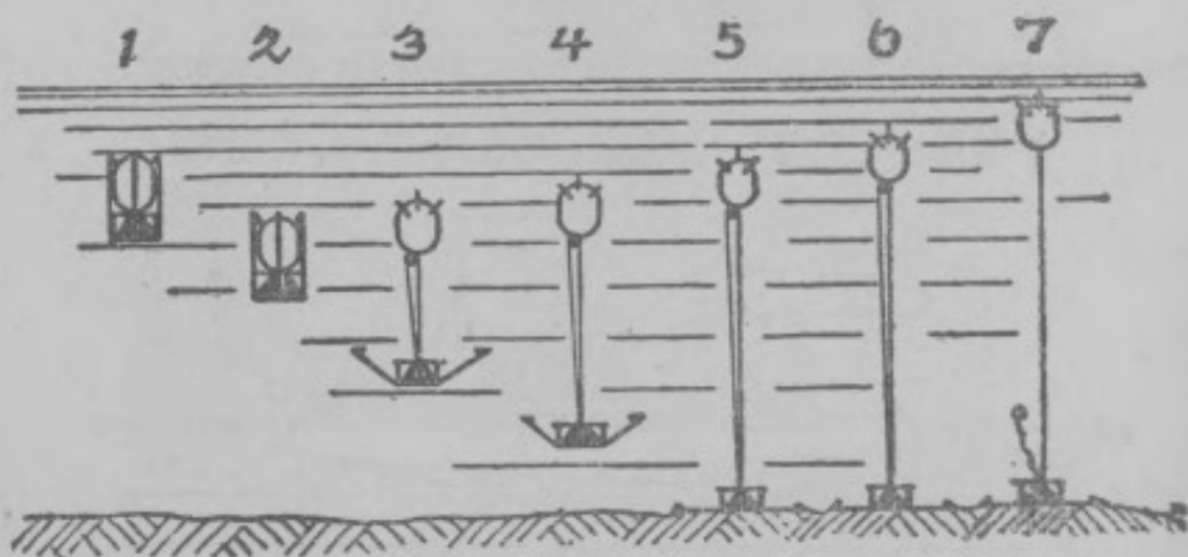
潛水艦艇所用繫留機雷的敷設狀態
