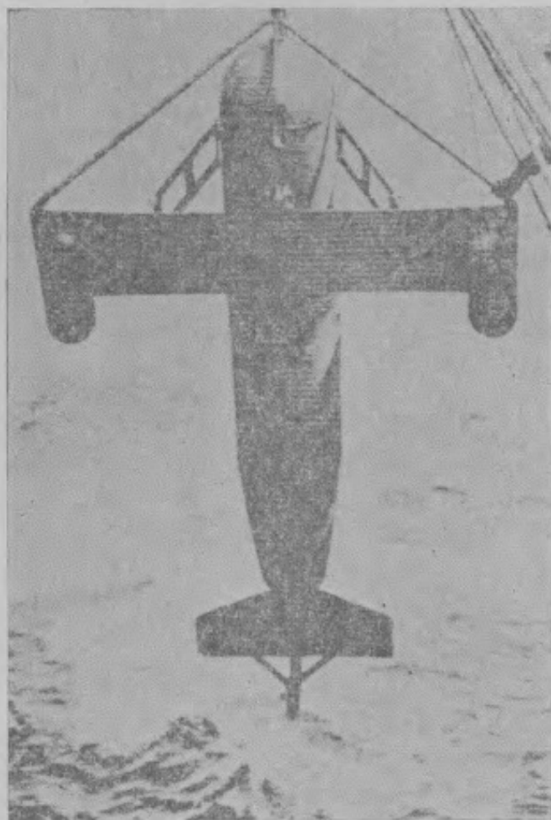
防 雷 具 ( 即 展 開 器 )
