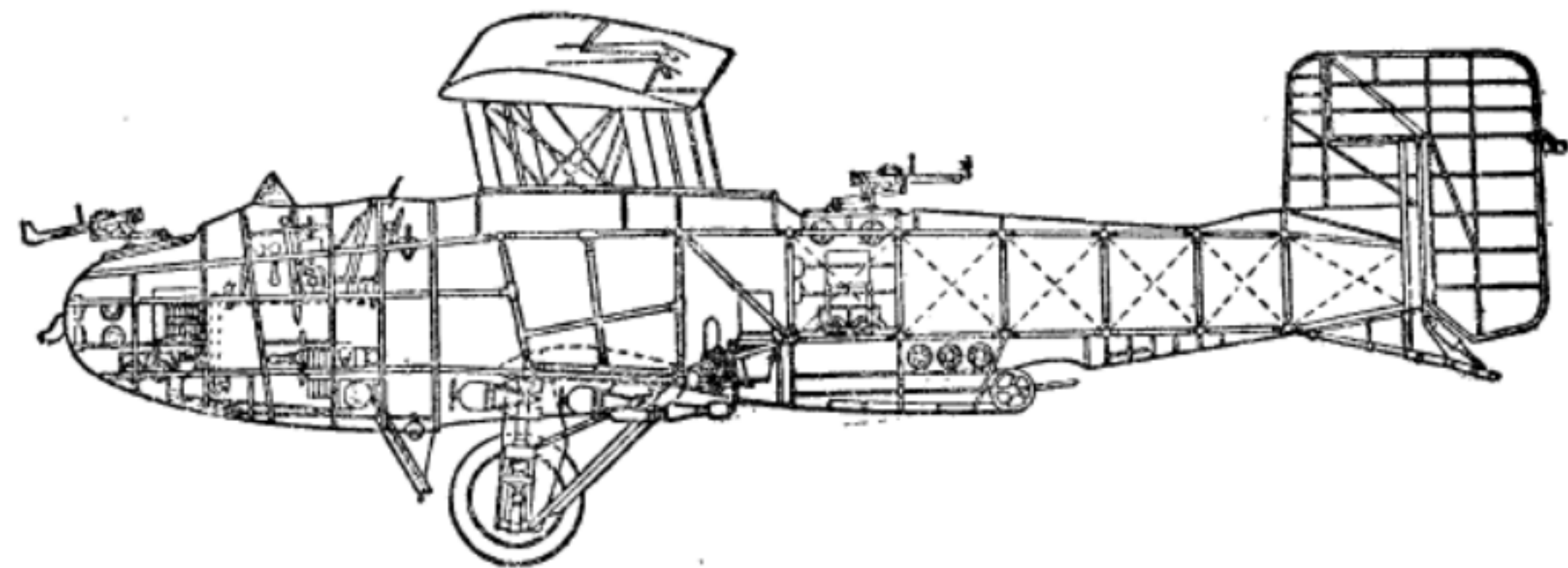
英國布爾頓·保爾(Boulton & Paul)“Sidestrand”轟炸機的裝備 (上圖為側面,下圖為縱剖面)
