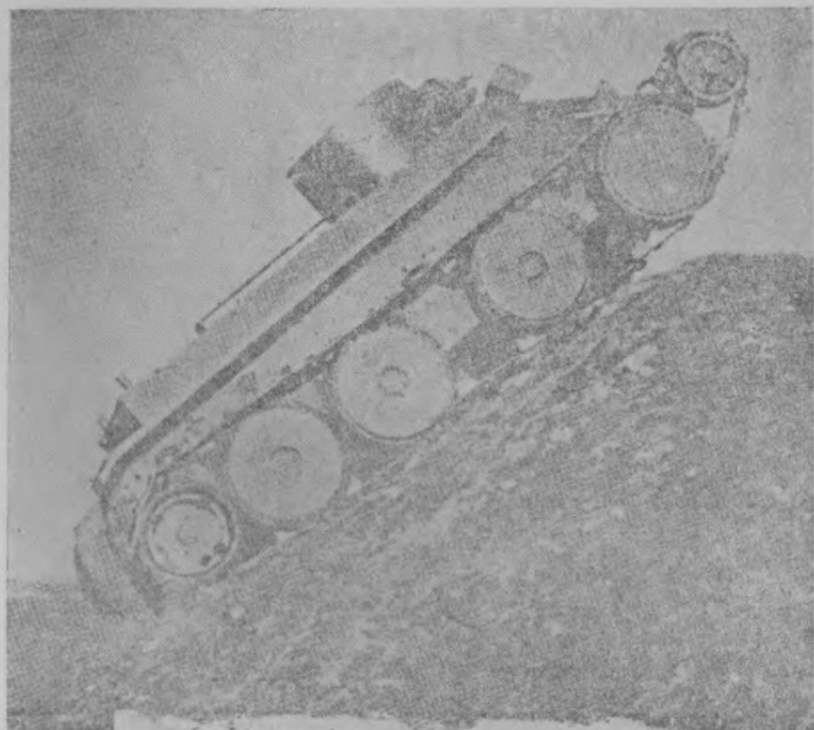
戰車在山坡上之行進
