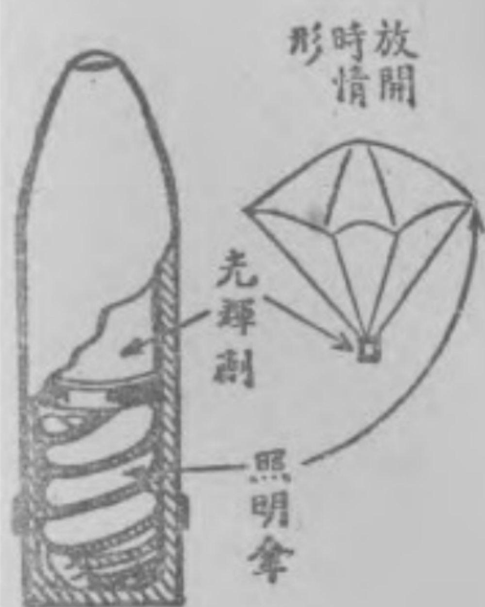
照明彈
