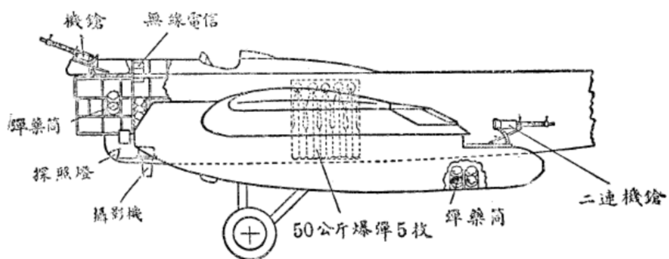
法國勃萊列奧 (Blériot) 127 式轟炸機的裝備
