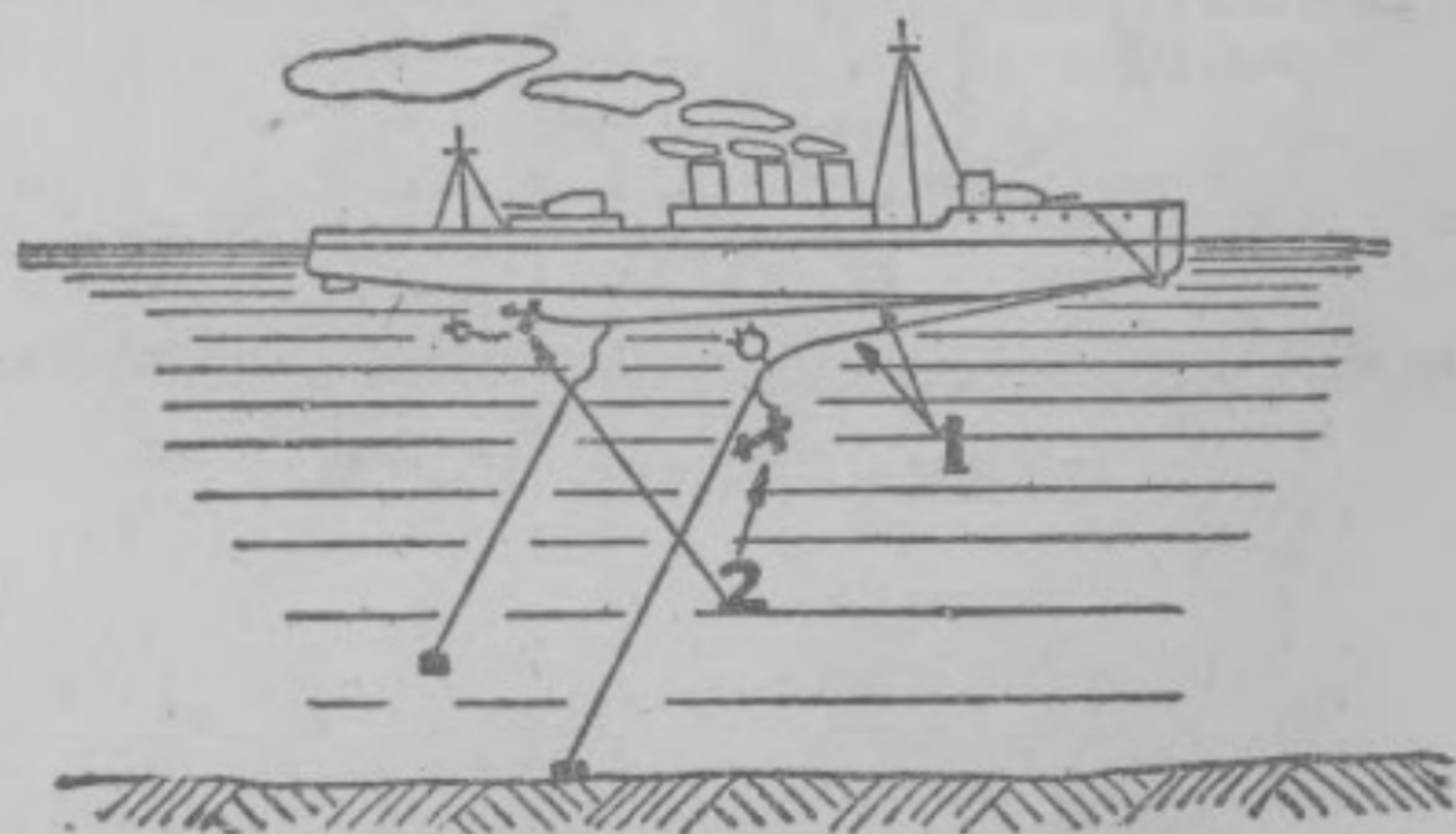
防雷具曳航的狀態(1.曳索, 2.展開器)
