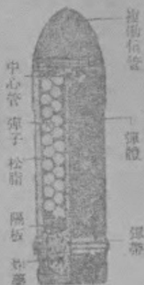
榴霰彈
