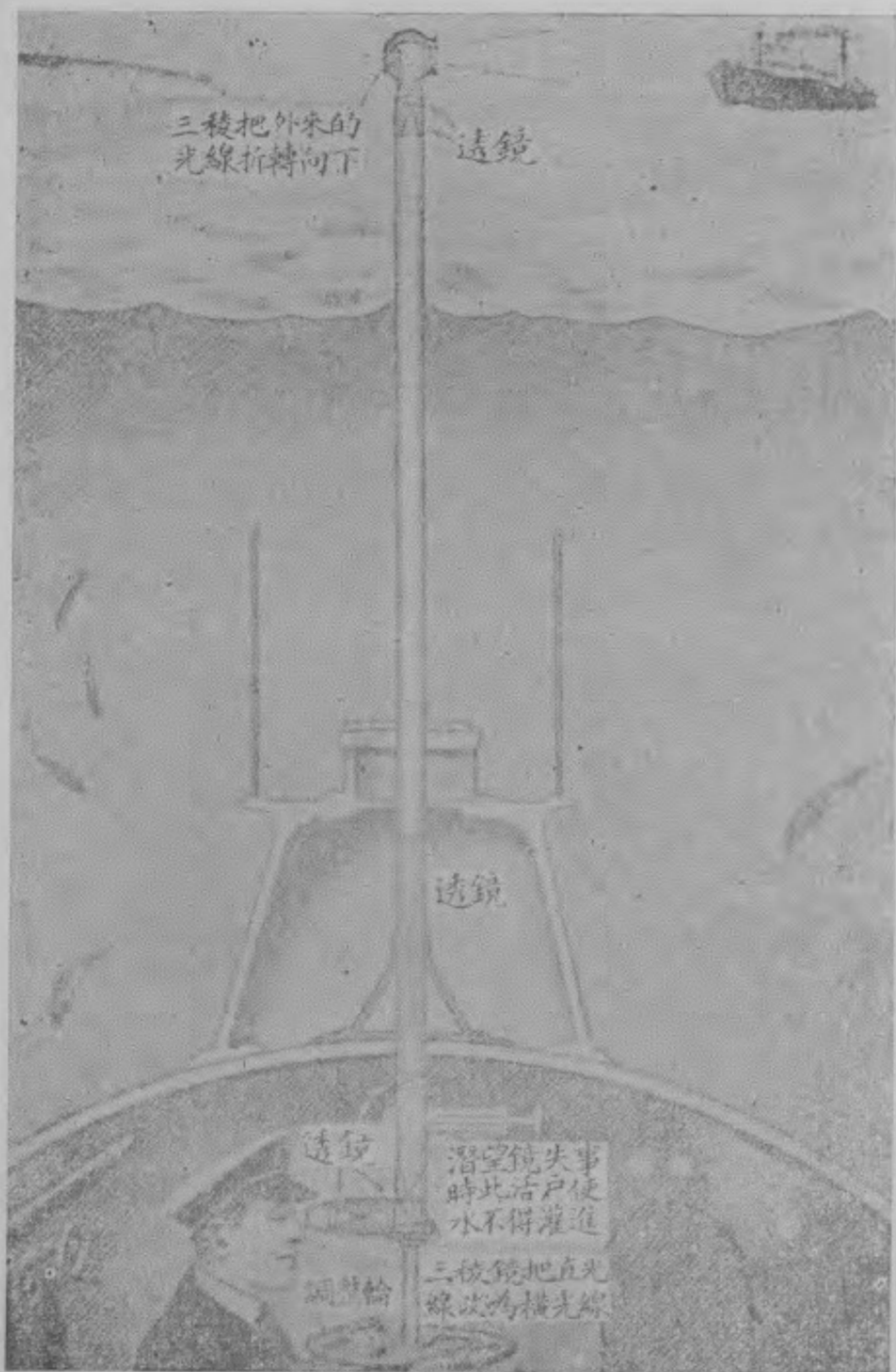
潛望鏡的構造
