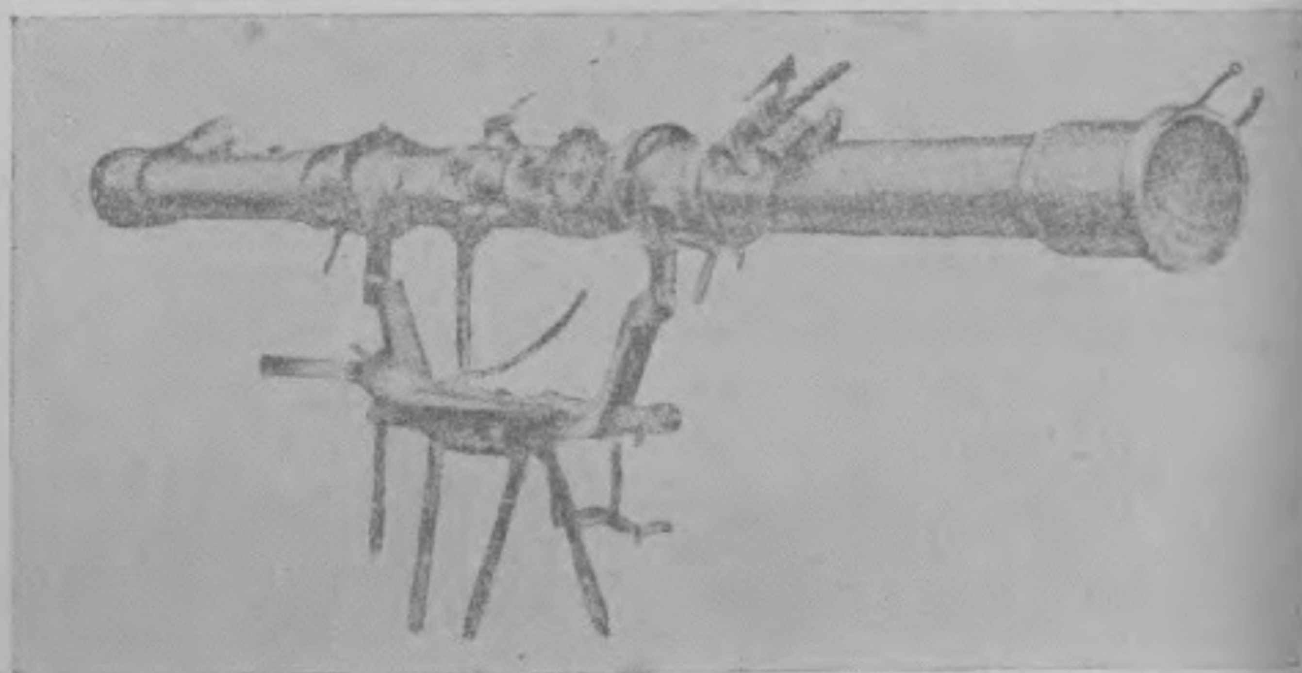
測距儀(斯的利奧式)
