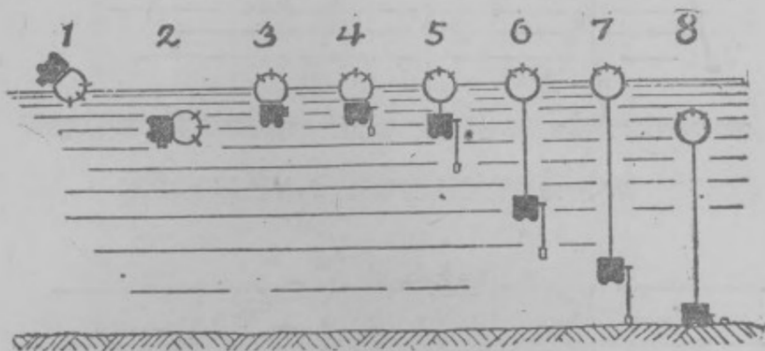
水上艦艇所用繫留機雷的敷設狀態
