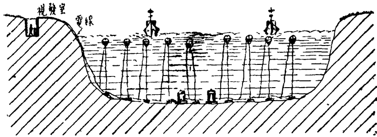
水雷佈置實寫
