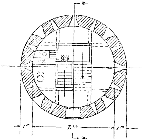
平 面
