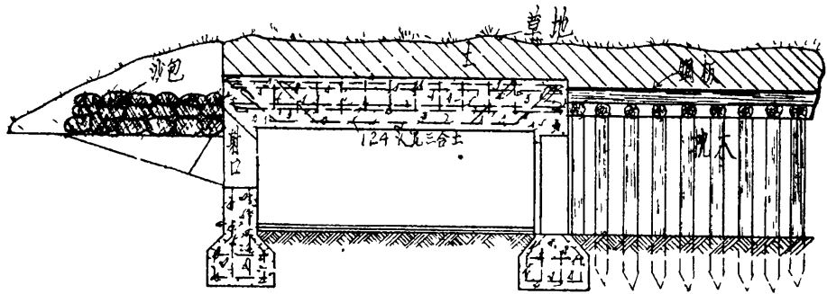
A-A 剖面
