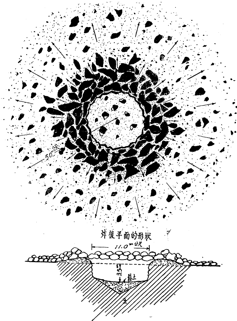
炸 後 情 形 剖 面
