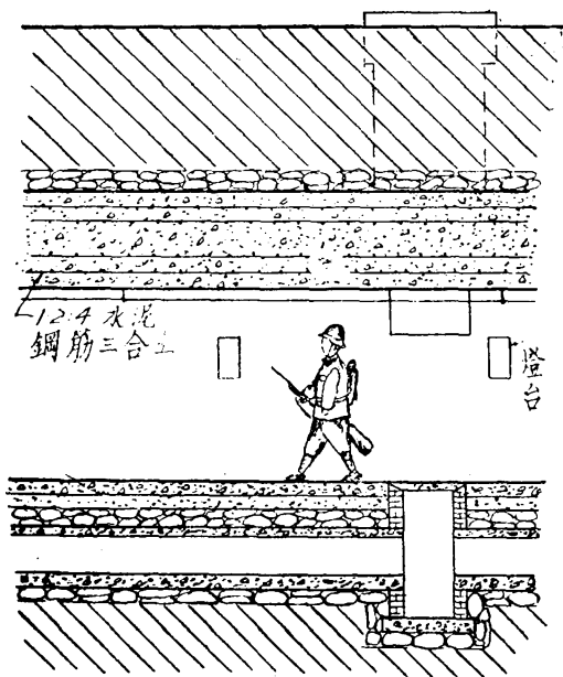
縱剖面
