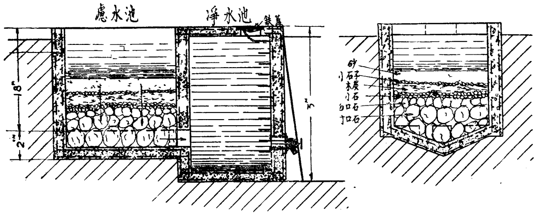
濾水池剖面
