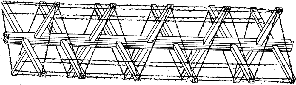
拒馬構造圖
