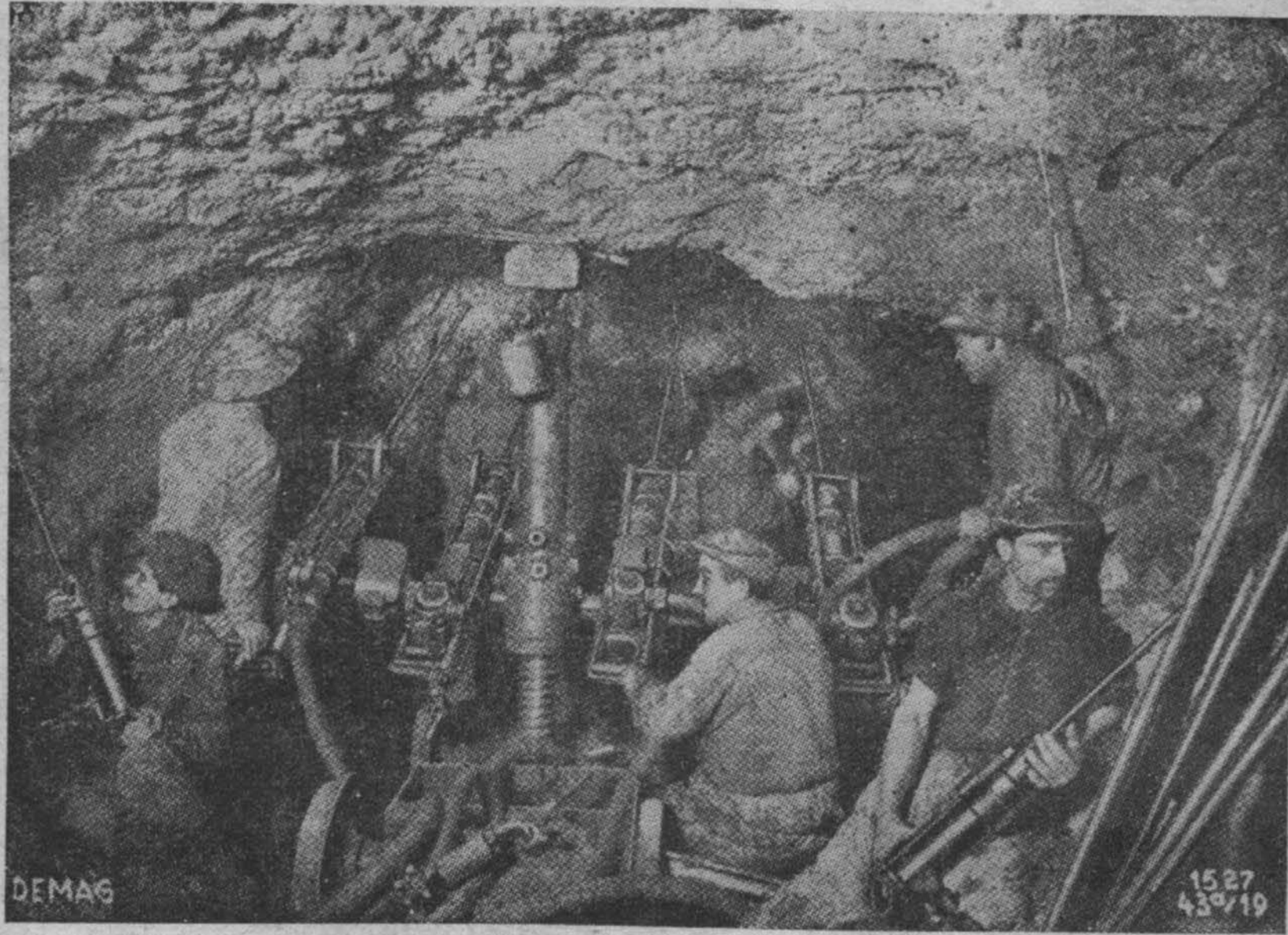
德 國 用 機 械 開 鑿 山 洞 圖
