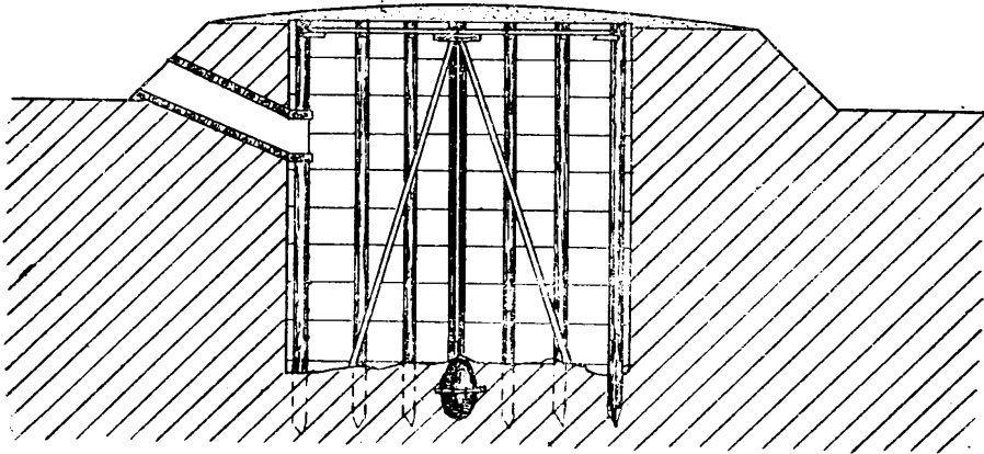
陷 阱 構 造 圖
