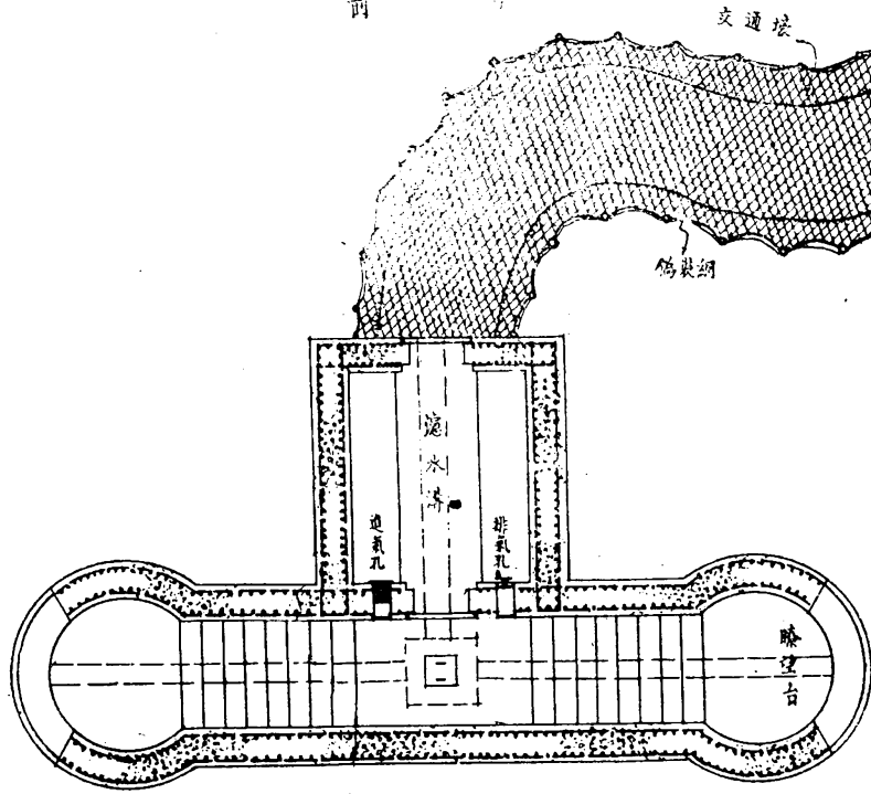
平 面
