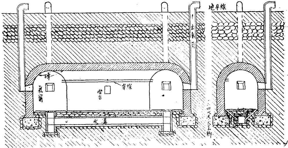
A-A 剖面
