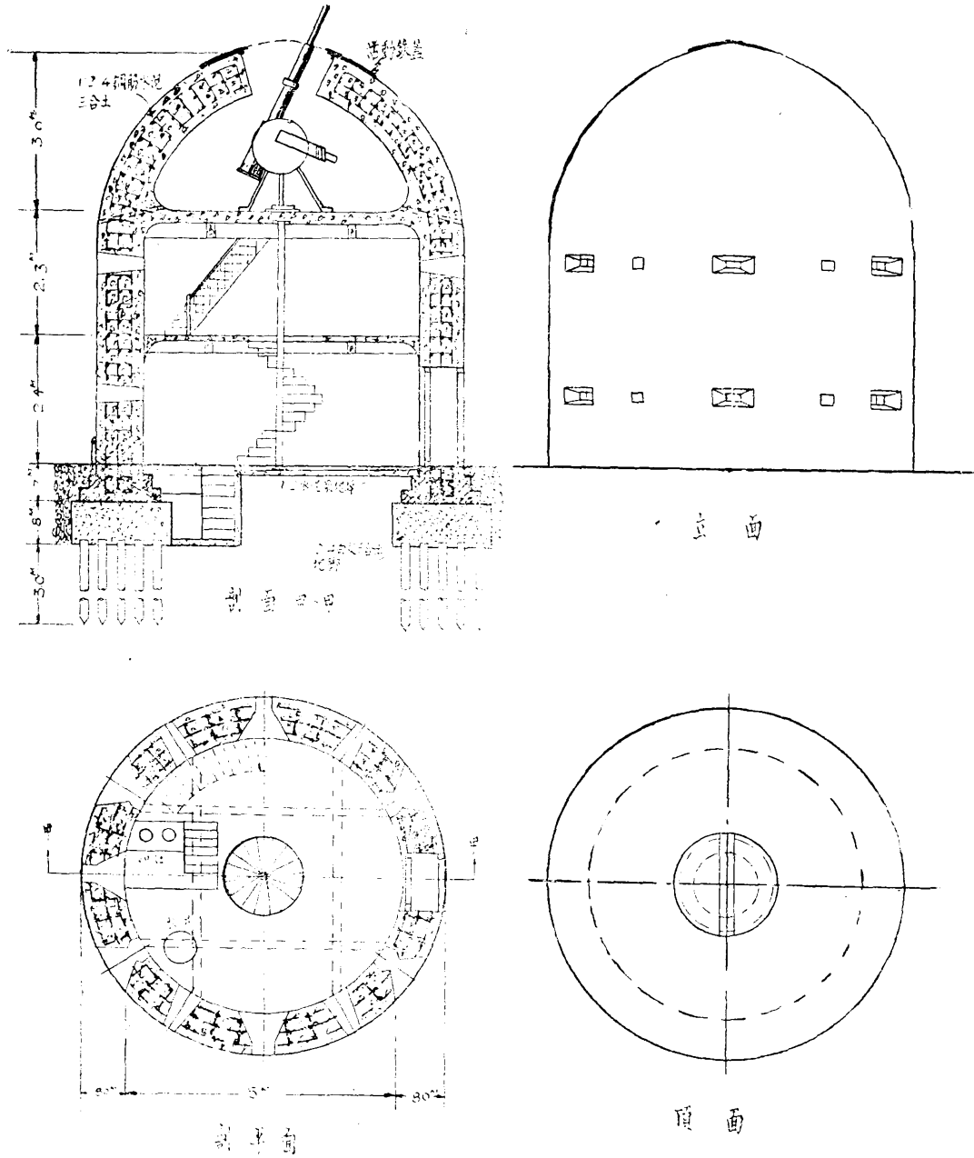
圓堡構造圖
