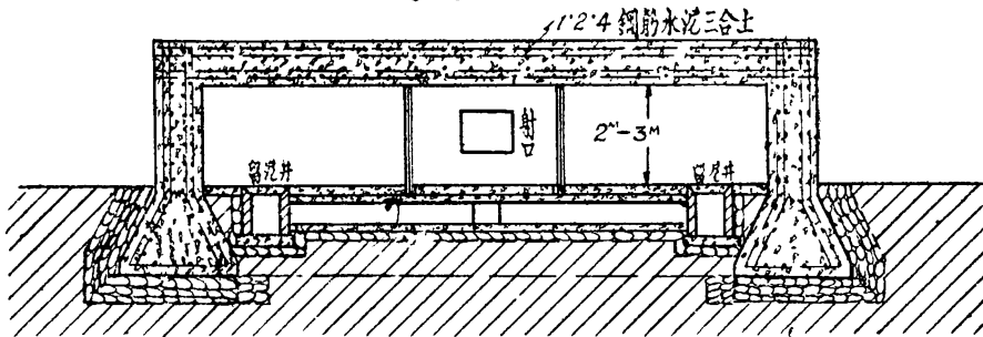
乙-乙剖面
