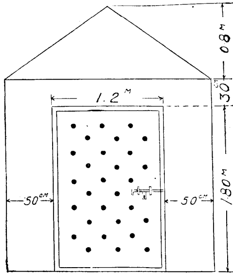
門的正視
