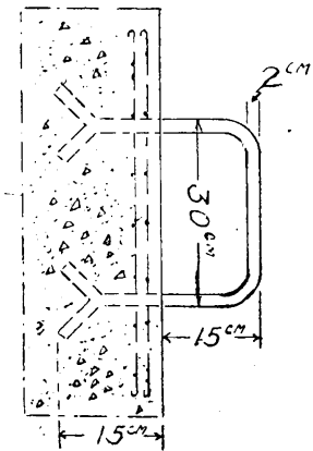
扒梯平視
