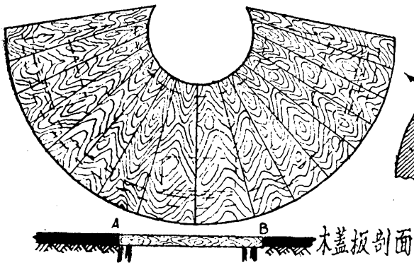
駐鋤坑蓋板
