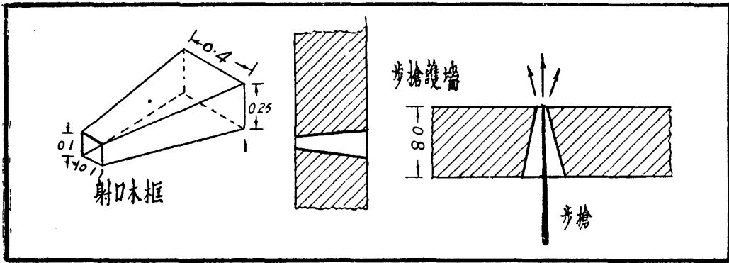
步槍射口
