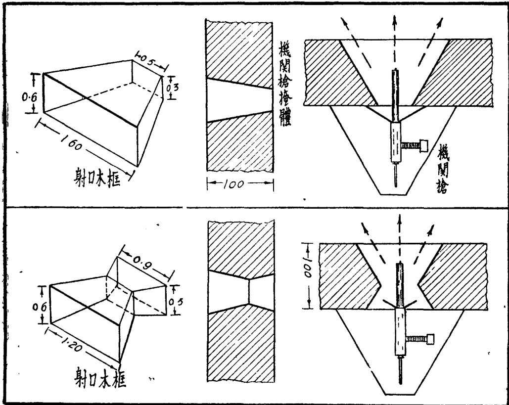
機關槍射口
