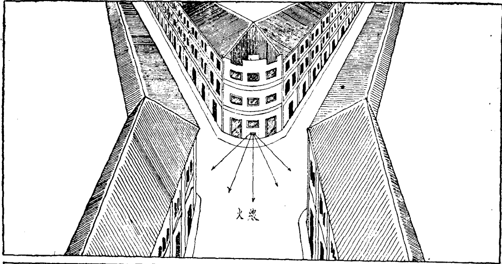
三义路口巷戰機關槍掩體建在屋內圖
