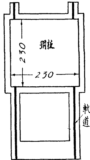
剖面乙-乙
