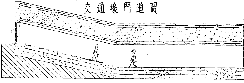
樓 梯 踏 步
