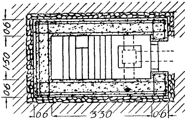
剖面甲-甲
