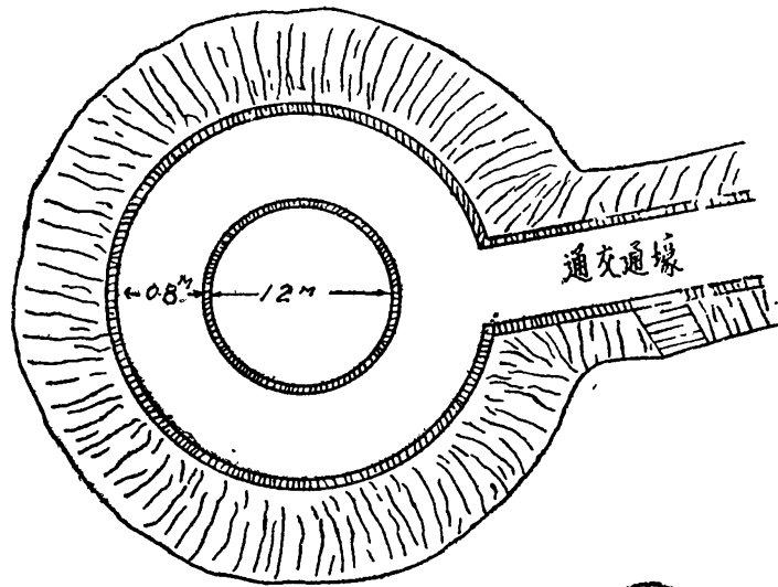
平 面
