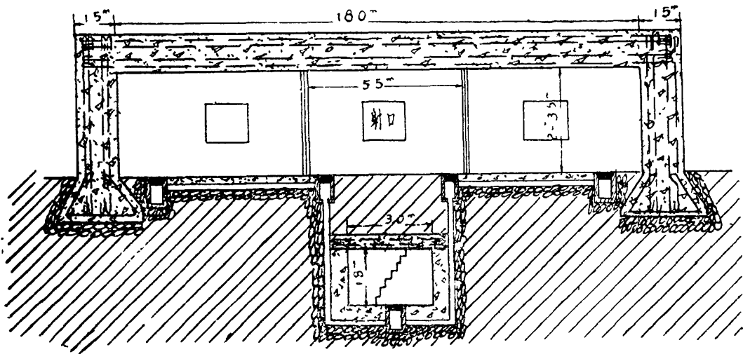
乙-乙剖面
