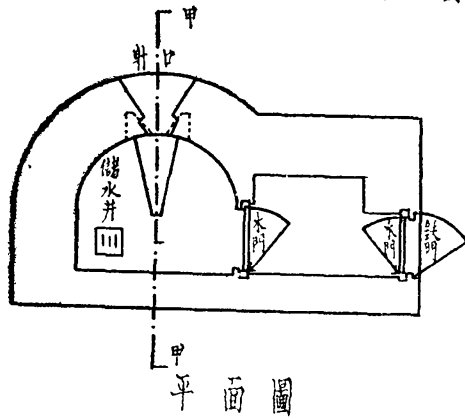
鋼筋水泥三合土機閘掩體圖
