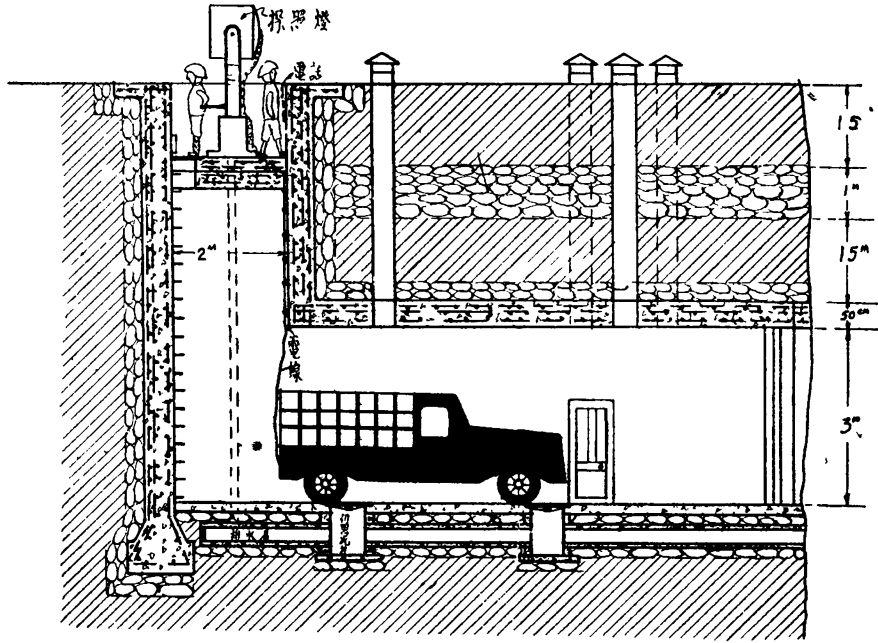
探照燈掩體構造圖 · 無蓋式
