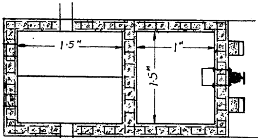
平面
