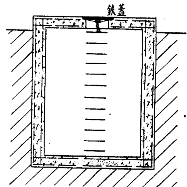
淨水池断面
