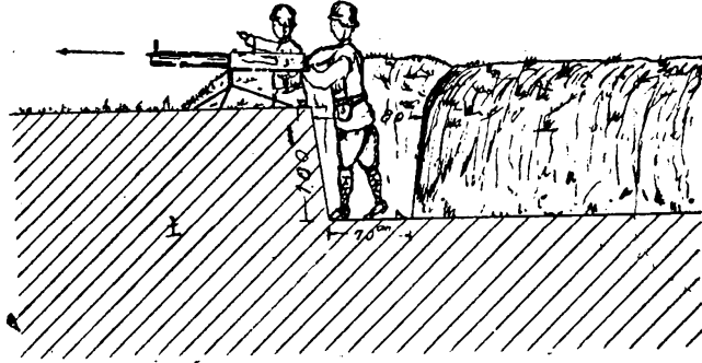
剖 視
