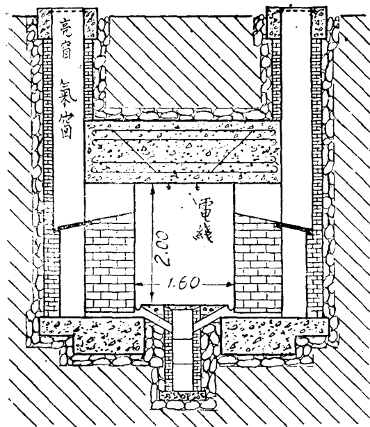
橫剖面
