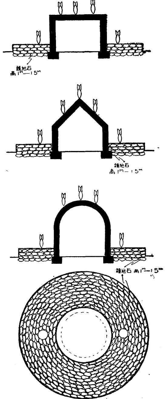
有側防的掩體
