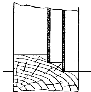
木 檻 大 樣
