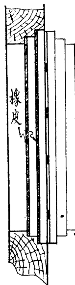
A—A 剖面
