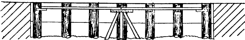
架 板 構 造 圖
