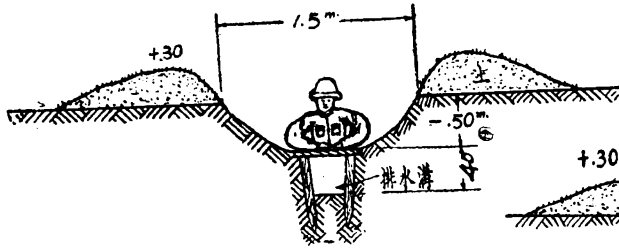
單人交通壕
