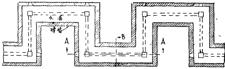
平 剖 面
