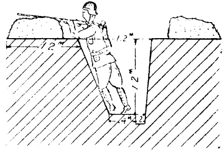
橫牆式
