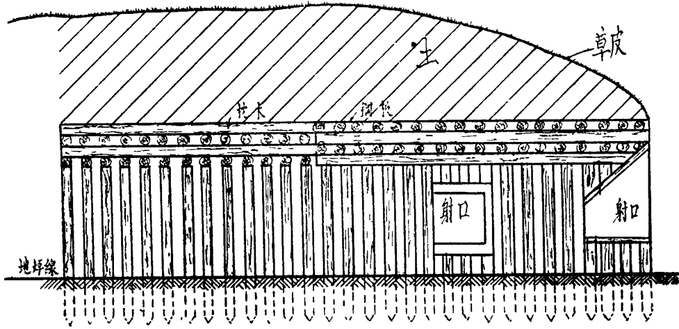
剖面 甲-甲
