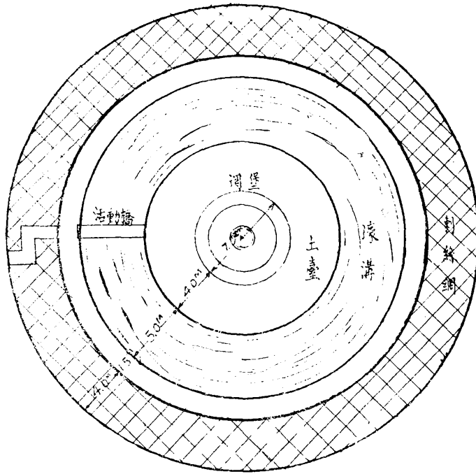
平 面
