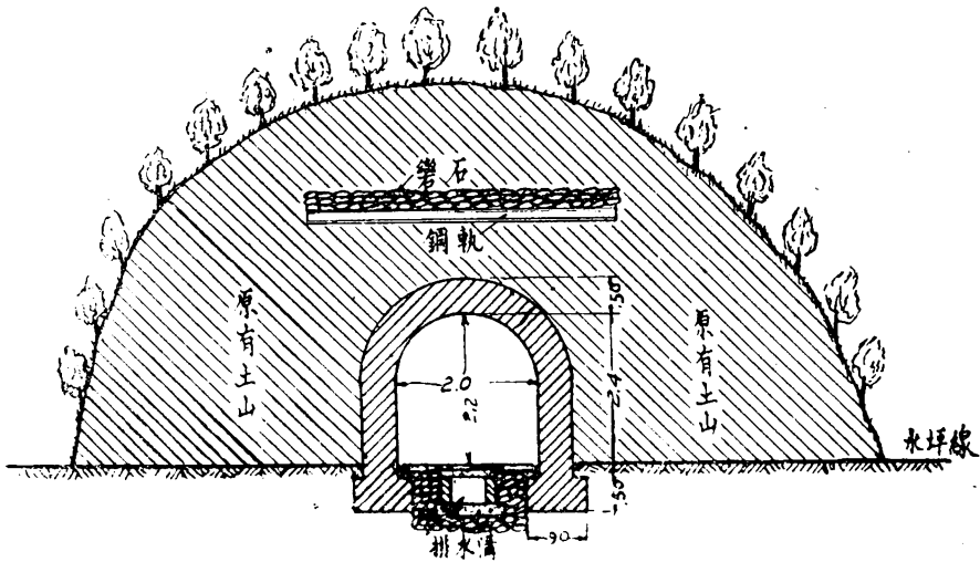
剖面 A-A
