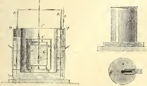
Рис. 1. Приборъ для калориметрическихъ опредѣленій по Бертелю.
