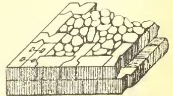
Рис. 16. Смѣшанная кладка. Соединеніе камней притескою. Соединеніе широнами.
