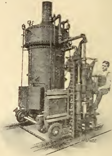
Рис. 1. Машина для производства вертикальныхъ вѣтровъ въ системѣ Нигерсоль-Сергентъ.
