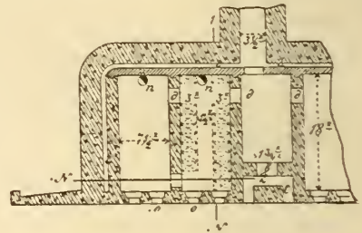
Рис. 1. Часть жилой казармы.
