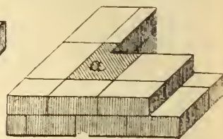
Рис. 6. Перевязка швовъ тесовой кладки.—Угольные камни.
