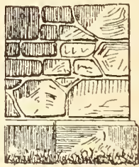
Рис. 4. Сопряженіе тесовой облицовки угловъ съ бутовой кладкою въ средневѣковыхъ зданіяхъ.
