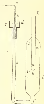
Рис. 4. Ледяной калориметръ Буинена.
