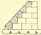
Рис. 15. Разрѣзка наклонныхъ стѣнъ изъ тесовой кладки (ледорѣзъ моста).
