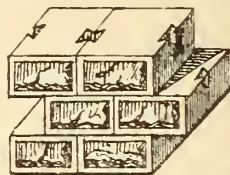
Рис. 5. Тесовая кладка. Обдѣлка лица рустами.—Соединеніе камней зачатчатыми скобами.
