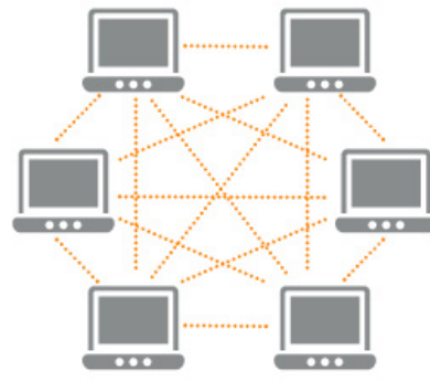
P2P
