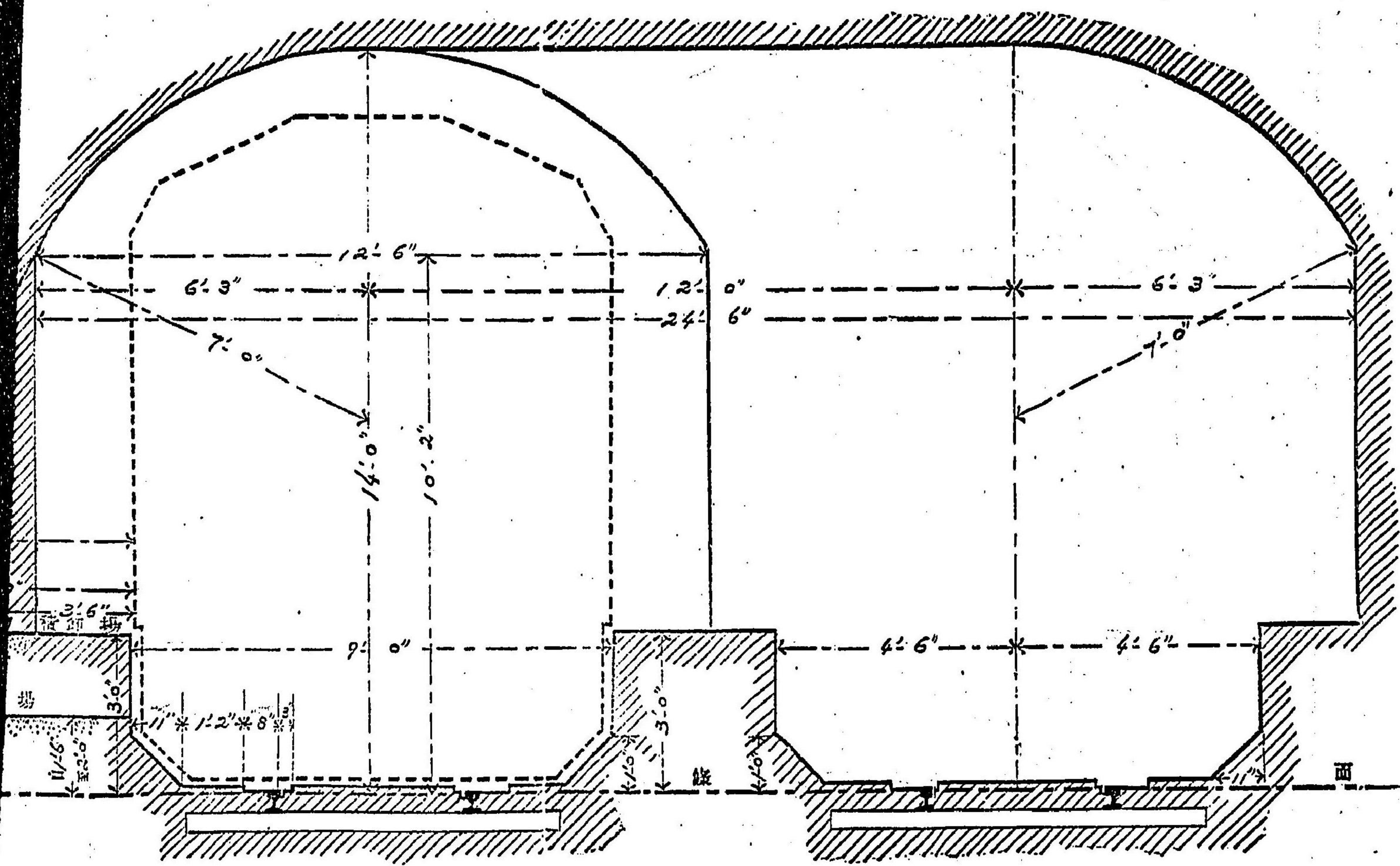
甲 號 圖 面 ( 第 一 ) 停 車 場 內 建 築 定 規
