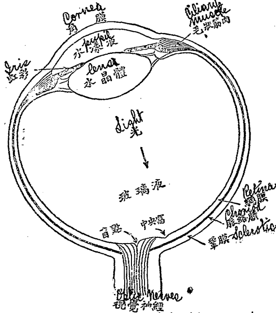
Horizontal Cross section 圖24—右眼的橫切面
