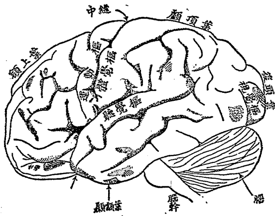
圖 11—腦的左半球，示運動樞與感覺樞(嗅覺樞見圖 41)。
