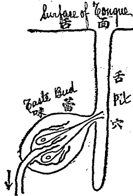
圖20—味覺細胞。味蕾內有二覺感細胞，沿此二細胞底者為味覺神經之軸索狀突起的末端。
