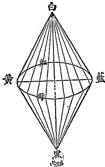
圖29—色圓錐 The Color Cone
