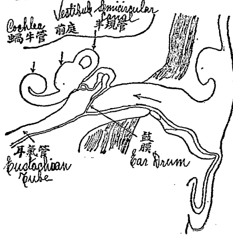
圖23—聲浪由外耳經中耳入內耳的路途，其方向以箭示之。
