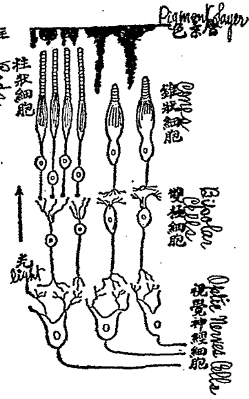
圖22—網膜的感覺細胞與神經細胞。光射過網膜，直達色素層，激動棒狀與錐狀細胞。這樣興起的神經流，過雙極細胞，達視覺神經細胞，再藉軸索狀突起傳入腦中心。
