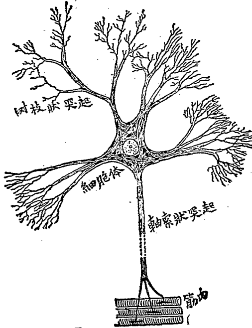
圖 4-1-1 一個放大的脊椎 髓中的運動神經細胞。
