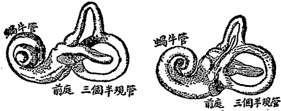
圖25—內耳的兩面觀。感覺細胞位在內耳腔內，三半規管互成垂面。
