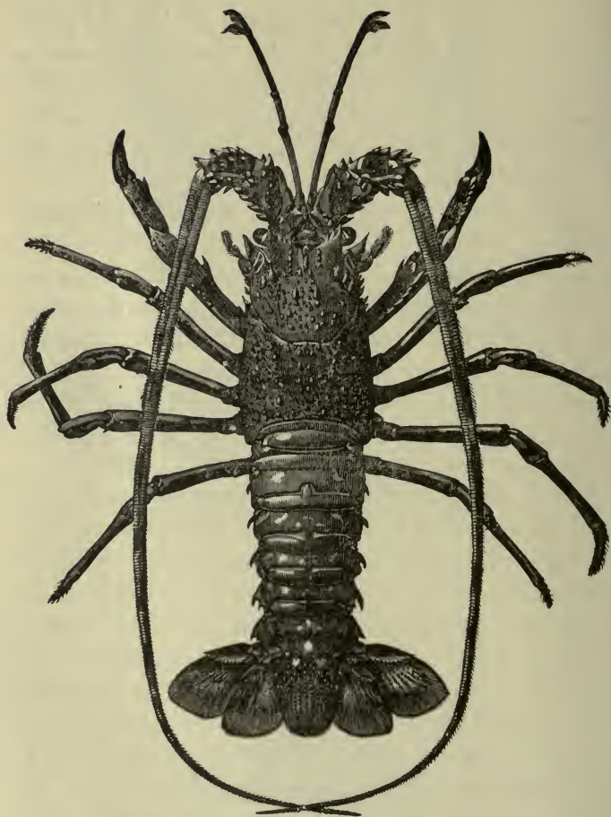
FIG. 70. Palinurus vulgaris (about \frac{1}{4} nat. size).
