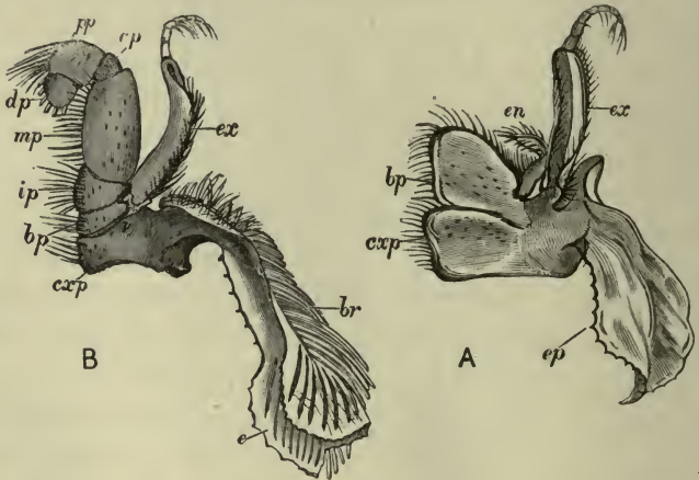
FIG. 45.— Astacus fluviatilis .—A, the first; B, the second maxillipede of the left side ( \times 3 ). exp , coxopodite; bp , basipodite; e , br , podobranchia; ep , epipodite; en , endopodite; ex , exopodite; ip , ischiopodite; mp , meropodite; cp , carpopodite; pp , propodite; dp , dactylopodite.
