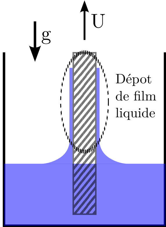
Situation dynamique
