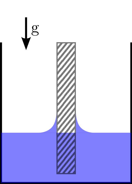
Situation statique
