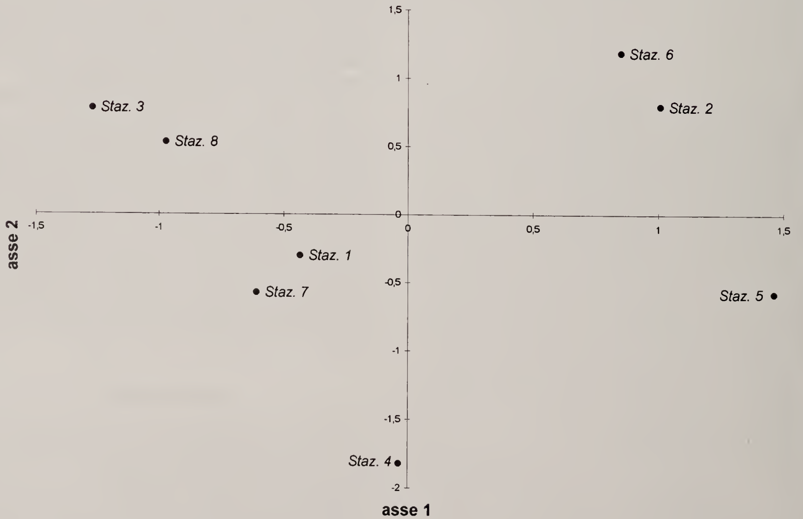
Fig. 6.2 - Confronto delle stazioni 1-8 mediante analisi delle componenti principali.
