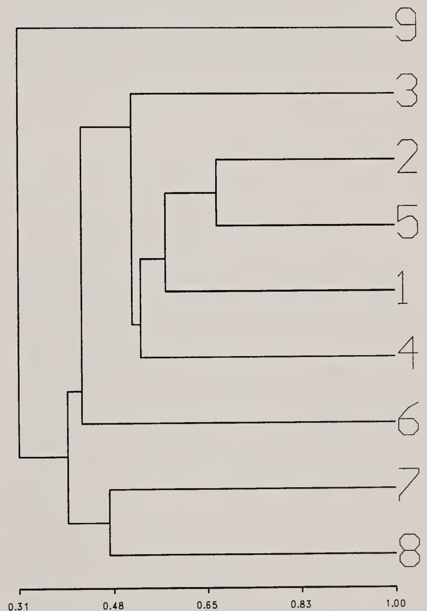
Fig. 8 - Dendrogramma di similarità fra le stazioni 1-9 basato sui campionamenti di Curculionidi (indice di Dice/Sorensen + WPGMA).
