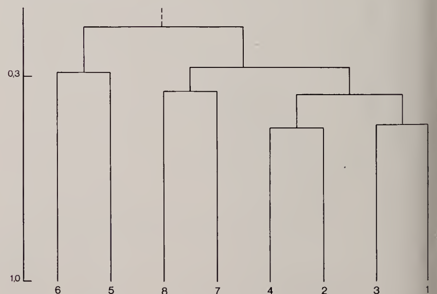
Fig. 5 - Dendrogramma delle stazioni 1-8 (WPGMA su Percent Similarity).
