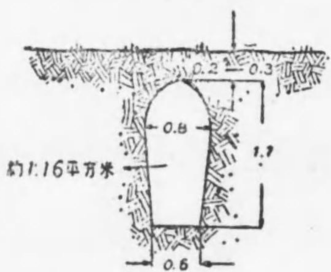
壕通交ノ面斷窪穹
