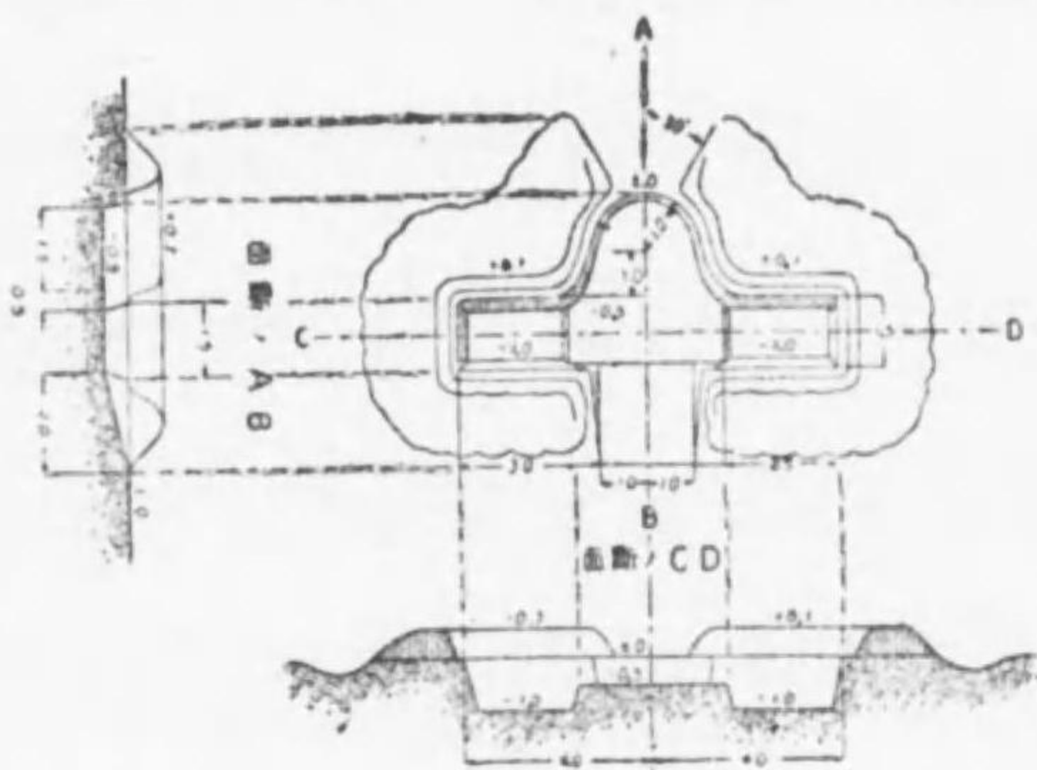
山砲ノ掩體
