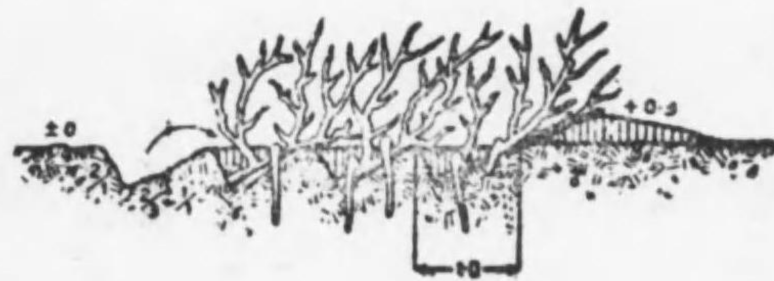
樹枝鹿砦
