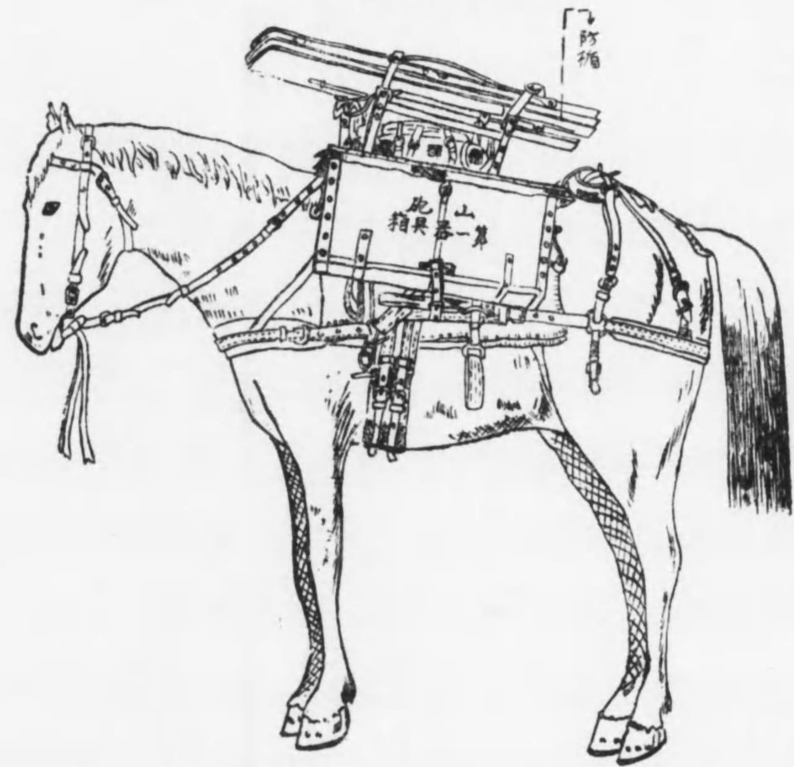
圖六第 載馱ノ箱具器防 (只ノ箱兵器一ノ例也)
