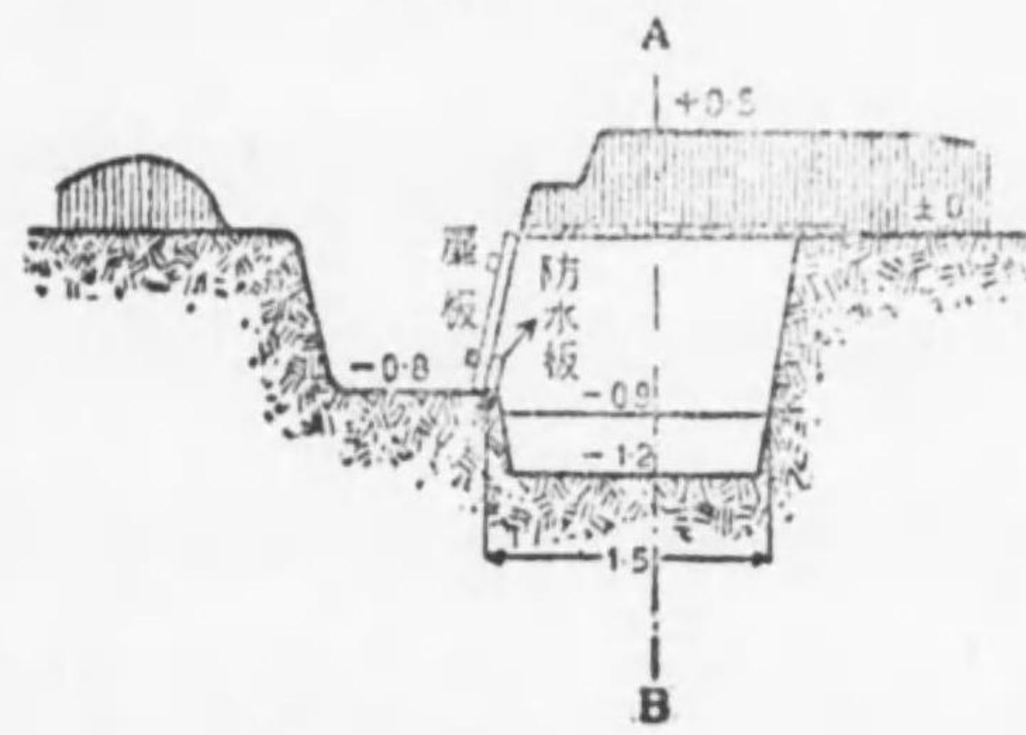
面斷ノC D
