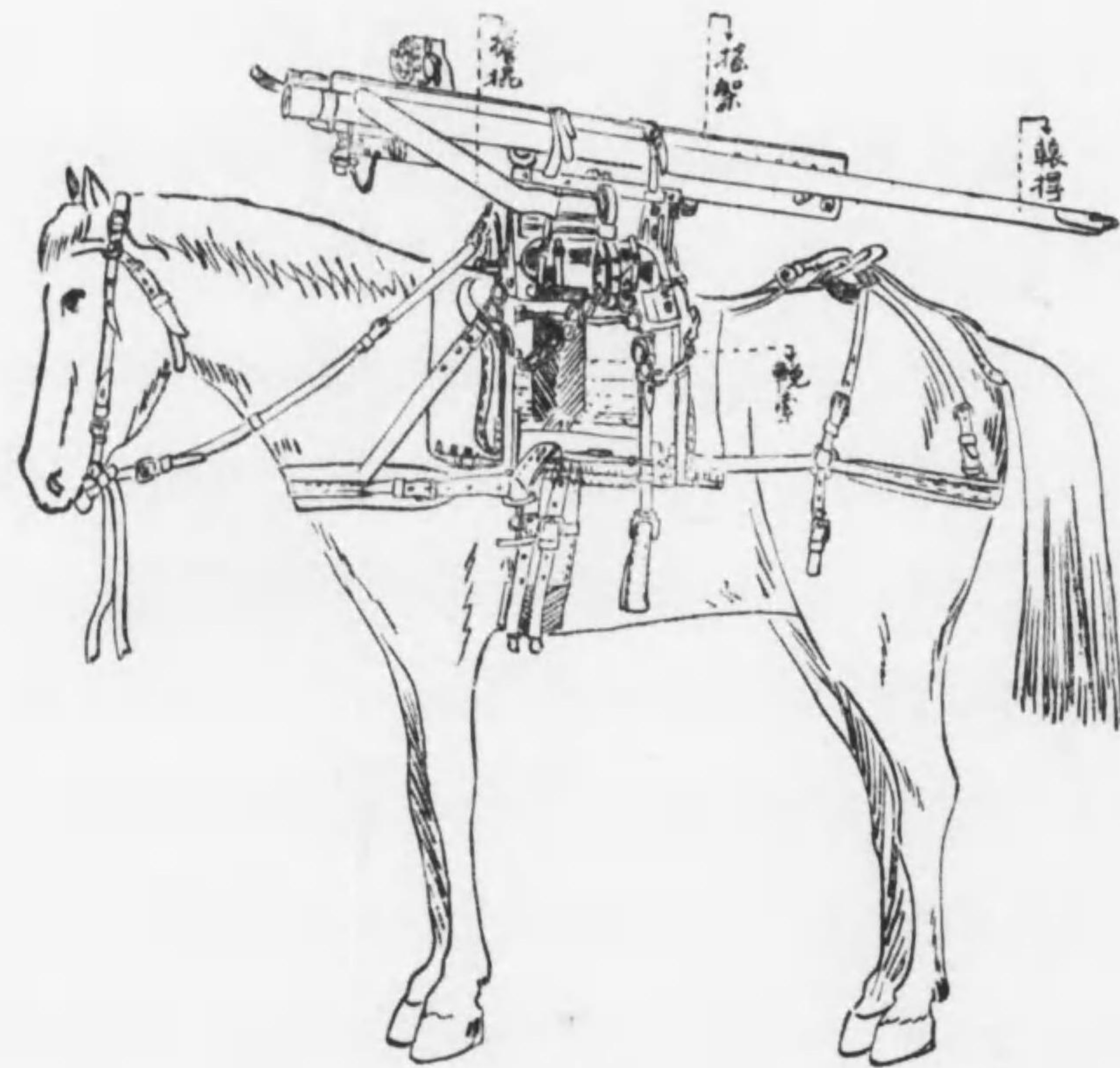
圖三第 載馱、架控
