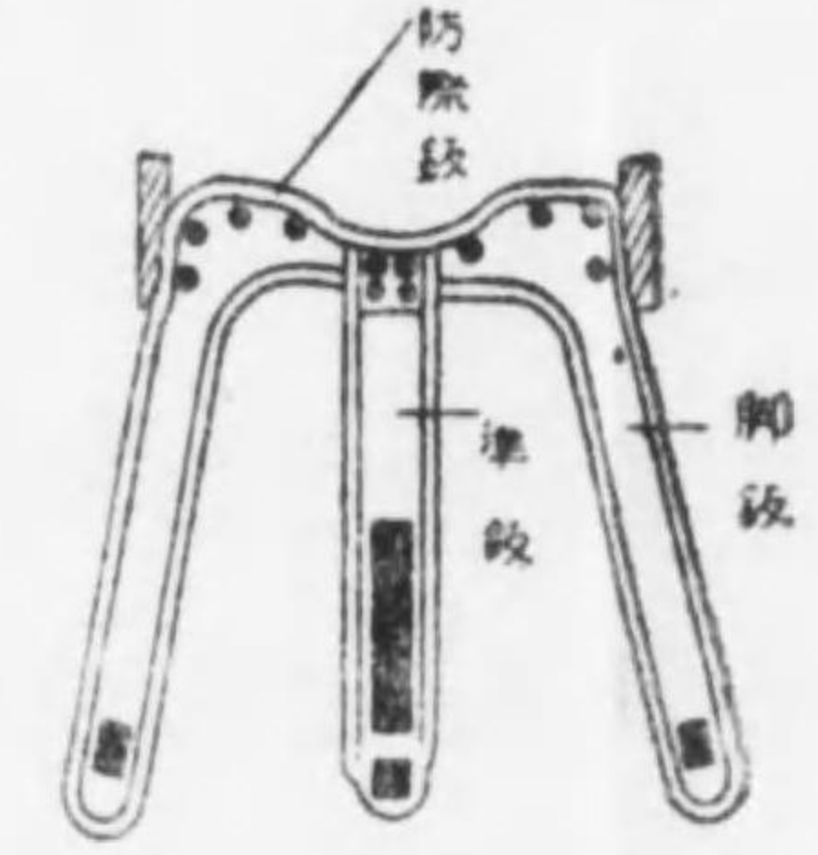
匡架身砲 面側
