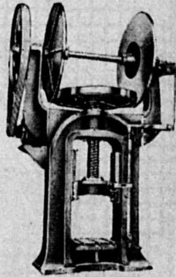
フリクションプレス
