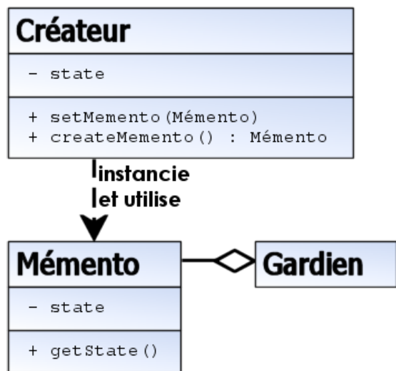
Diagramme de classes UML du patron de conception Mémento
