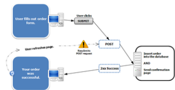
Diagramme d'un problème de multiple soumission.
