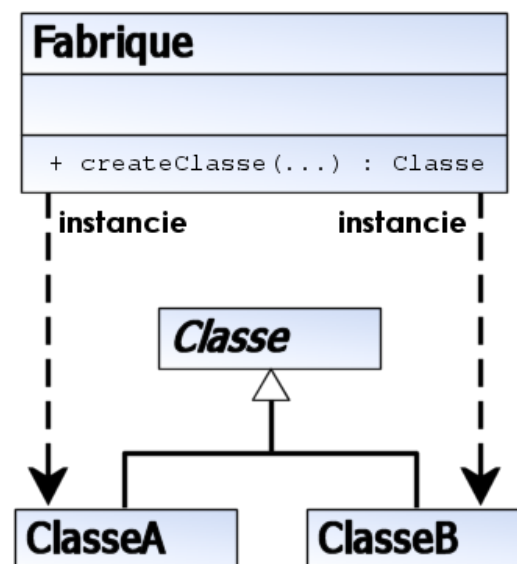
Diagramme de classe pour le patron de conception Fabrique
