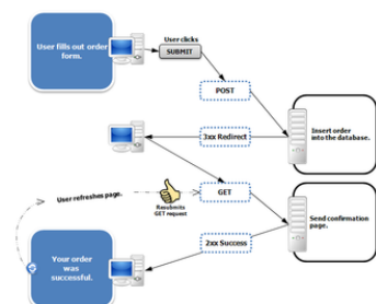
Diagramme de la résolution du problème avec le patron PRG.
