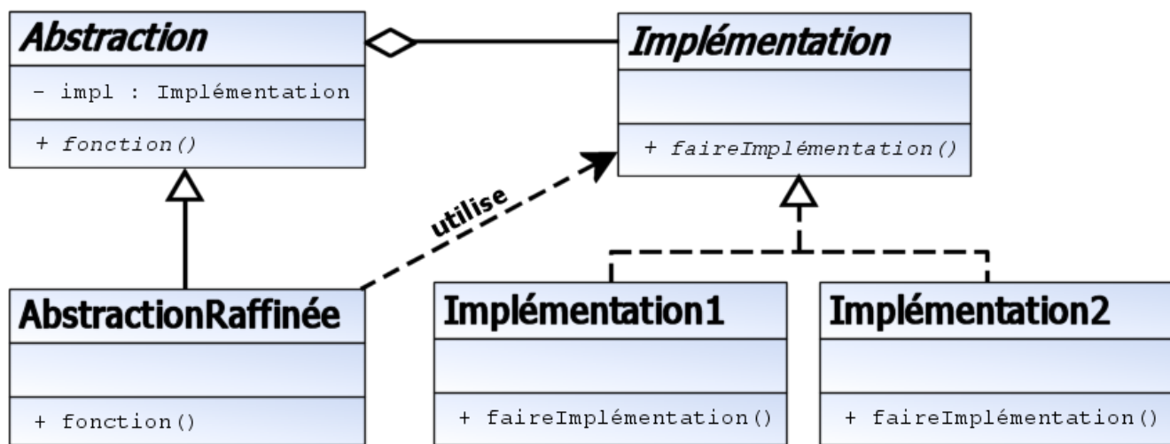
Diagramme UML de classes du patron de conception Pont
