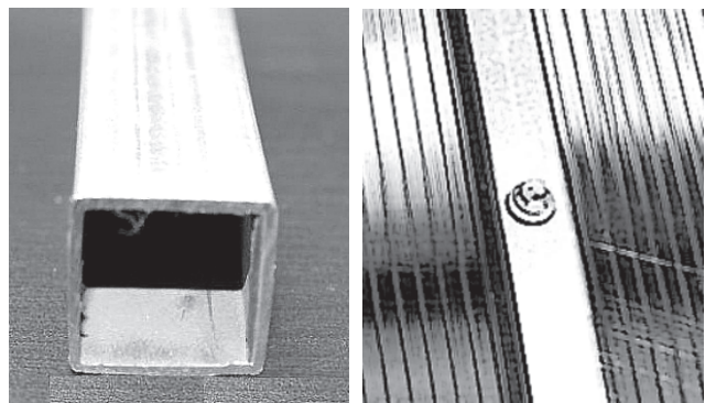
Вид оцинкованной квадратной профильной трубы Усиленное крепление: саморез + оцинкованная лента
