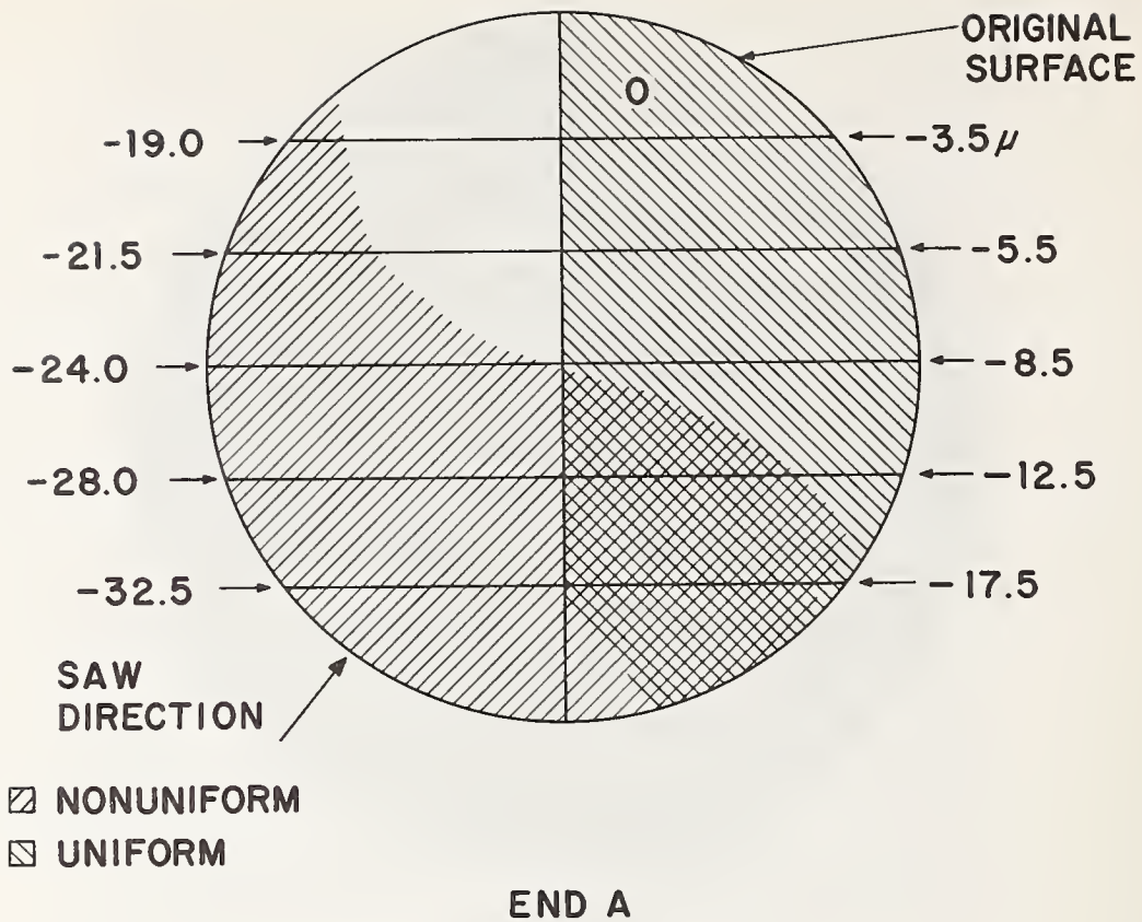
Fig. C.8. Damage map, end A.
