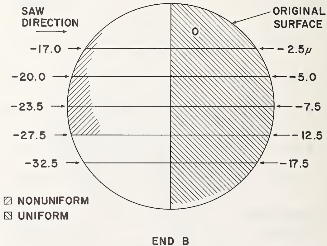
Fig. C.9. Damage map, end B.
