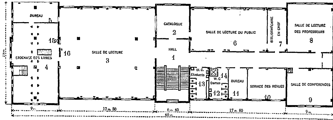
震旦大學新圖書館主要部份平面圖
