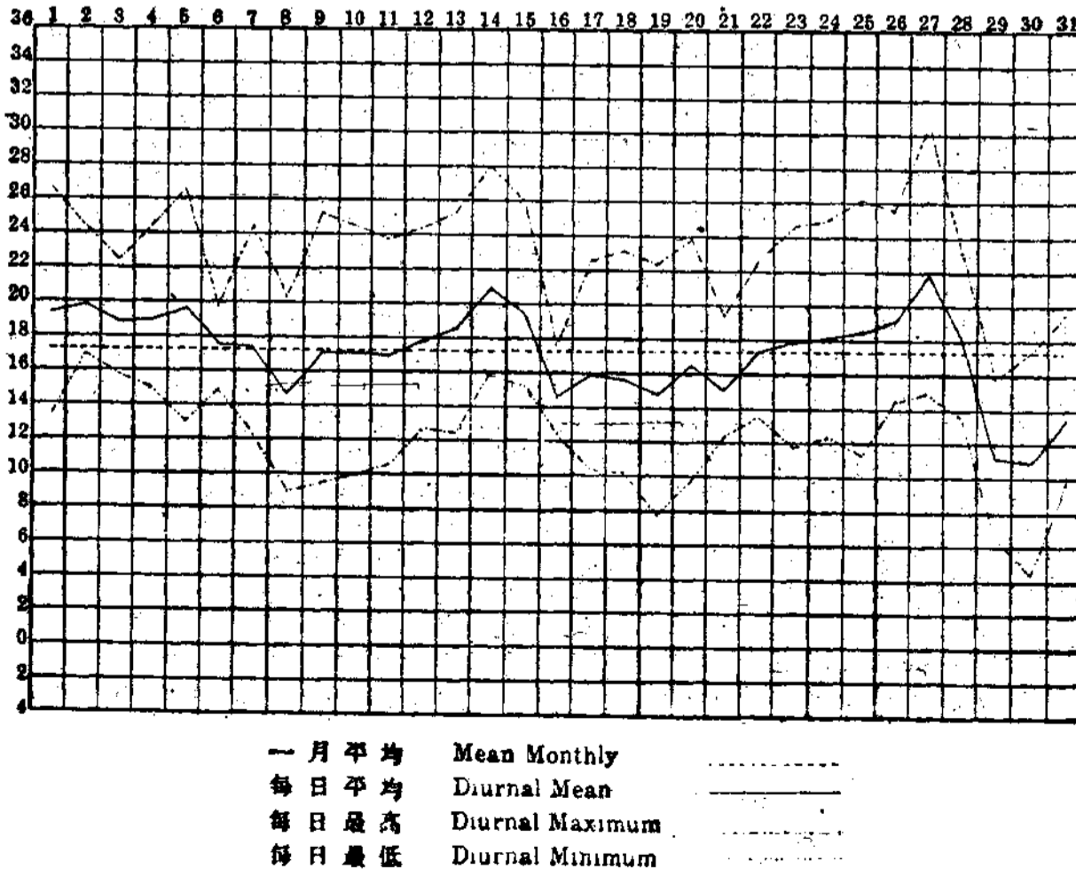
中華民國十七年十月份氣溫變遷圖 (°C) The March of Temperature in the Month of October, 1928. (°C)
