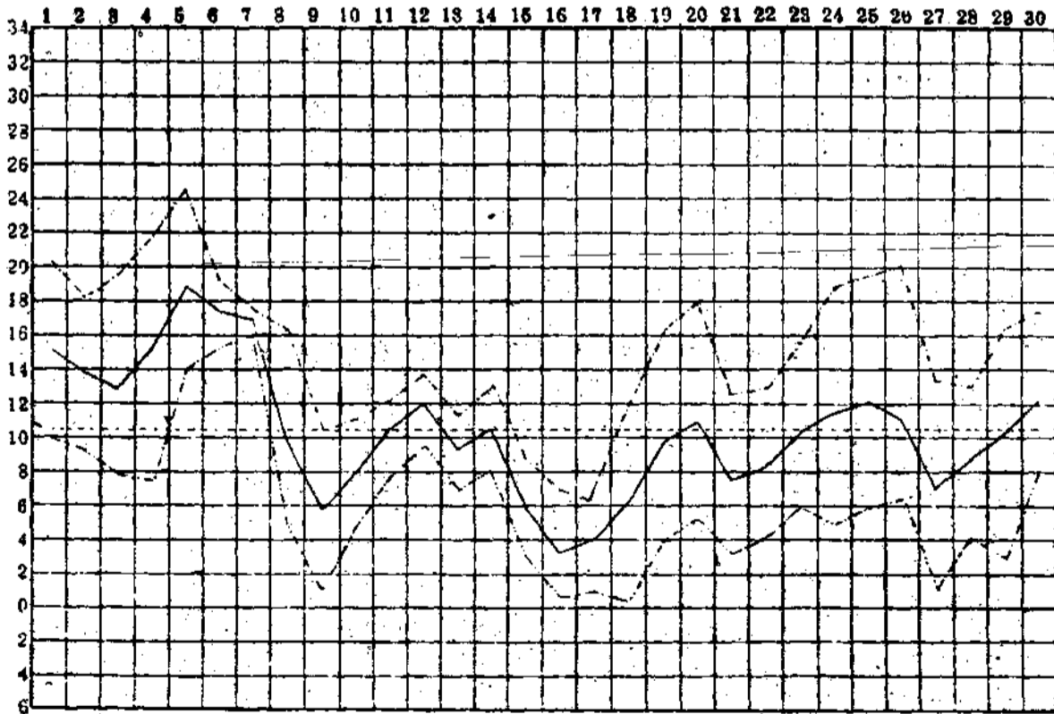
中華民國十七年十一月份氣溫變遷圖 (°C) The March of Temperature in the Month of November, 1928 (°C)
