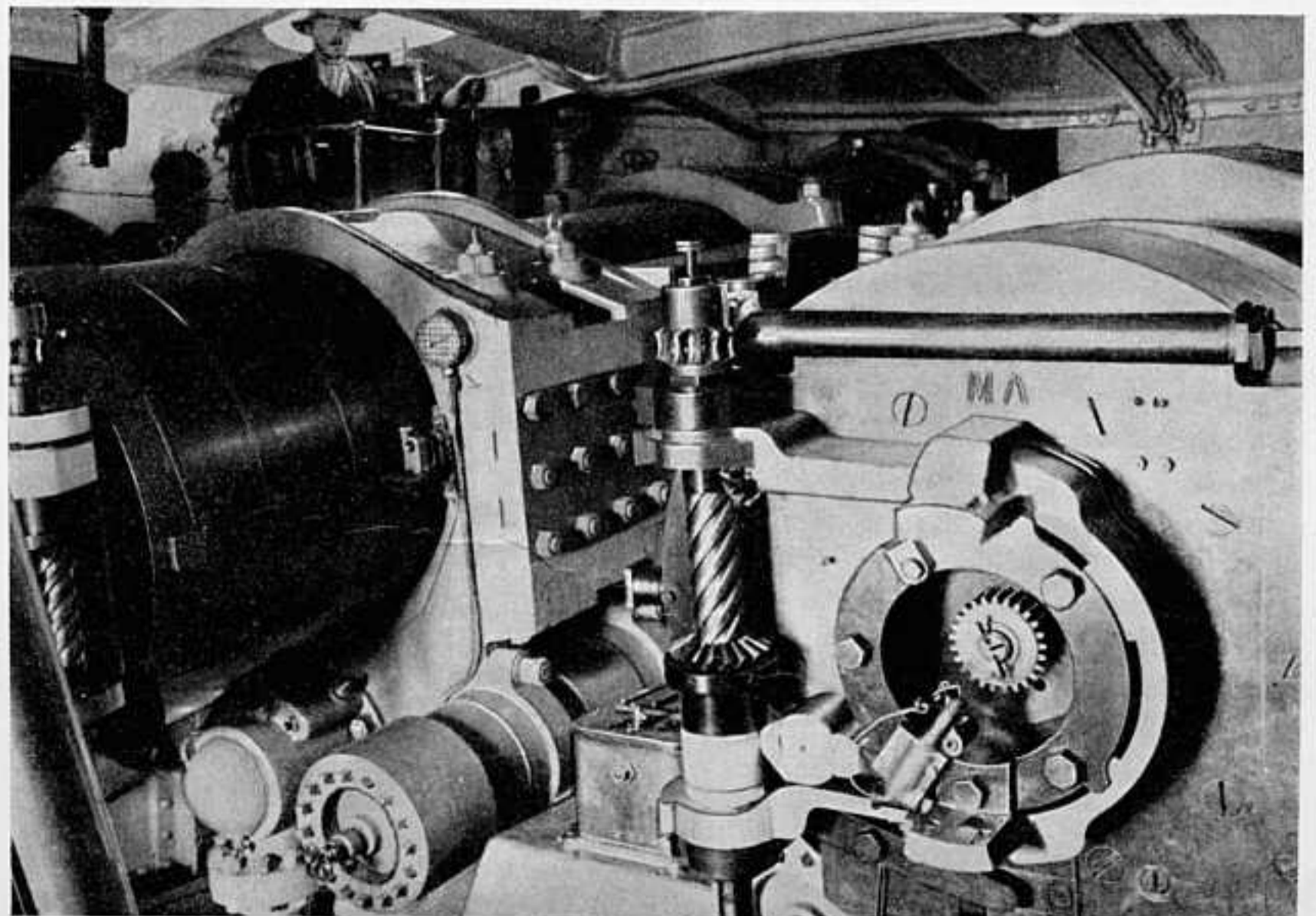
КАЗЕННАЯ ЧАСТЬ 12-ТИ-ДЮЙМОВЫХЪ ОРУДІЙ.
