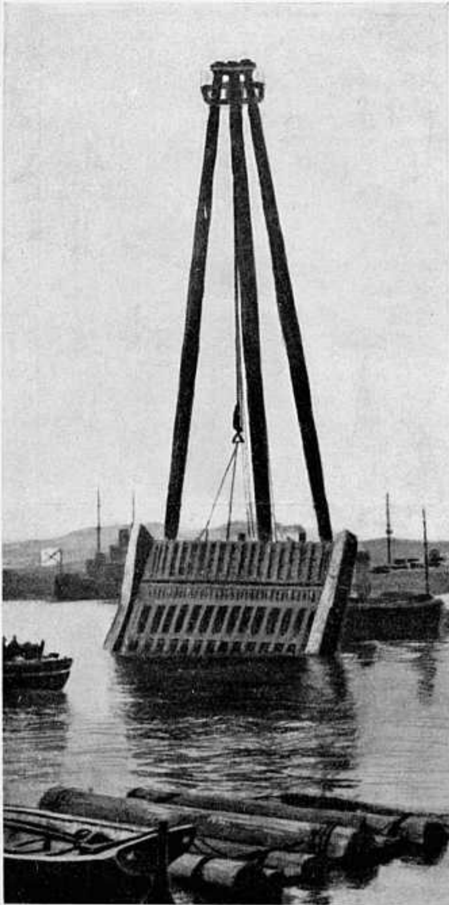
ПОНТОНЪ, ПРИ ПОСРЕДСТВѢ КОТОРАГО ЗАДѢЛЫВАЛИСЬ ПРОБОИНЫ НА ПОВРЕЖДЕННЫХЪ СУДАХЪ.
