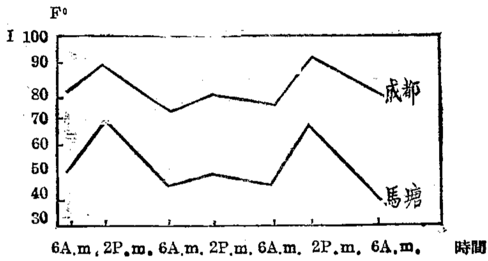
圖四： 成都與威塘日溫變化圖
