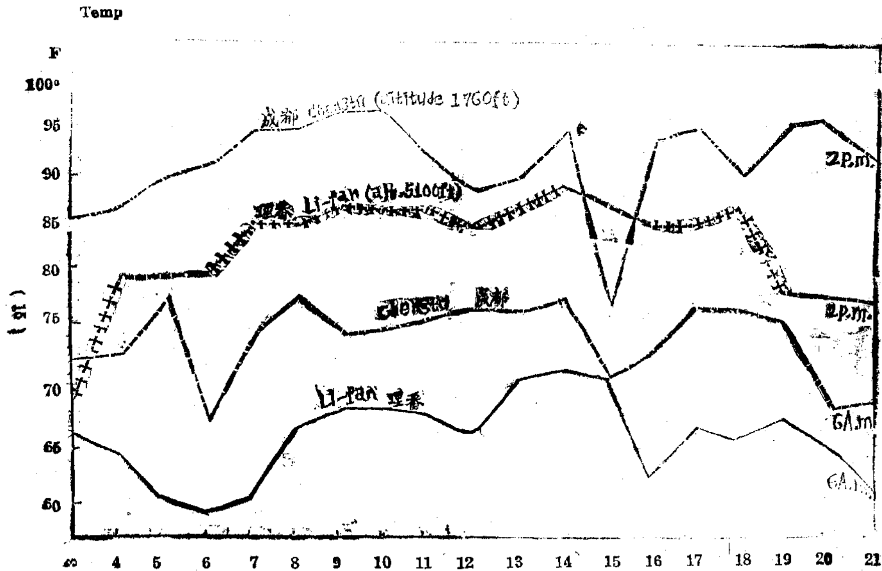
圖三： 成都與理番最高最低溫度比較(一九四一年八月三日至二十一日)
