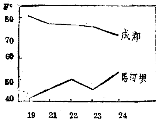
圖五： 成都與馬河壩溫度之比較
