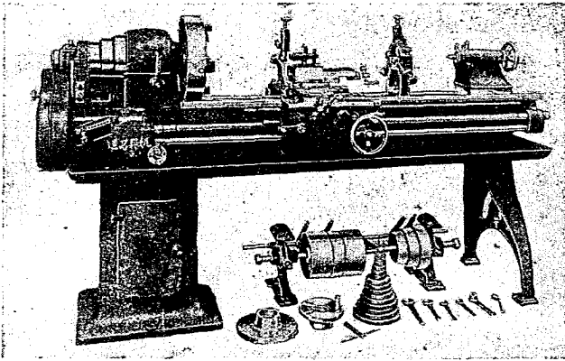
新式車床 (計分六尺八寸，二十三尺種)
