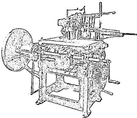
新式模範自動鑄字機 Automatic Type Caster Machine
