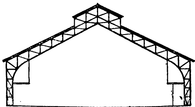
第十七圖 廣大之鋼架
