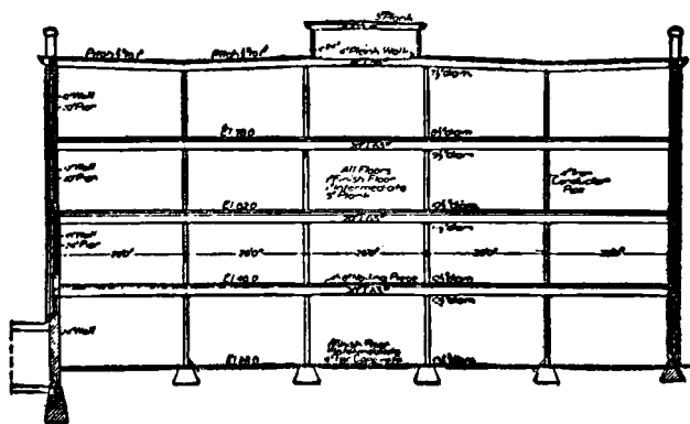
第十五圖 較大之鋼架廠屋結構
