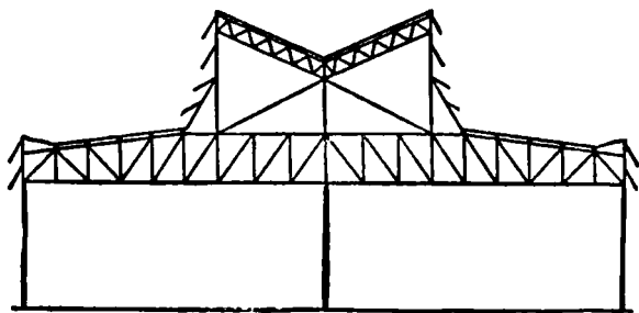
第八圖 斜坡向上之直脊式通風窗
