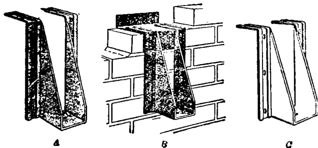
第十一圖 橫梁承攔於牆上之法
