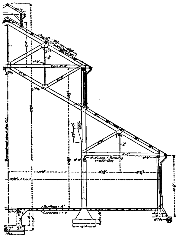
第十圖 柱與橫梁之結構
