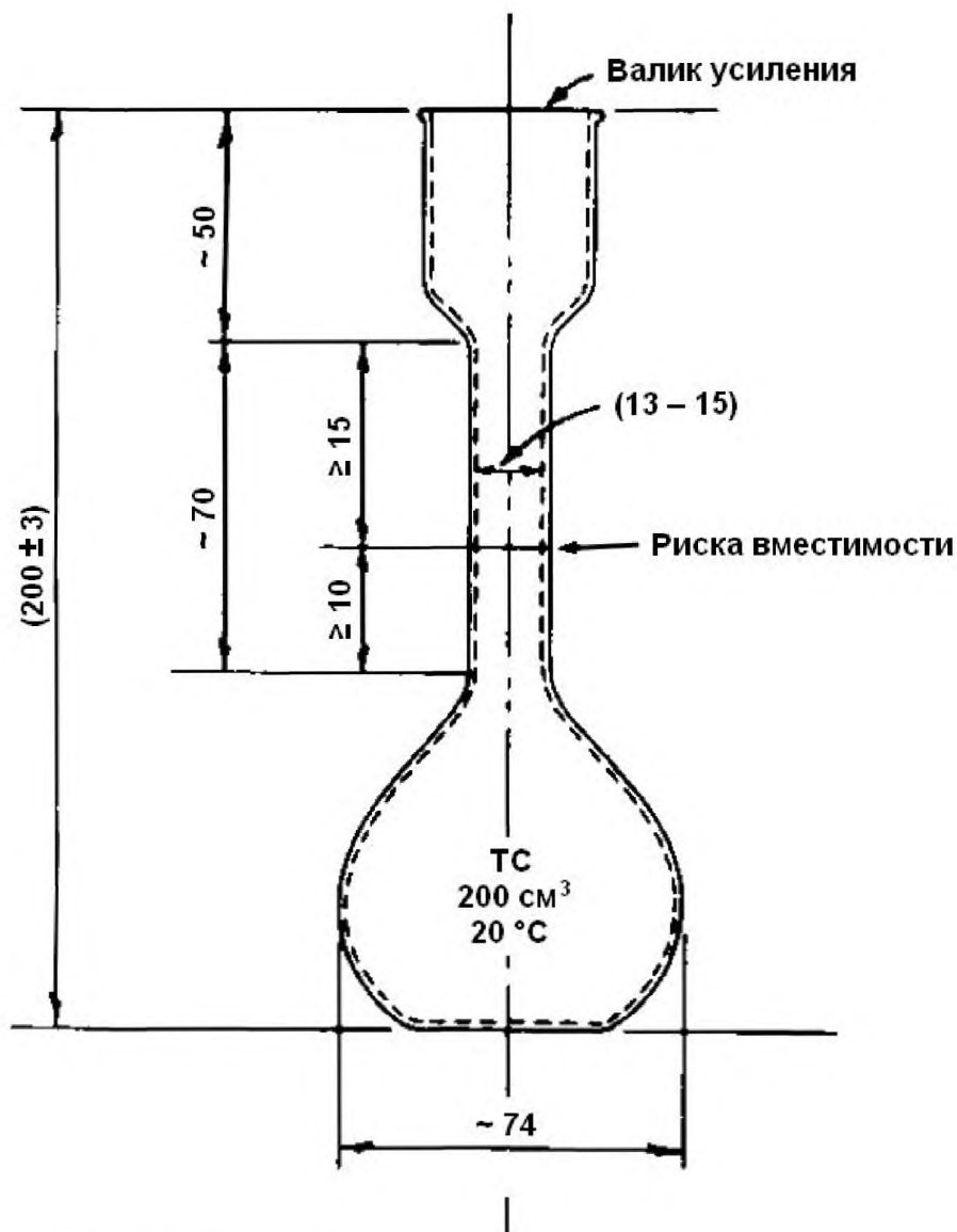
Рисунок 3 – Колба Кольрауша
