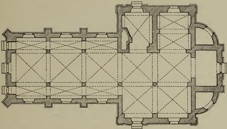
Grundriss der Kirche zu Meuselwitz.
