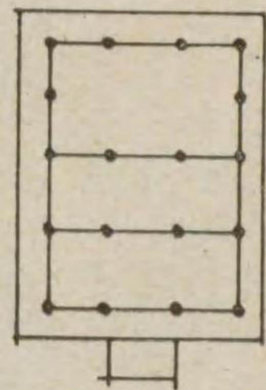
八幡造平面
