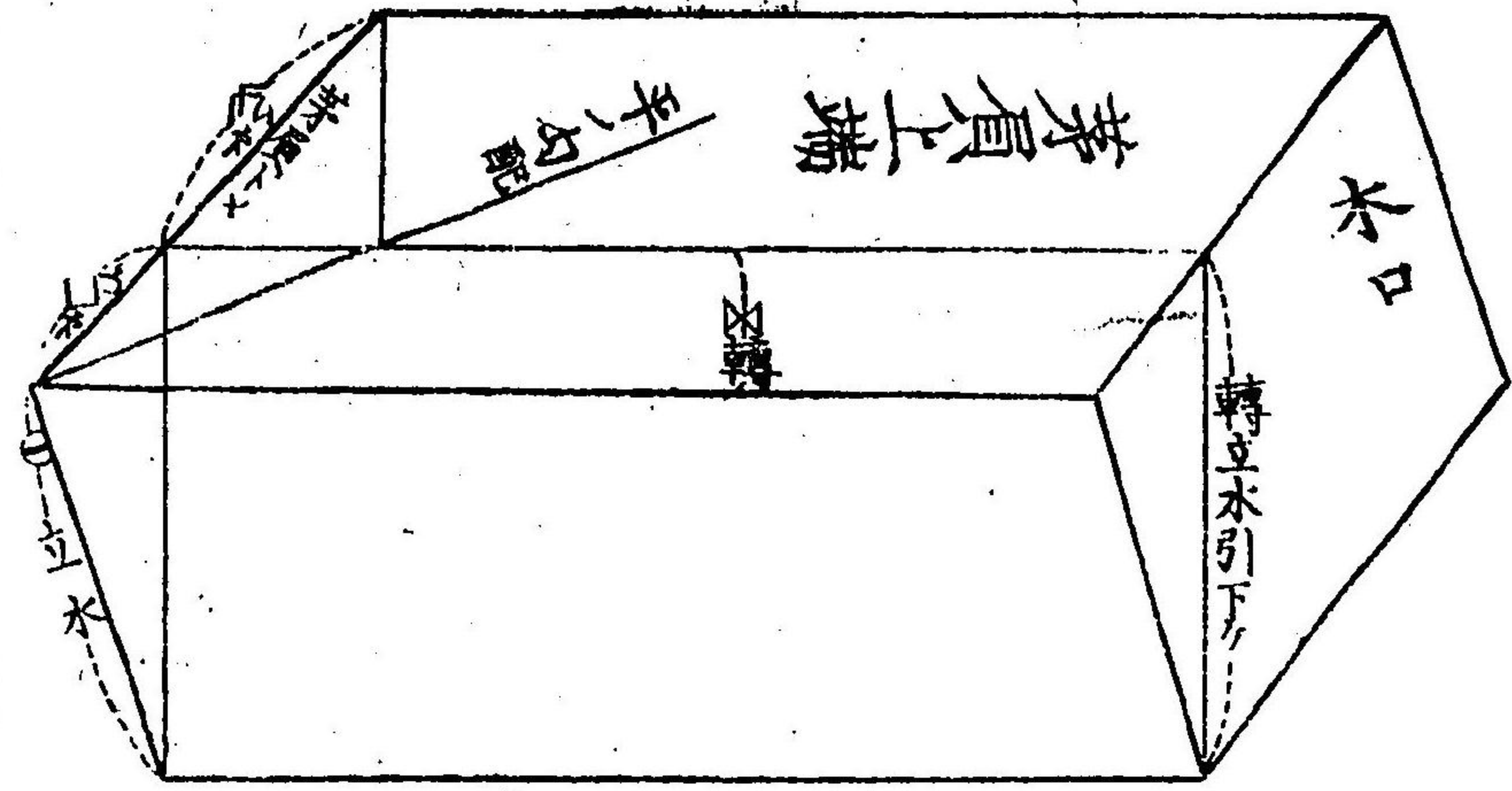
木負素肩隅木脇面打墨圖
