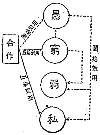
合作效用圖
