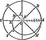
阿基米得螺線圖
