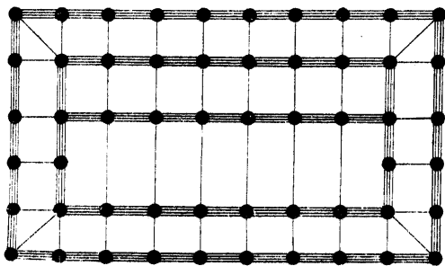
殿閣地盤殿身七間副階 周市各兩椽身內單槽
