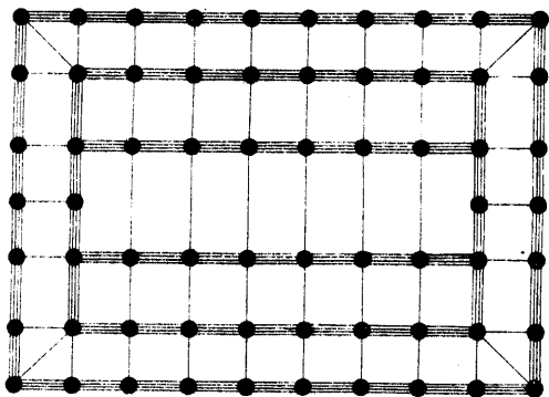
殿閣地盤殿身七間副階 周市各兩椽身內雙槽
