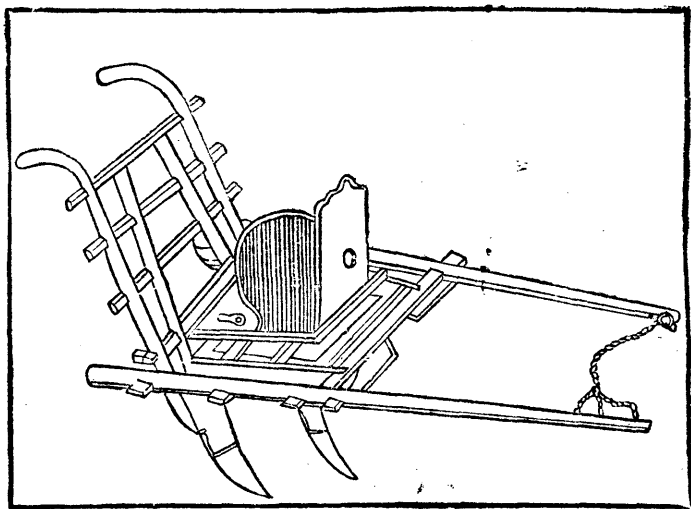
(書全政農) 車 種
