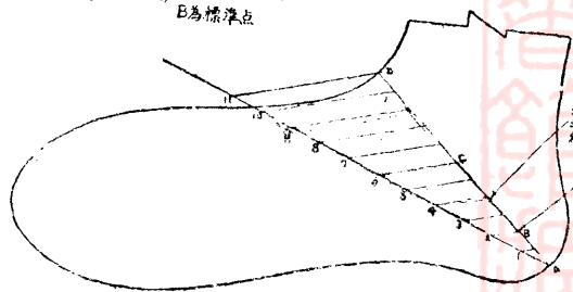
第十一圖 標準點之求法 說明：所給點均用圓點中 心A為跟線與圓底中心之距 AD為A至D之距離，D為跟線 上之點，BC為跟線之 切線，B為標準點
