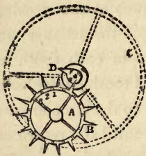
Duplex Escapement.
