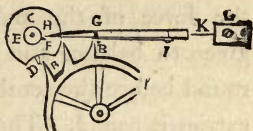
Chronometer Escapement.
