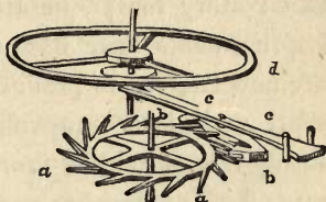
Lever Escapement.
