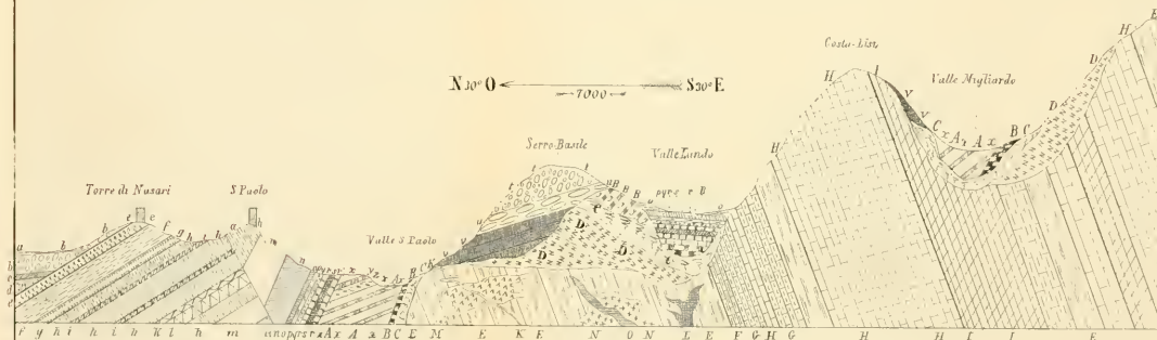
T. II. Riunione teorica di tali naturali secondo una linea che unisce Costa del Sardo a Collaina
