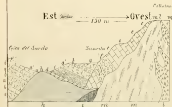
T. II. Riunione teorica di tali naturali secondo una linea che unisce Costa del Sardo a Collaina
