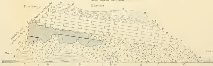
T. III. Sezione teorica trasversalmente al Capo di Milazzo Ovest ← 500 m circa → Est
