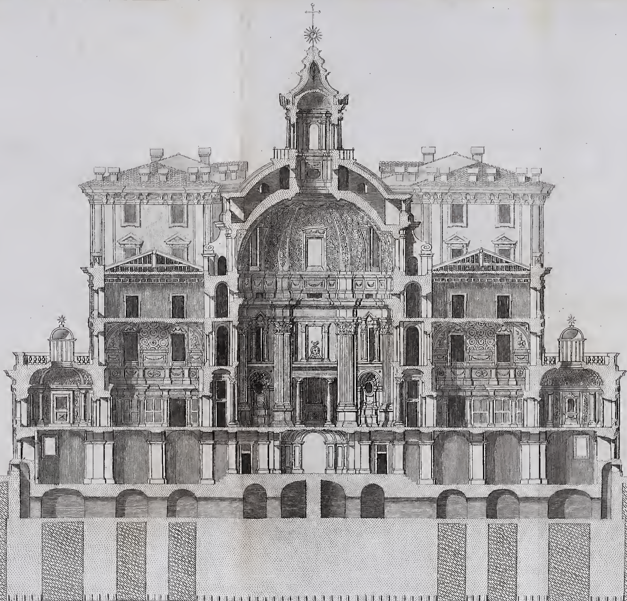
Scenographia diagonalis Cellae, et Sacrarii Canoniorum, Sacrarii Majoris, Cellae, et Sacrarii Beneficiorum versus Aquilonem. Cryptoporticus. Hypogea Conditoria. Fundamenta. in Tab. Ichn. VII. Lit. T. V. V. p. 1844. Carloni inc.
