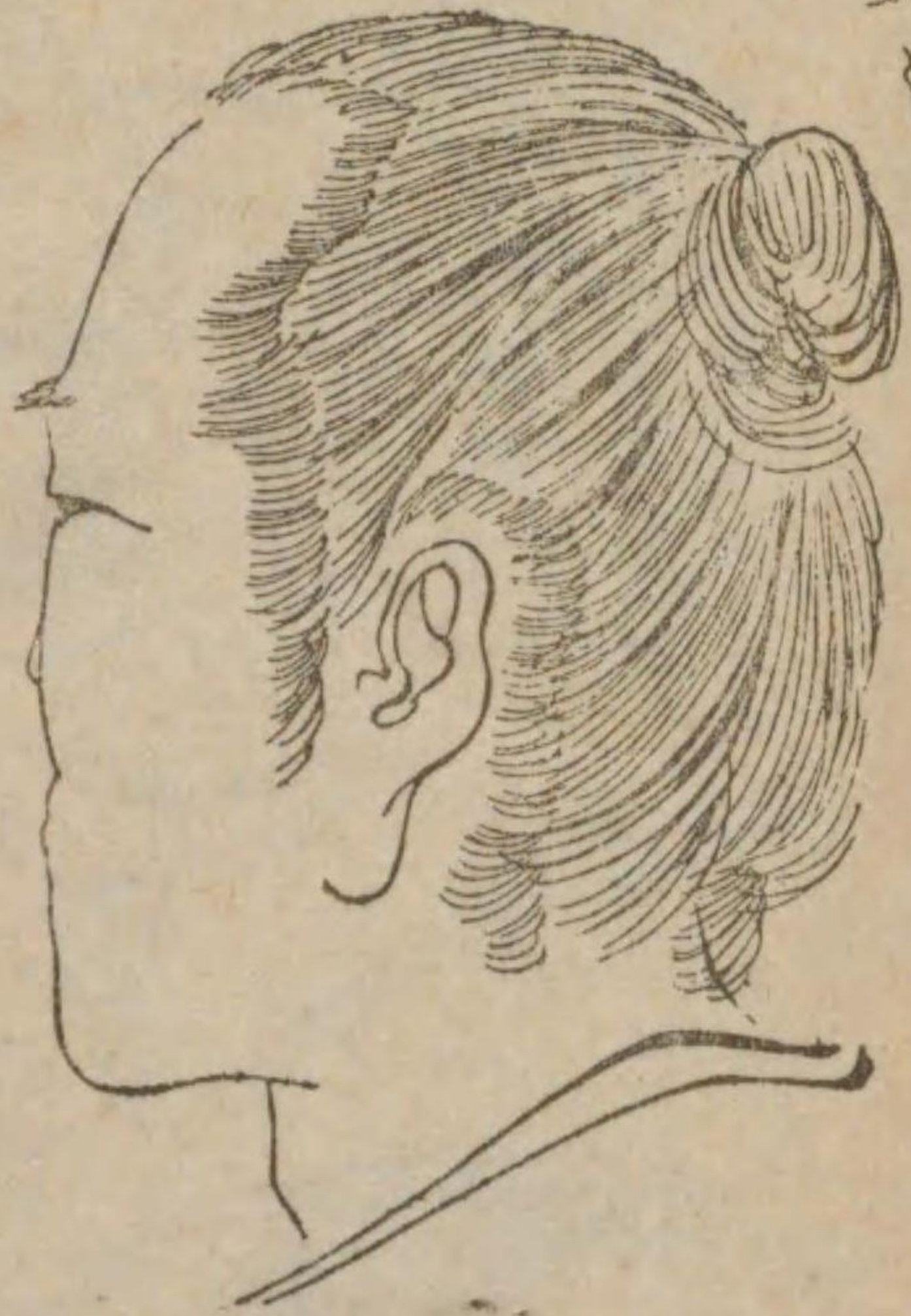
四分法
