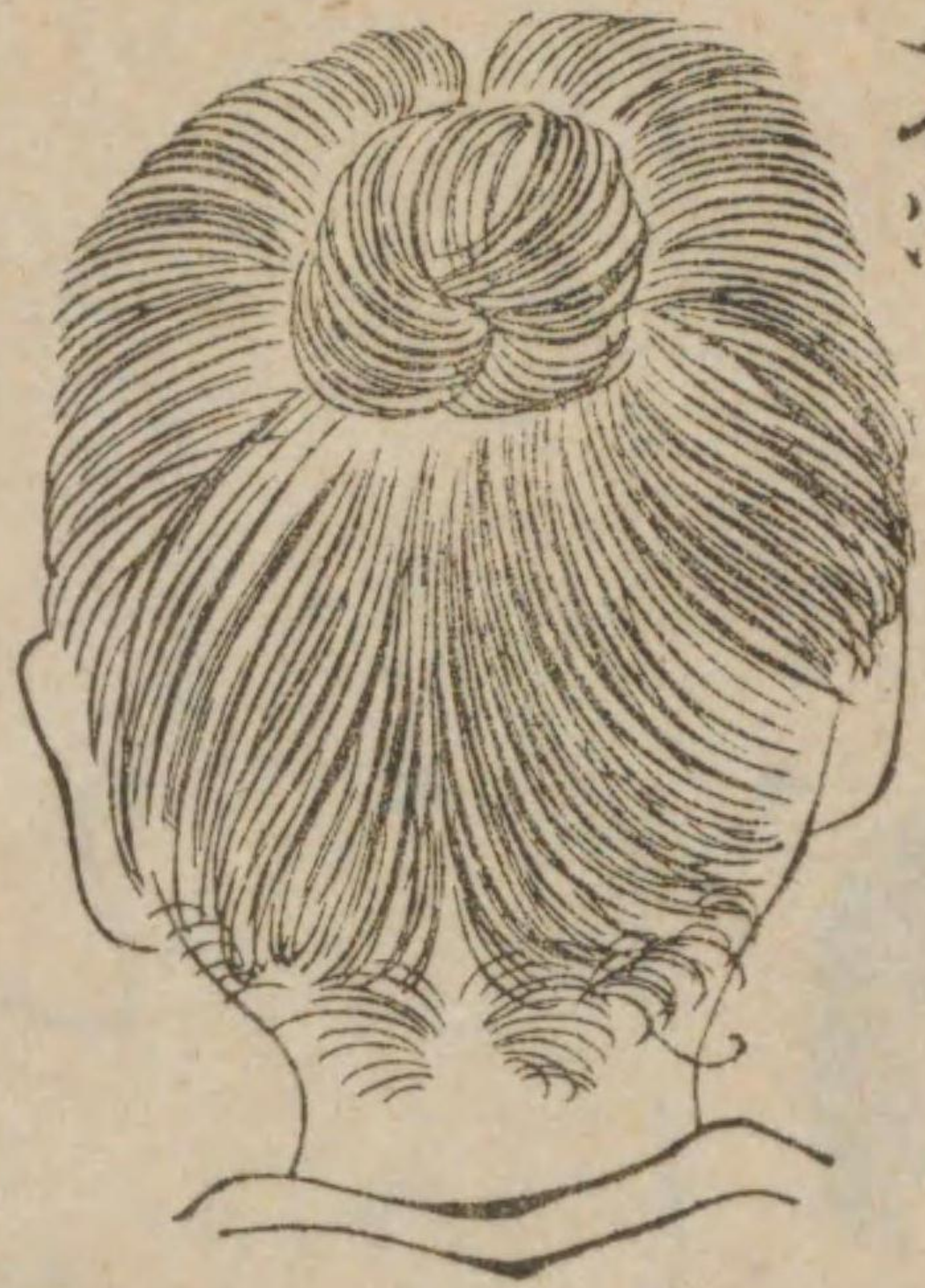
二分法
