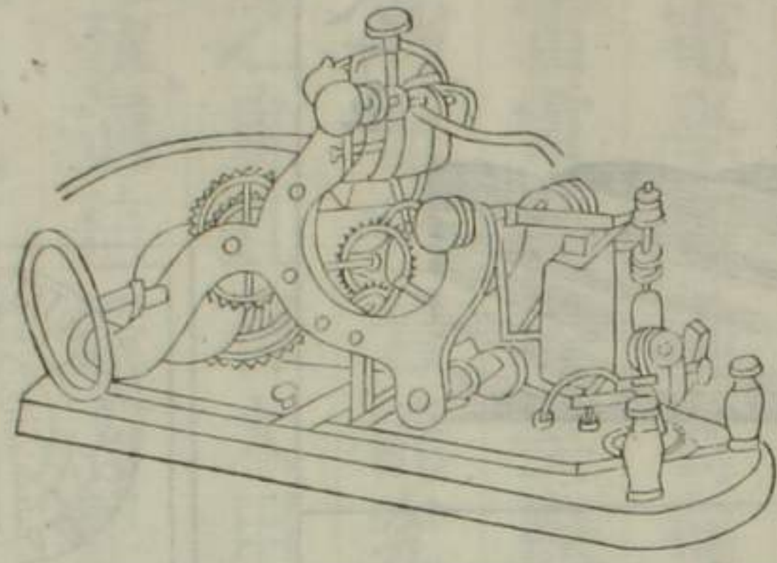
畫字機
