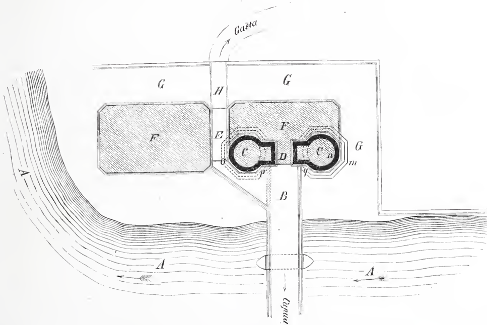
Fig. 1. Grundrissfizzi des Brückenkopfes am Volturmo bei Capua.
