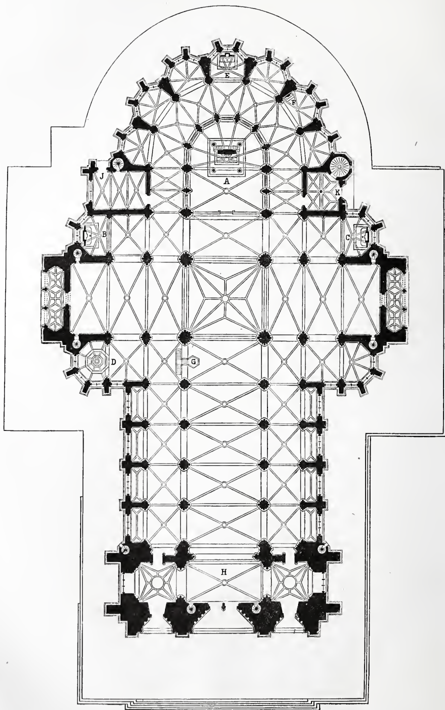
Grundriß der Botivkirche.
