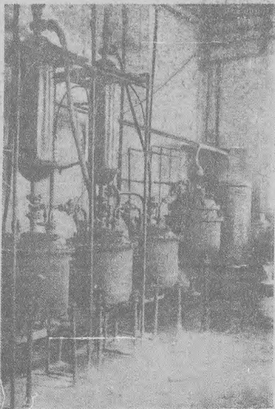
現代製香料之機器
