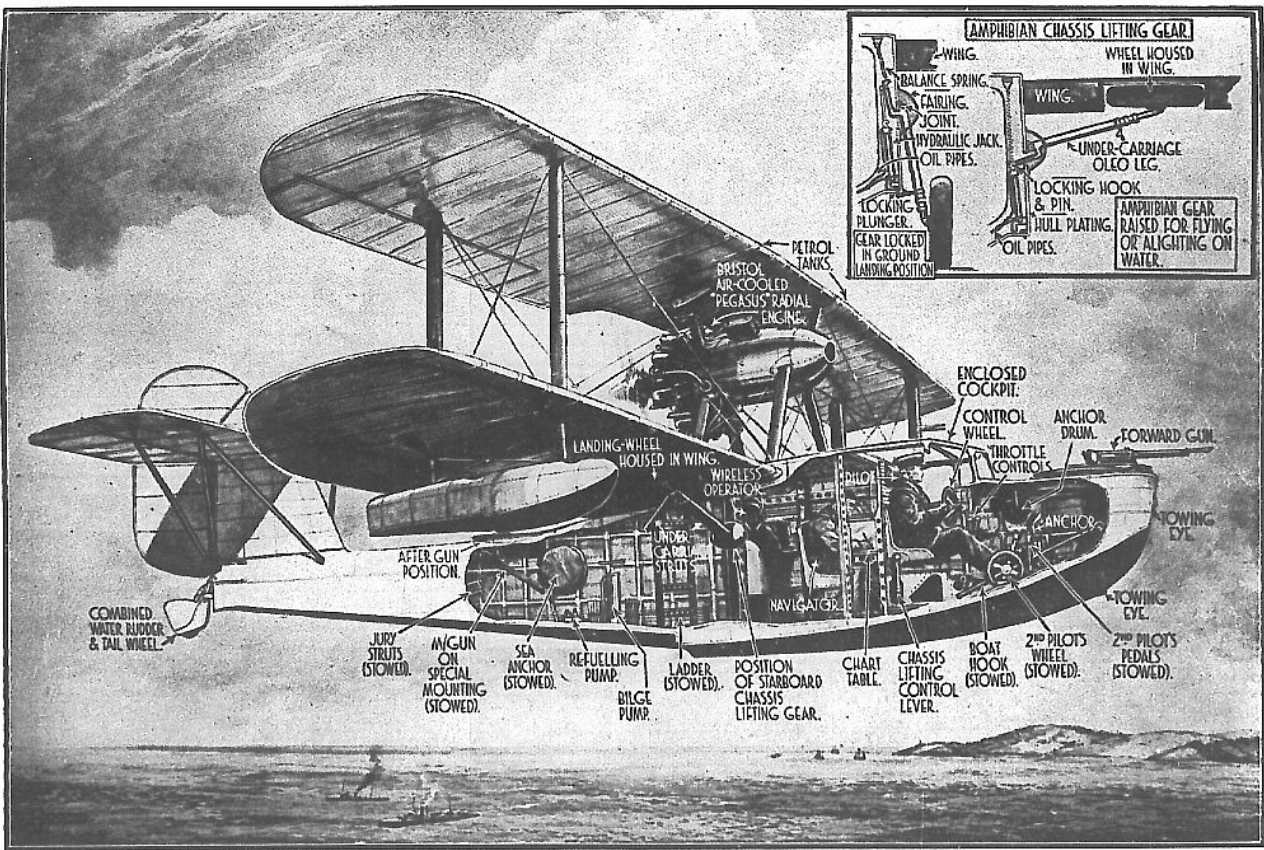
英國水上飛機 "Seagull" Mk V 內部構造
