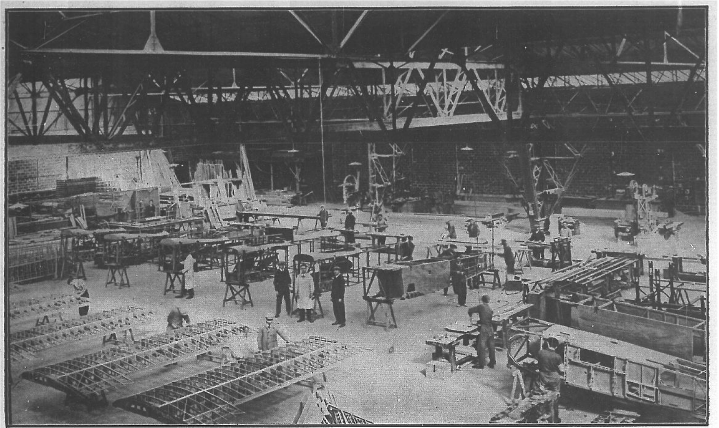
法國亨利歐(Hanriot)工廠製造機翼及機身部
