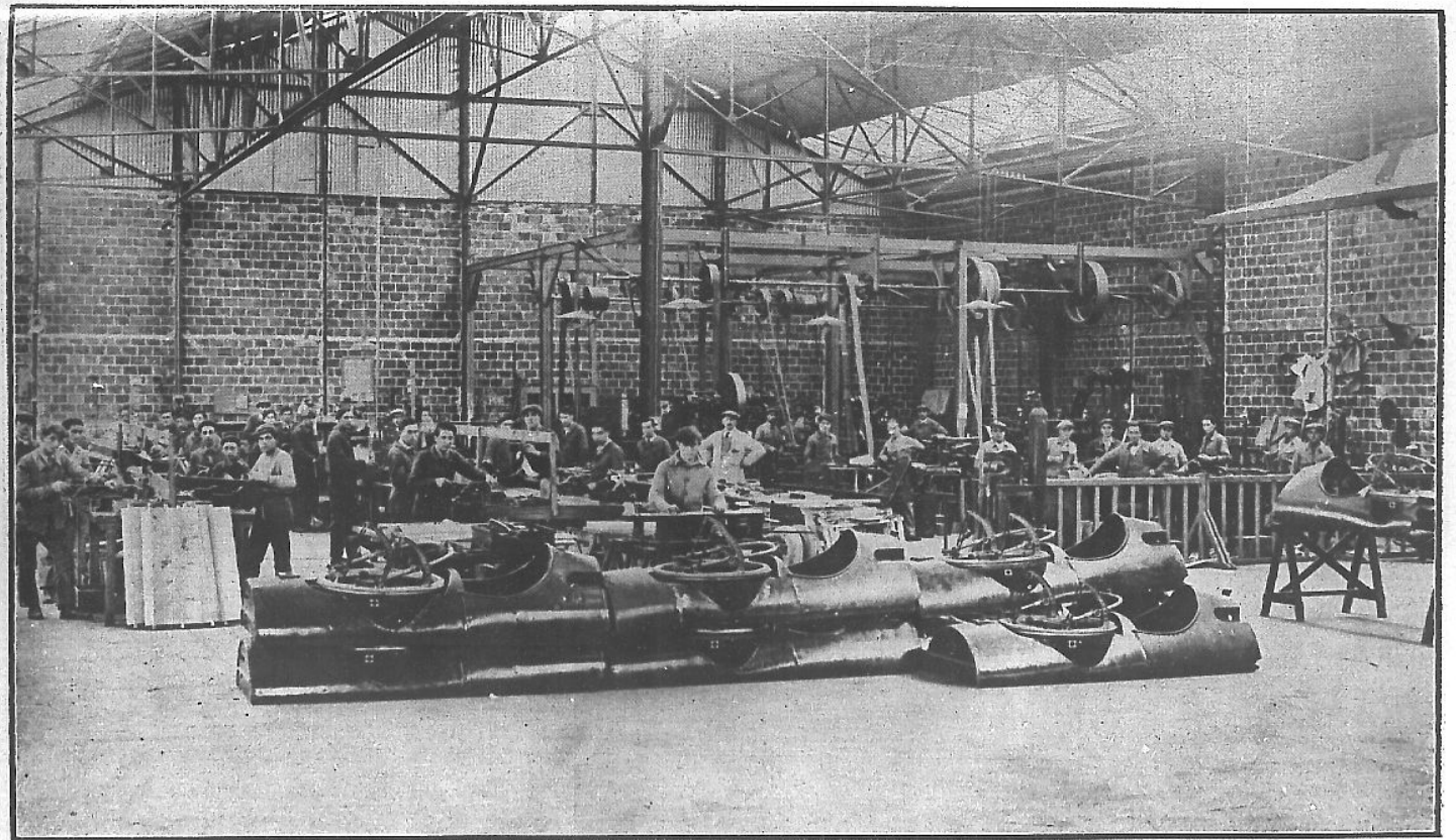
法 國 亨 利 歐 (Hanriot) 廠 製 造 機 身 上 機 關 槍 架 之 一 部
