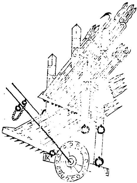
飛轅寨式
