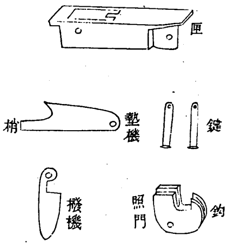
圖散機弩銅制新古改
