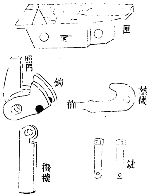
古銅弩機散圖
