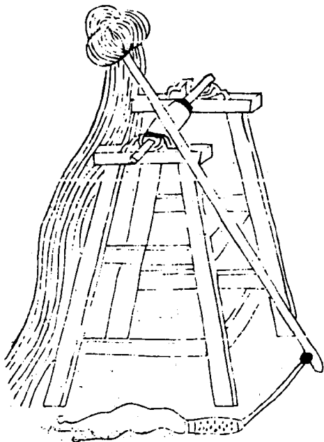
單稍砲
