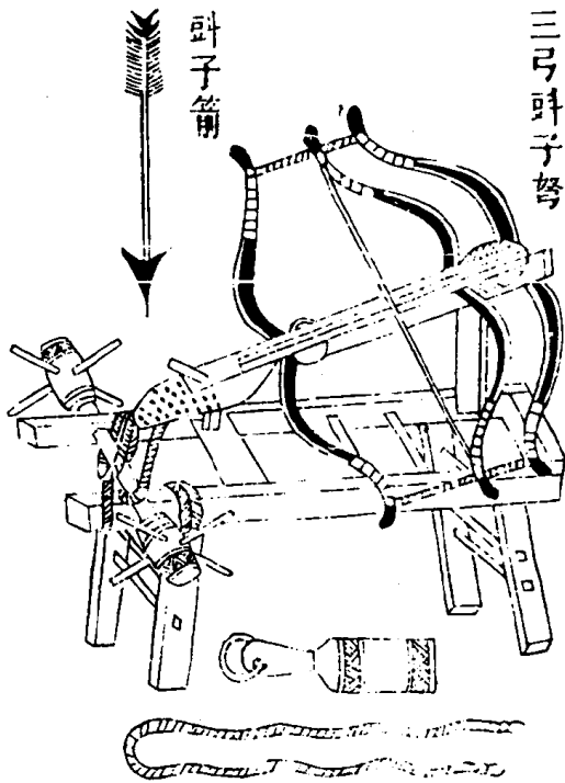
三弓射子弩
