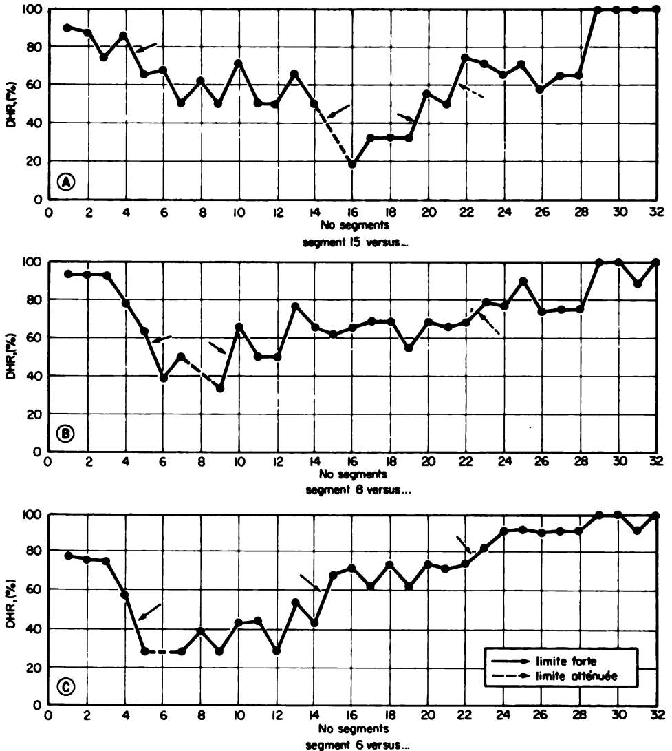
Figure 6. Interprétation graphique de la distance de Hamming relative selon un regroupement diôique: limite forte →; limite atténuée - - ->.
