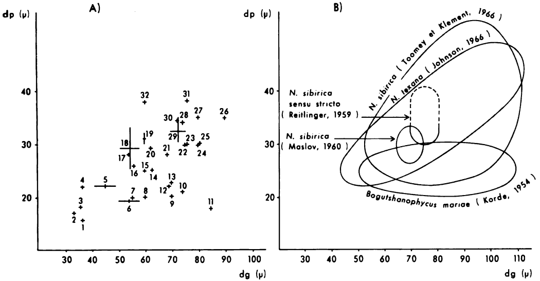
Figure 2. Rapport entre le diamètre du tube interne ( d_p ) et le diamètre du tube micritisé ( d_g ) chez nos spécimens de Nujia et chez les formes décrites dans la littérature 1 .
