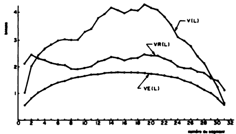
Figure 7. Profils de l'espérance mathématique VE(L) , de la valeur absolue V(L) et de la valeur relative de la limite VR(L) pour la ligne 63-73.
