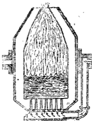
圖 鋼 迴 轉 爐 貝 ( 圖 五 第 )
