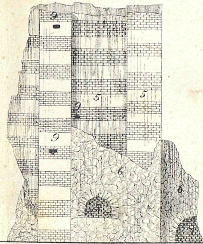
Фасадъ по линіи D. C.
