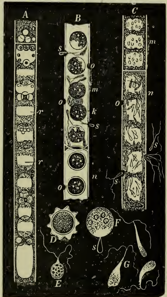
FIG. 10.— Sphaeroplea annulina .
