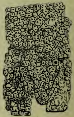
FIG. 140.— Pertusaria communis .
