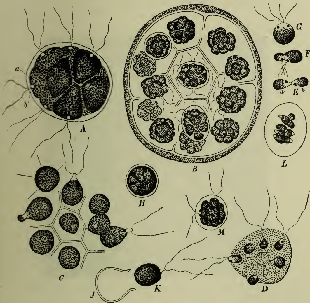
FIG. 45.— Pandorina morum .
