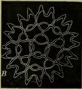
FIG. 50.— Pediastrum asperum .
