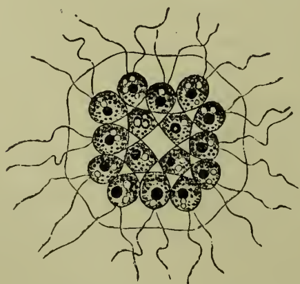
Fig. 44.— Gonium pectorale .
