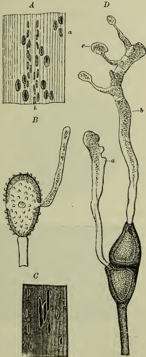
FIG. 146.— Puccinia graminis .
