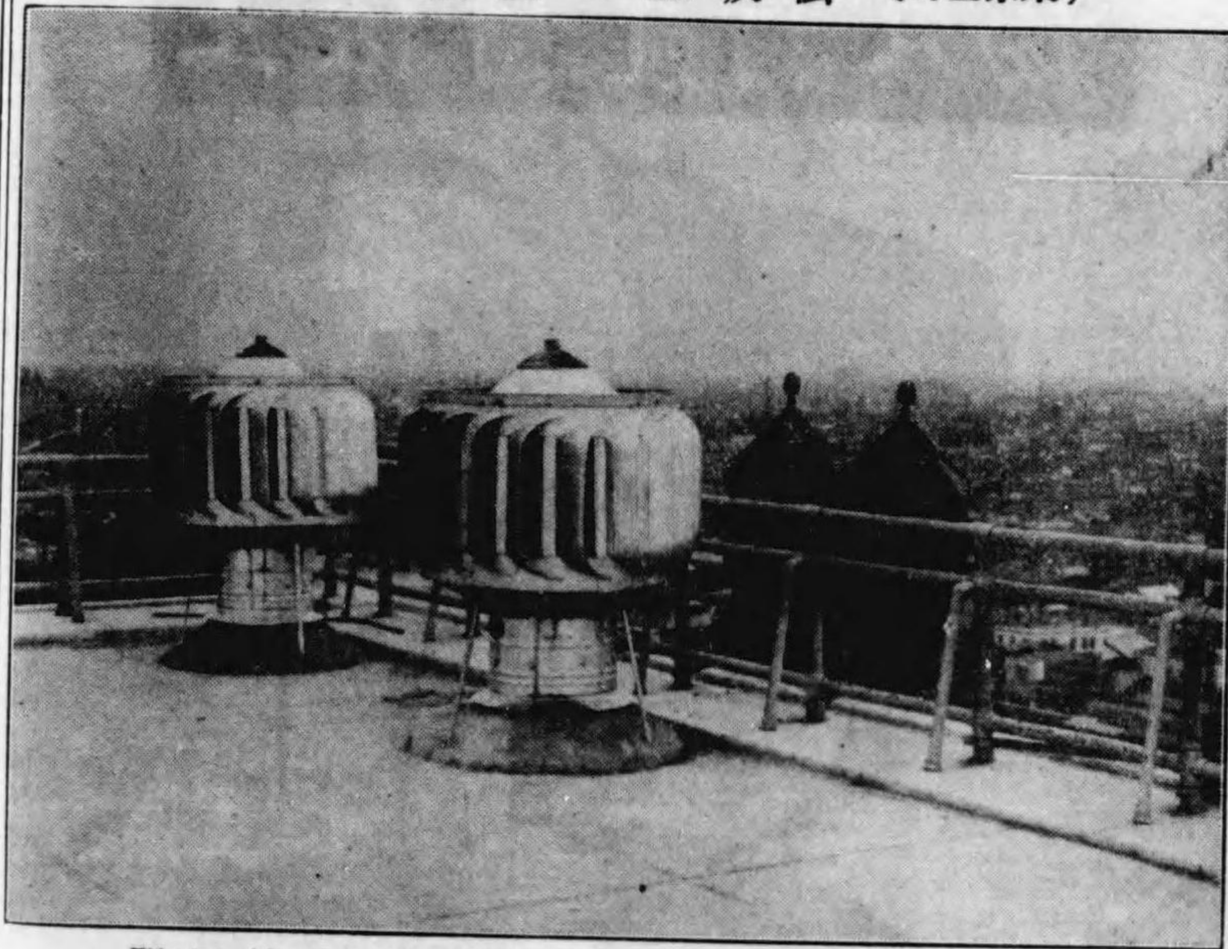
三星式通風頭三冠型換氣器
