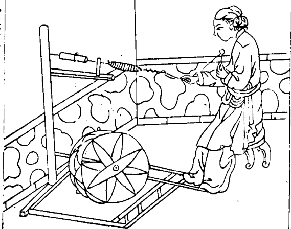
腳踏紡車圖
