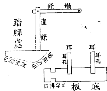
鞋板側面
