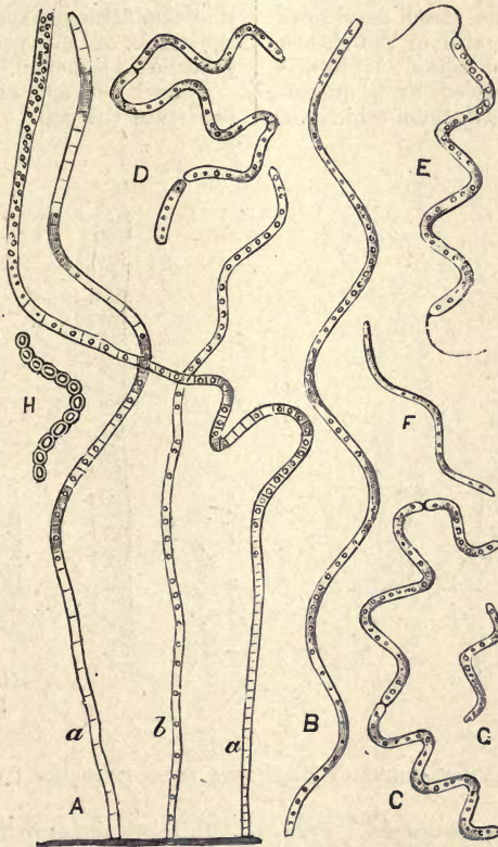
FIG. 215.— BEGGIATOA ALBA .
