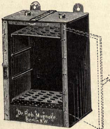
FIG. 251.—HOT-AIR STERILISER.
