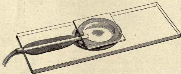
FIG. 56.—GAS CHAMBER.
