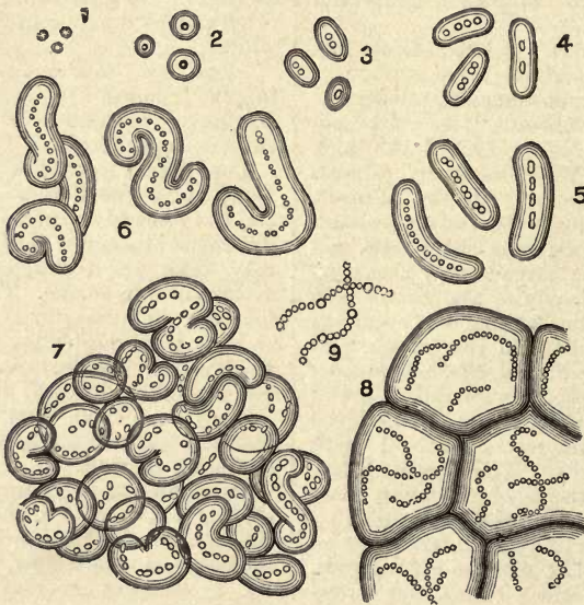
FIG. 219.—LEUCOCOCUS MESENTEROIDES.
