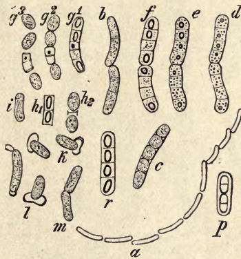
FIG. 4.—BACILLUS MEGATHERIUM.
