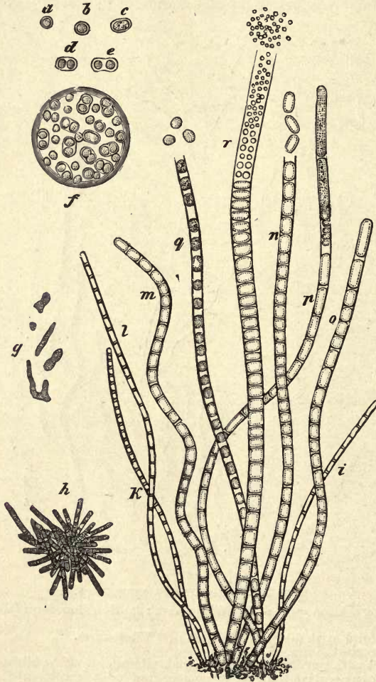
FIG. 218.—CRENOTHRIX KÜHNIANA.
