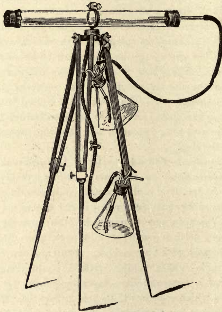
FIG. 71.—HESSE'S APPARATUS.
