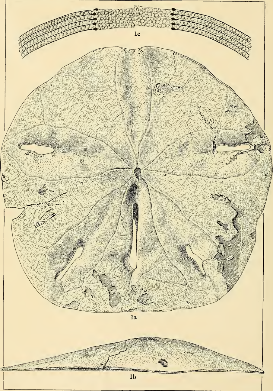
PLEISTOCENE ECHINOIDEA.
