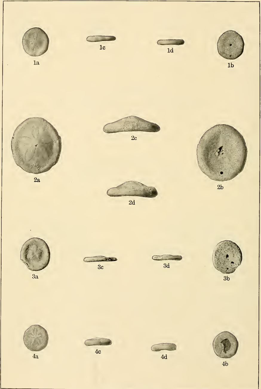
OLIGOCENE ECHINOIDEA.
