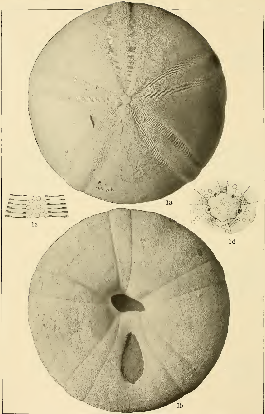
OLIGOCENE ECHINOIDEA.
