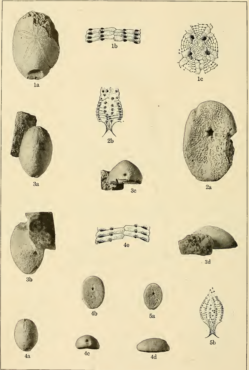
EOCENE ECHINOIDEA.
