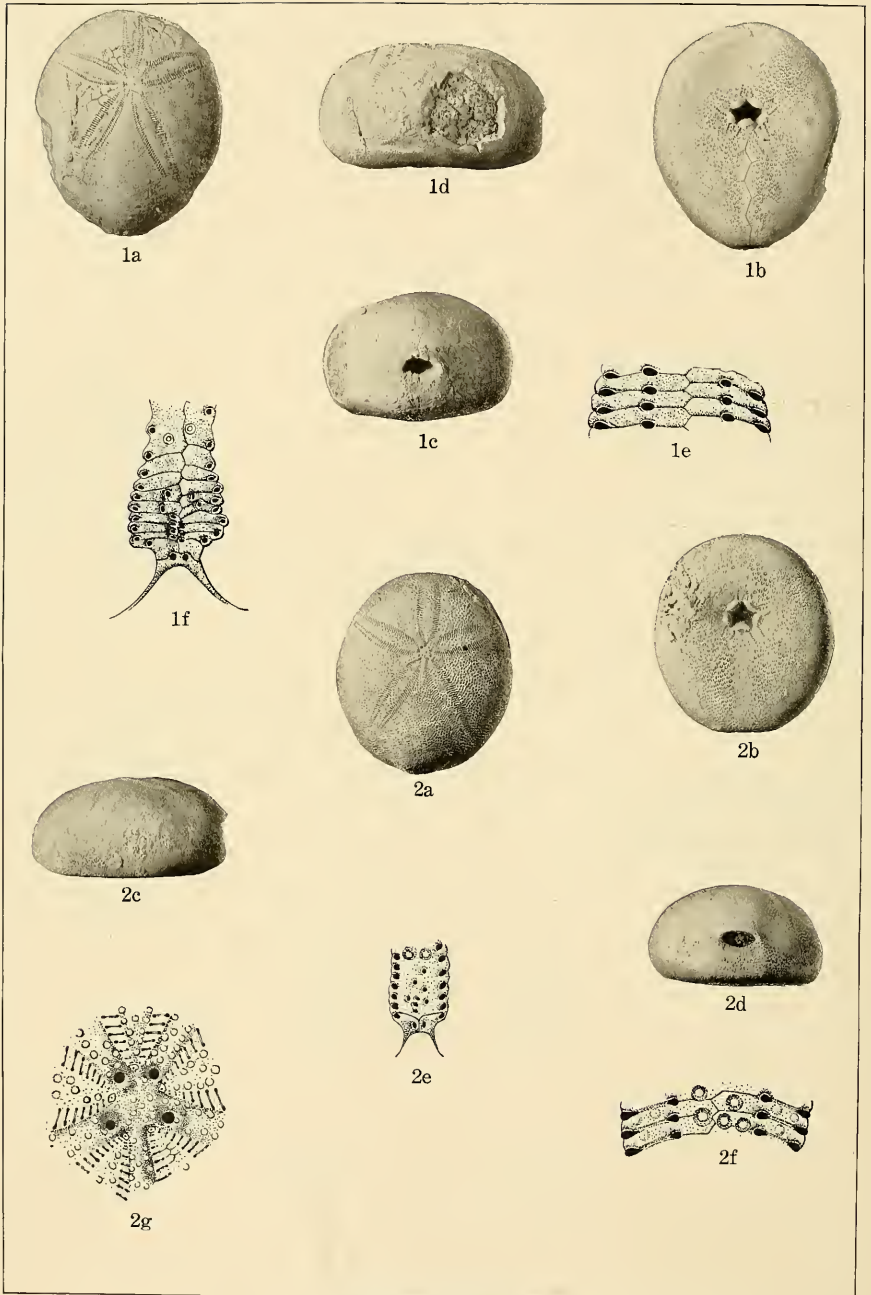
EOCENE ECHINOIDEA.
