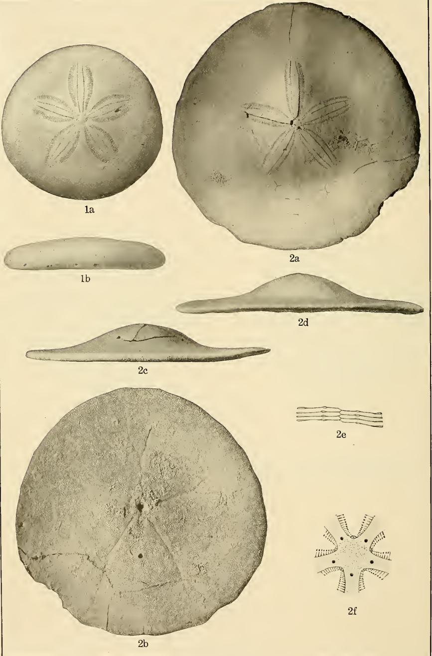
EOCENE ECHINOIDEA.
