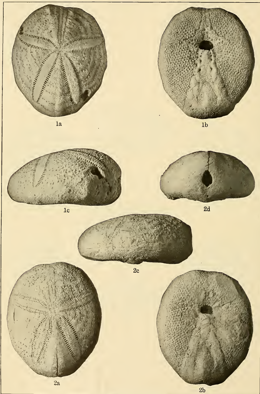
OLIGOCENE ECHINOIDEA.
