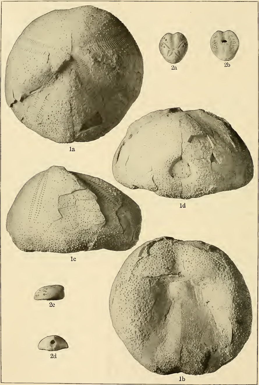
EOCENE ECHINOIDEA.
