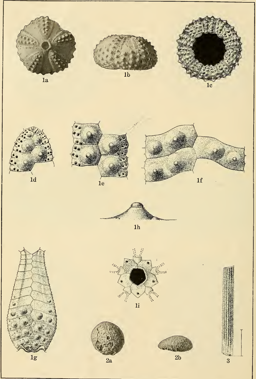
EOCENE ECHINOIDEA.
