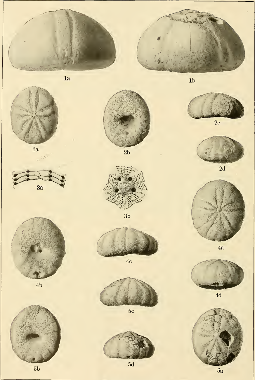
OLIGOCENE ECHINOIDEA.
