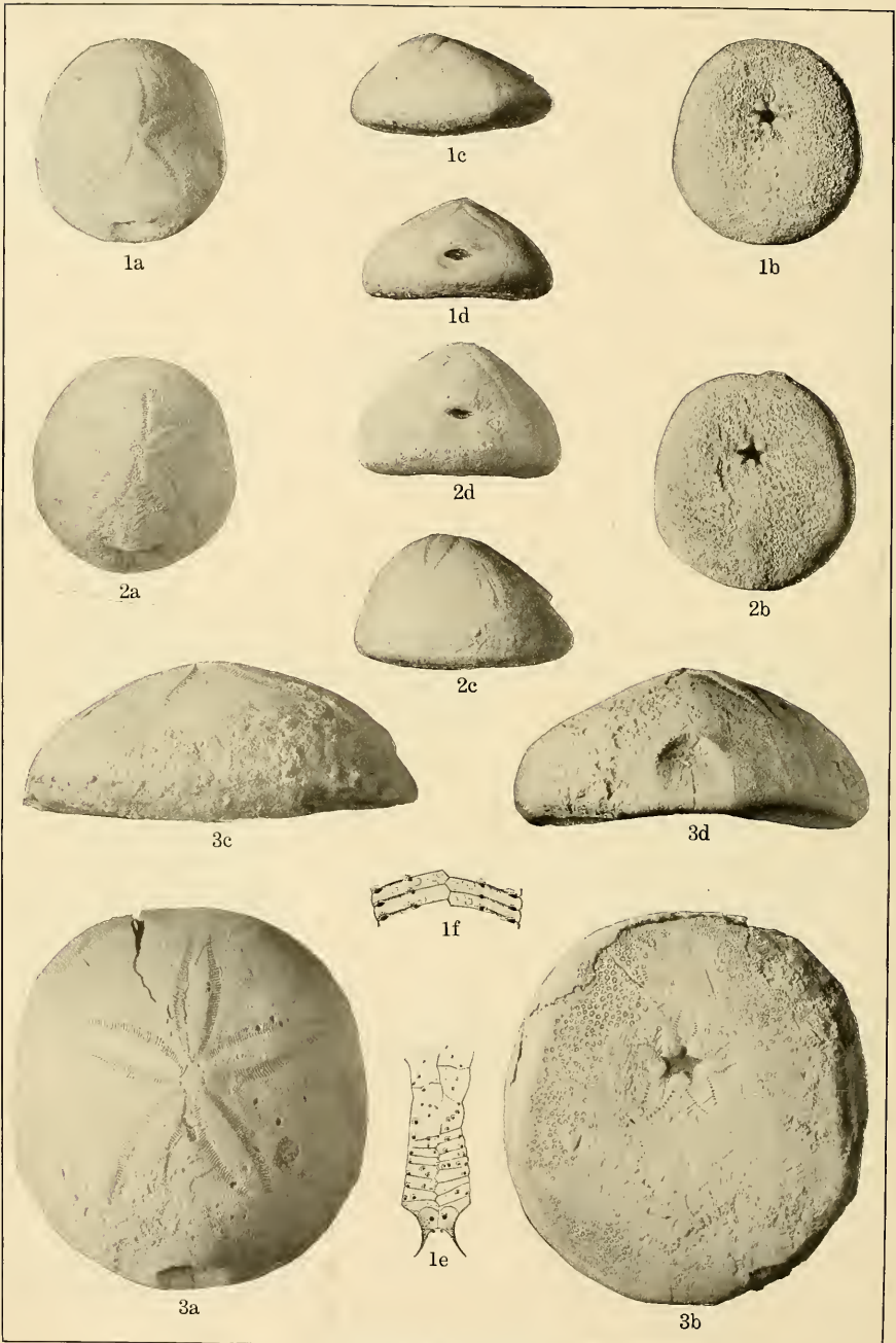
OLIGOCENE ECHINOIDEA.
