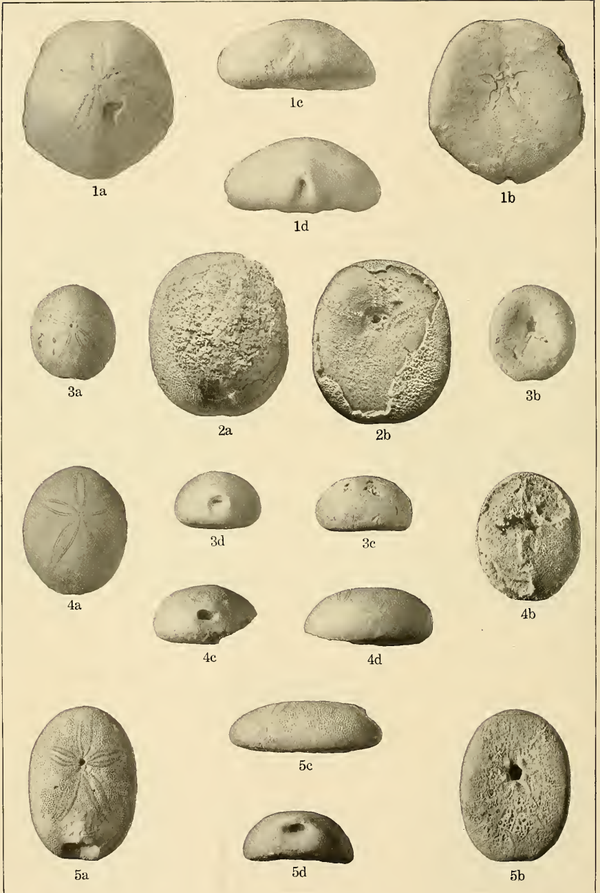
EOCENE ECHINOIDEA.
