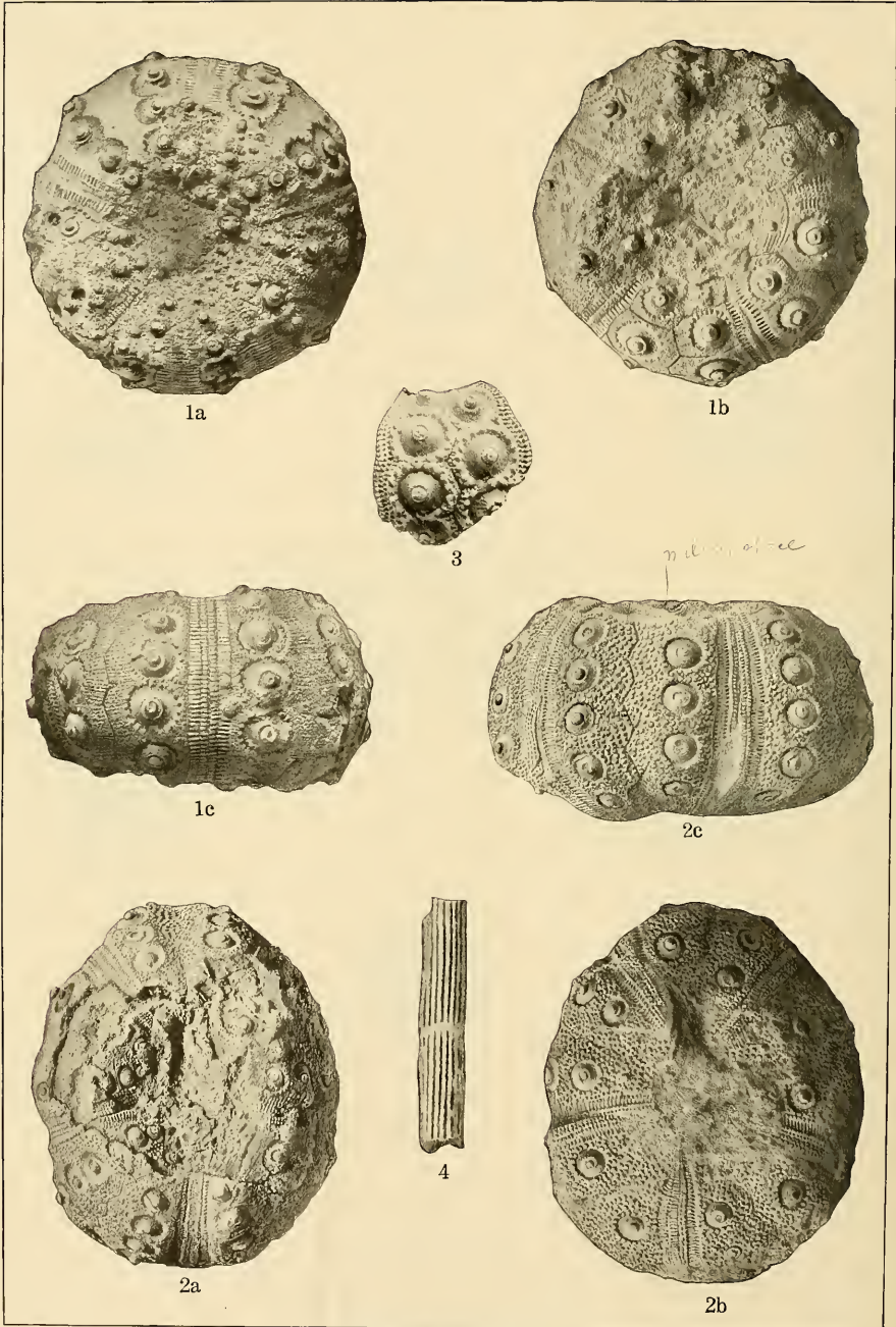
Eocene ECHINOIDEA.
