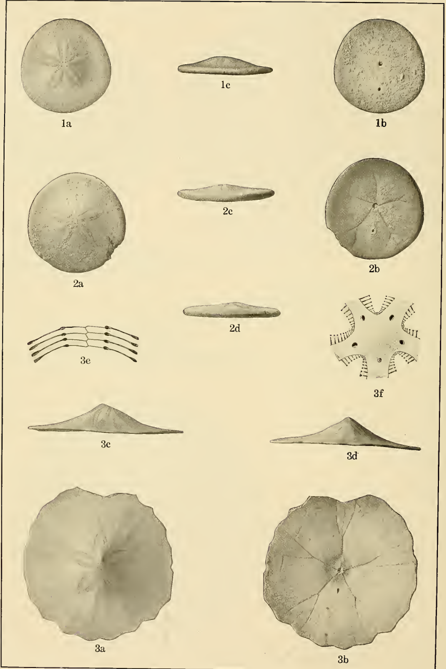
EOCENE ECHINOIDEA.
