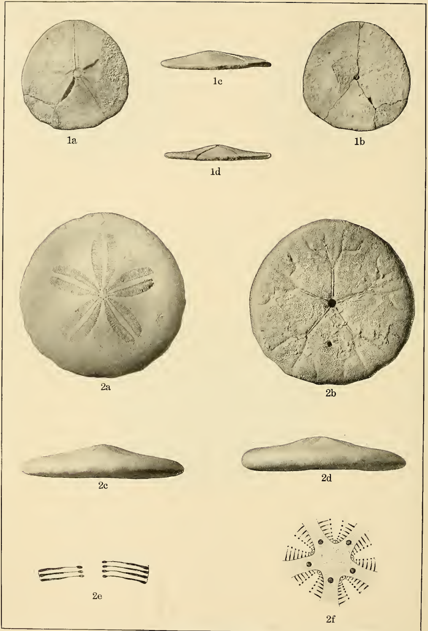
EOCENE ECHINOIDEA.
