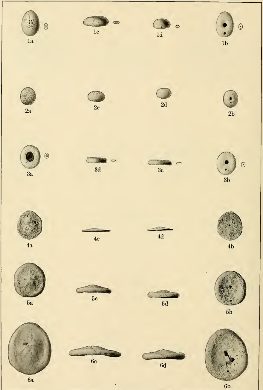
EOGENE ECHINOIDEA.
