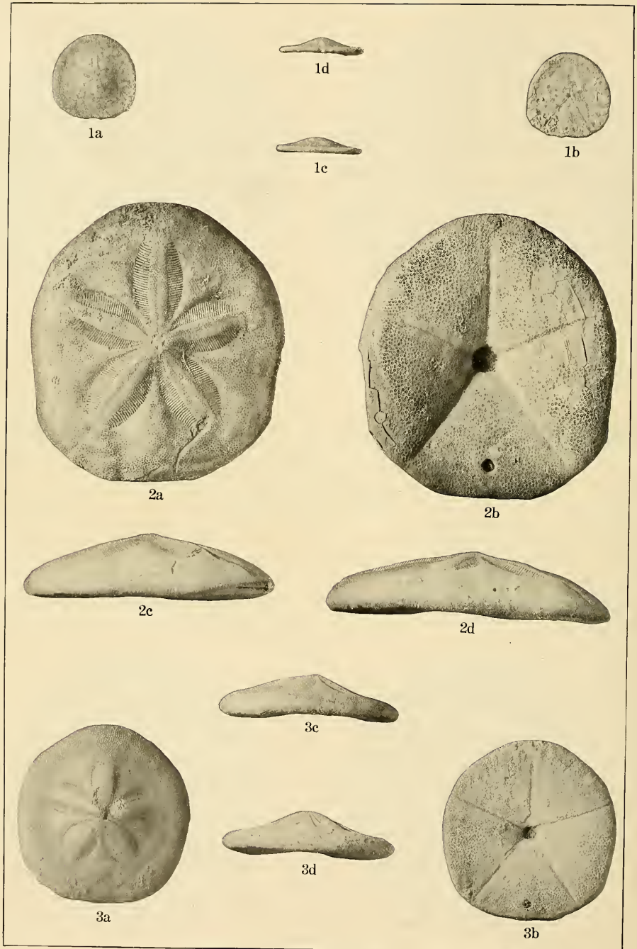
EOCENE ECHINOIDEA.
