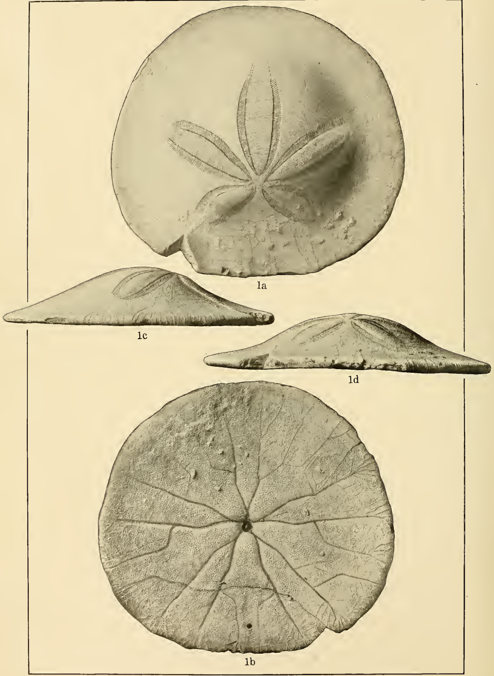
PLEISTOCENE ECHINOIDEA.
