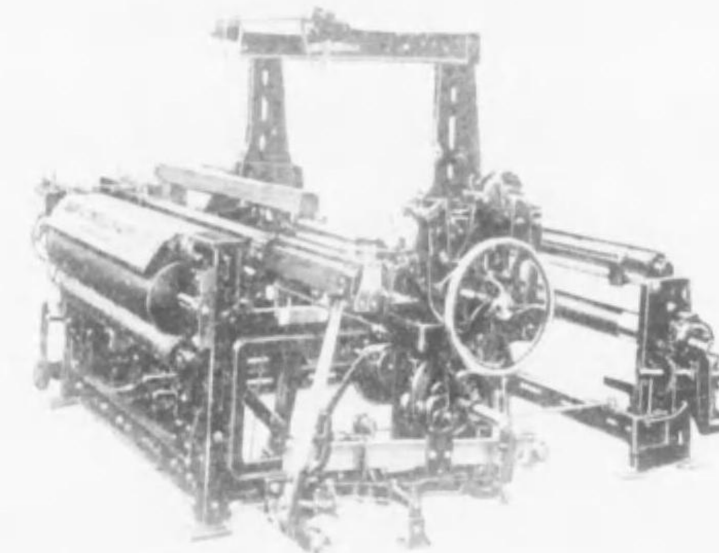
V型片側二丁杼人絹織機
