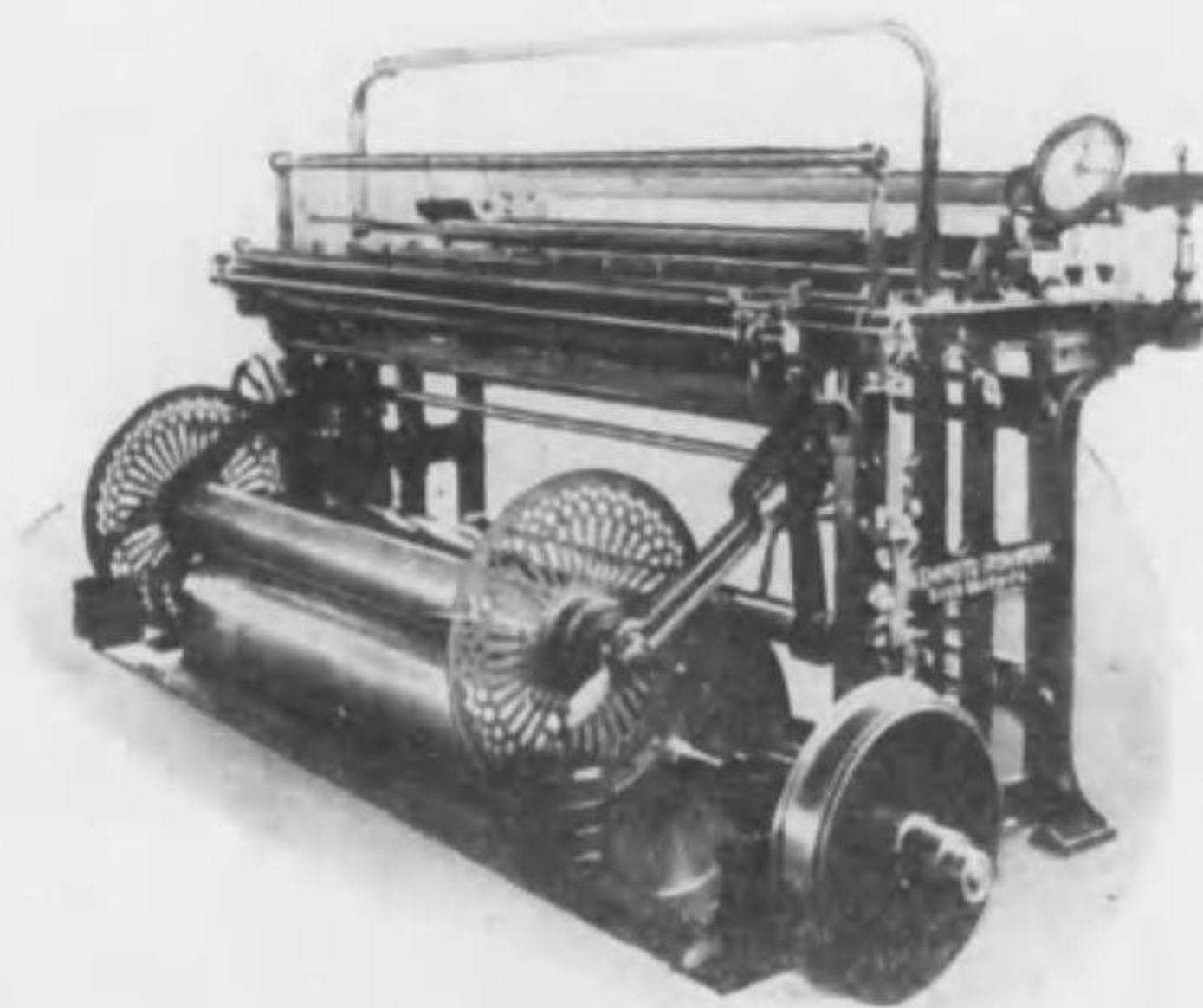
各種經糸用高速度整經機
