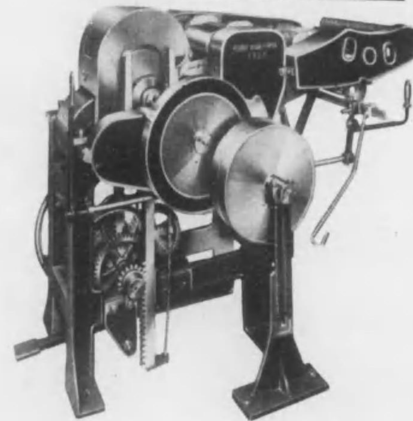
スライバーラツプマシン
