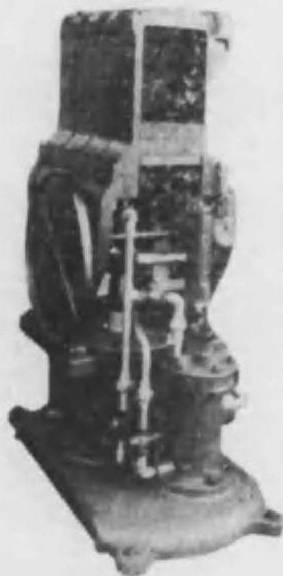
自動人絹玉繰機
