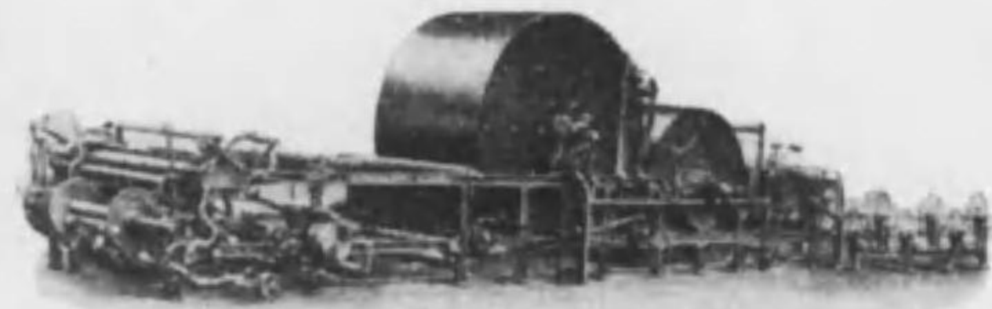
スラツシャー糊附機
