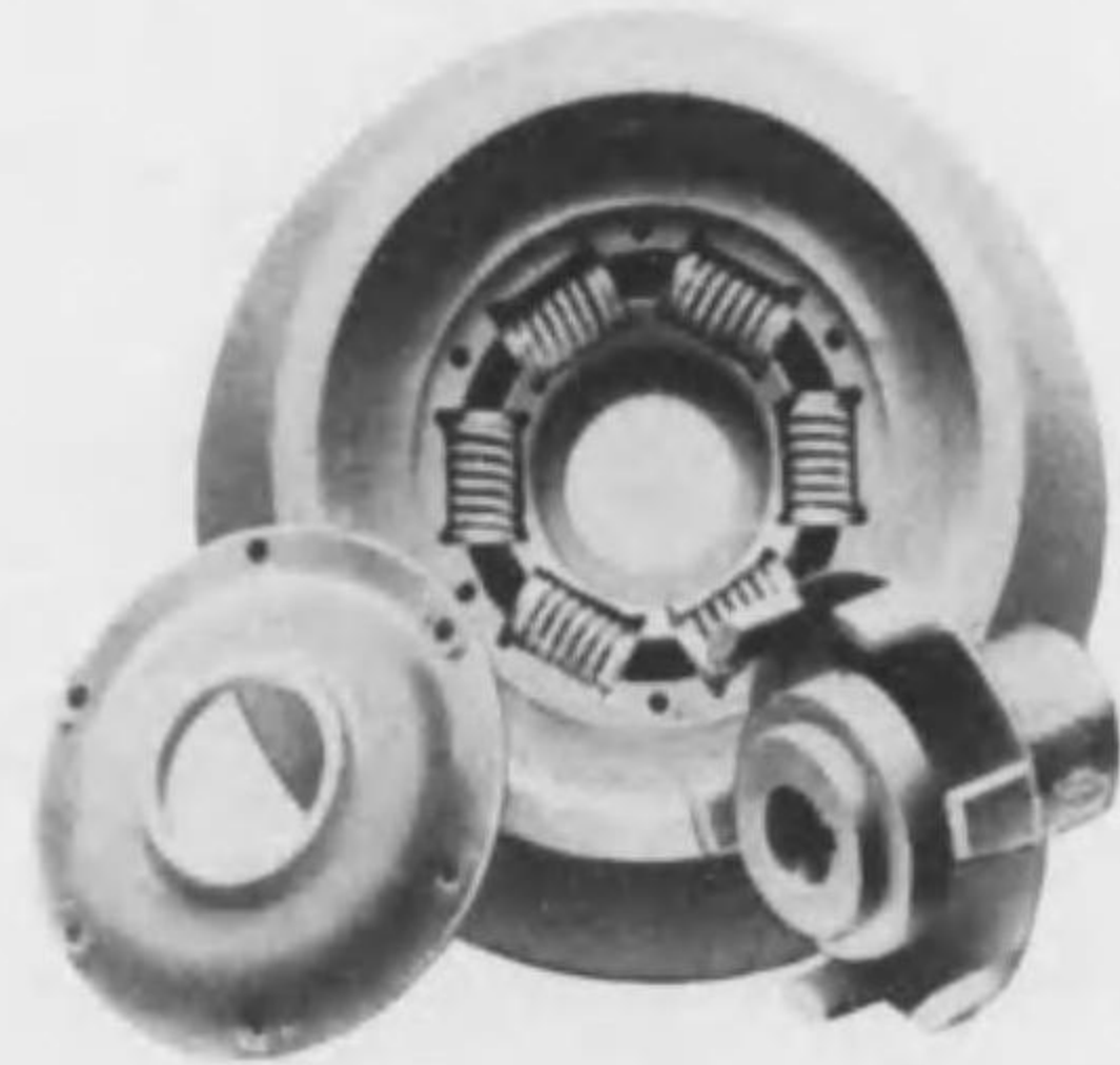
(分解圖)
