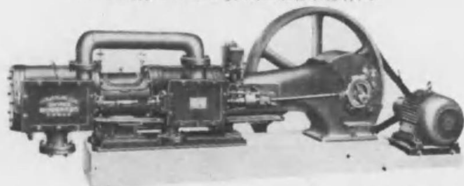
HVST型スライド弁式二段真空唧筒
