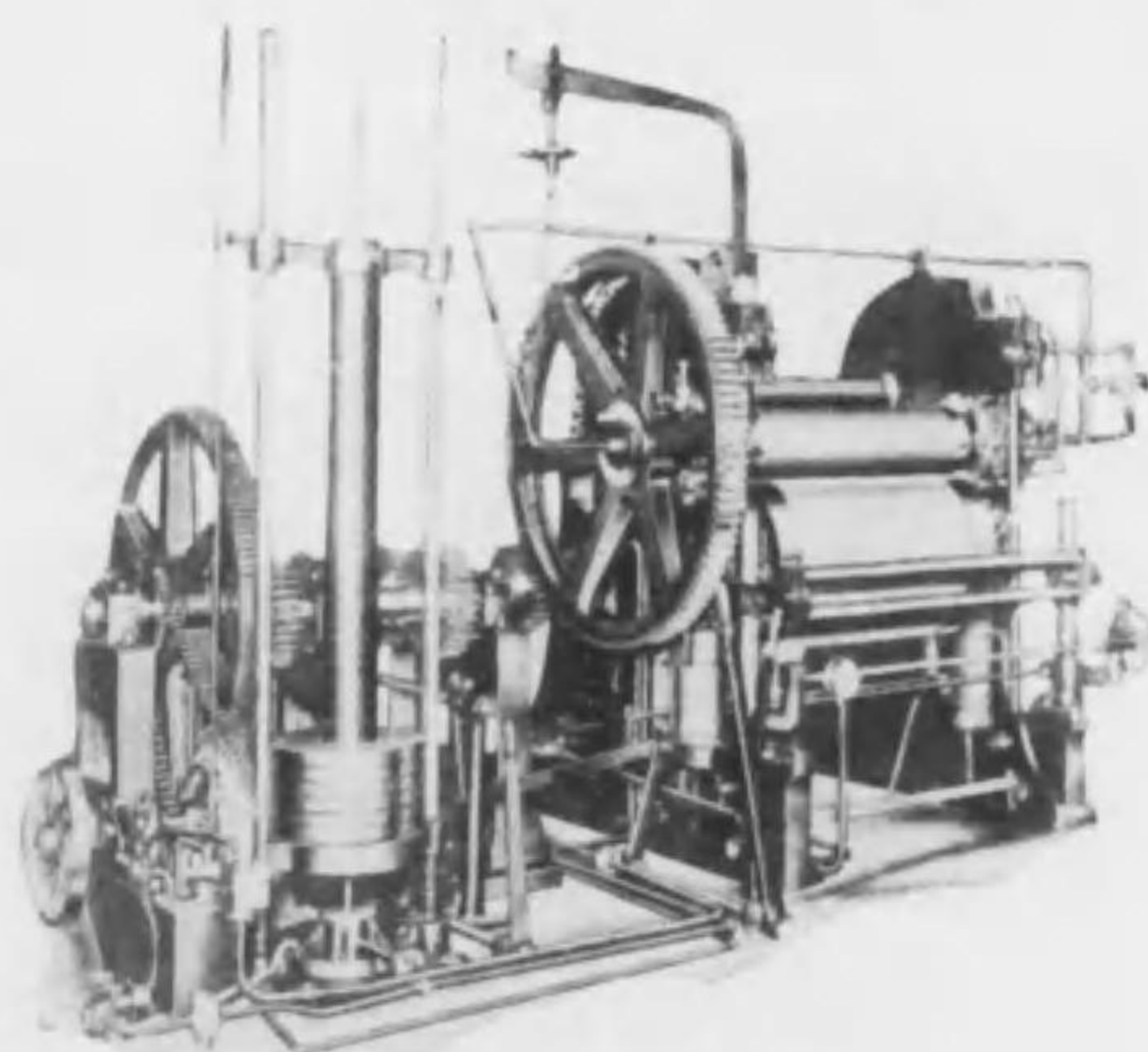
Hydraulic Schreiner Calender
