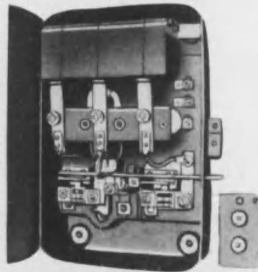
電磁開閉器
