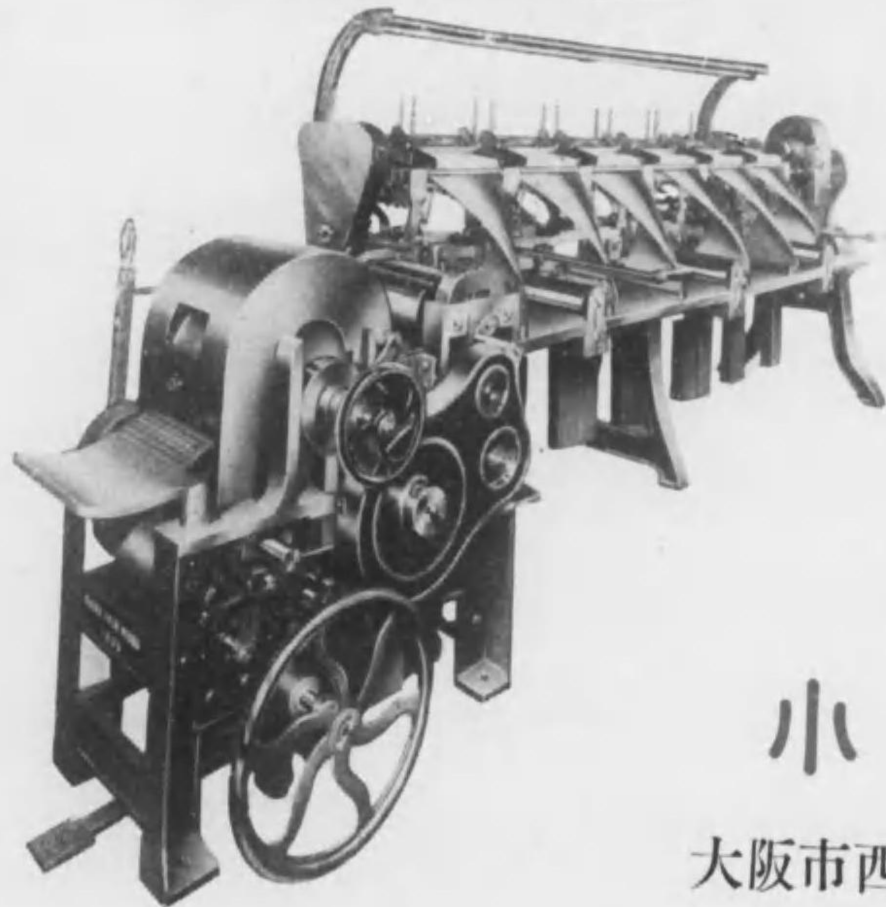
リボンラツプマシン
