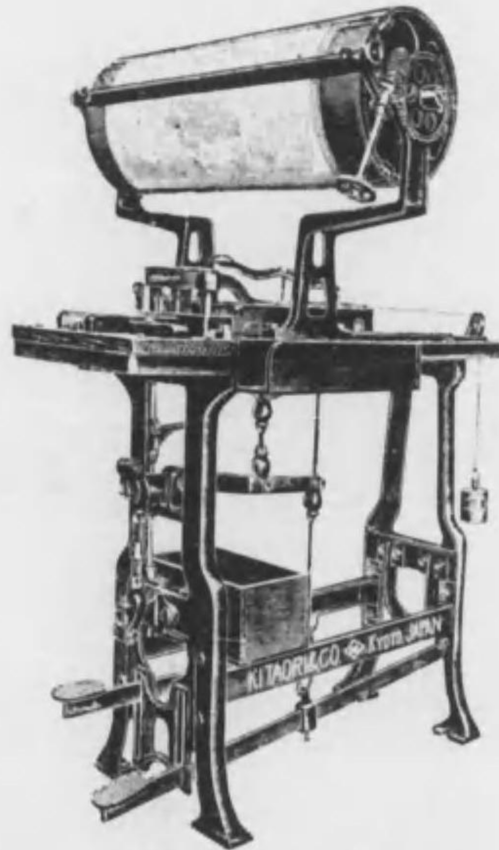
ピアノマシン紋紙穿孔機
