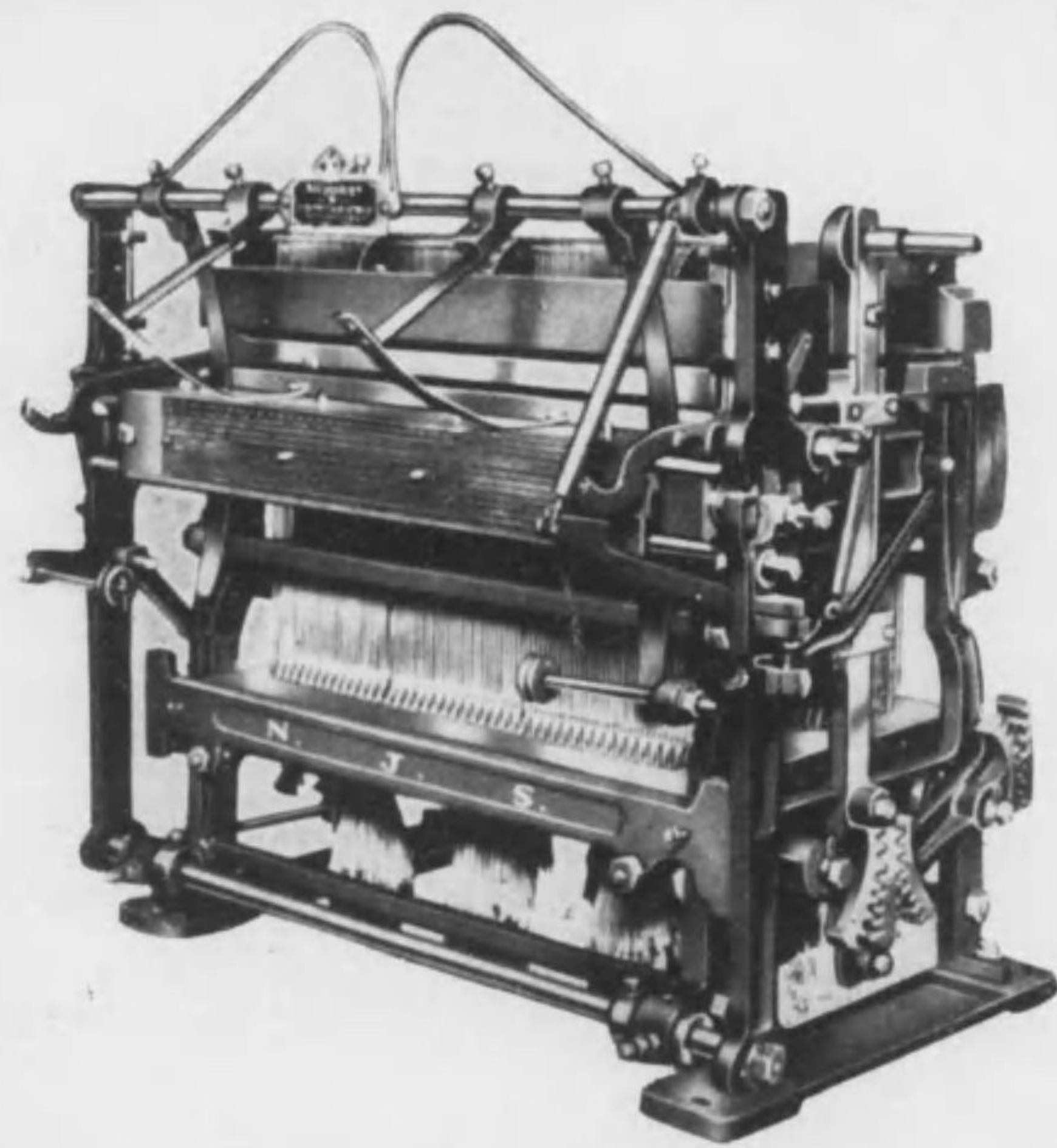
B型兩口(中口)ジャカード機 (二本ロット式)
