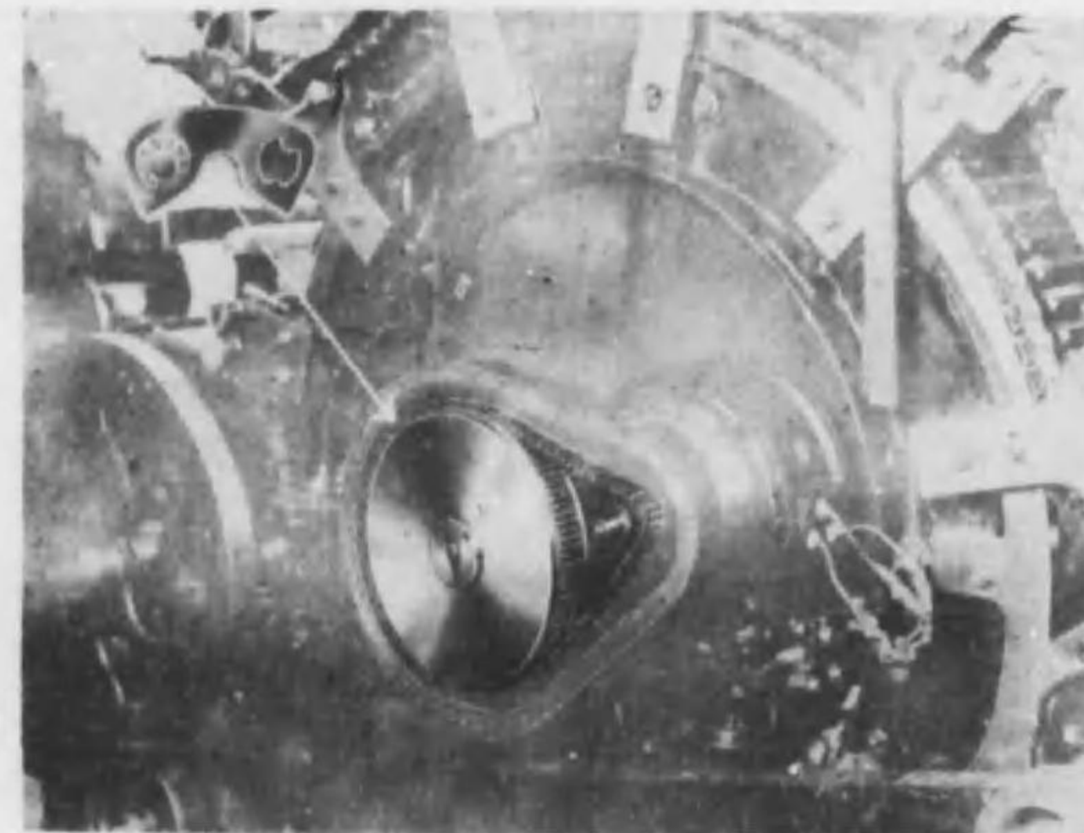
写真 徳島紡績ニ於ケル椿本製サイレントチェーンニ依ルカード單獨運轉装置ヲ示ス
