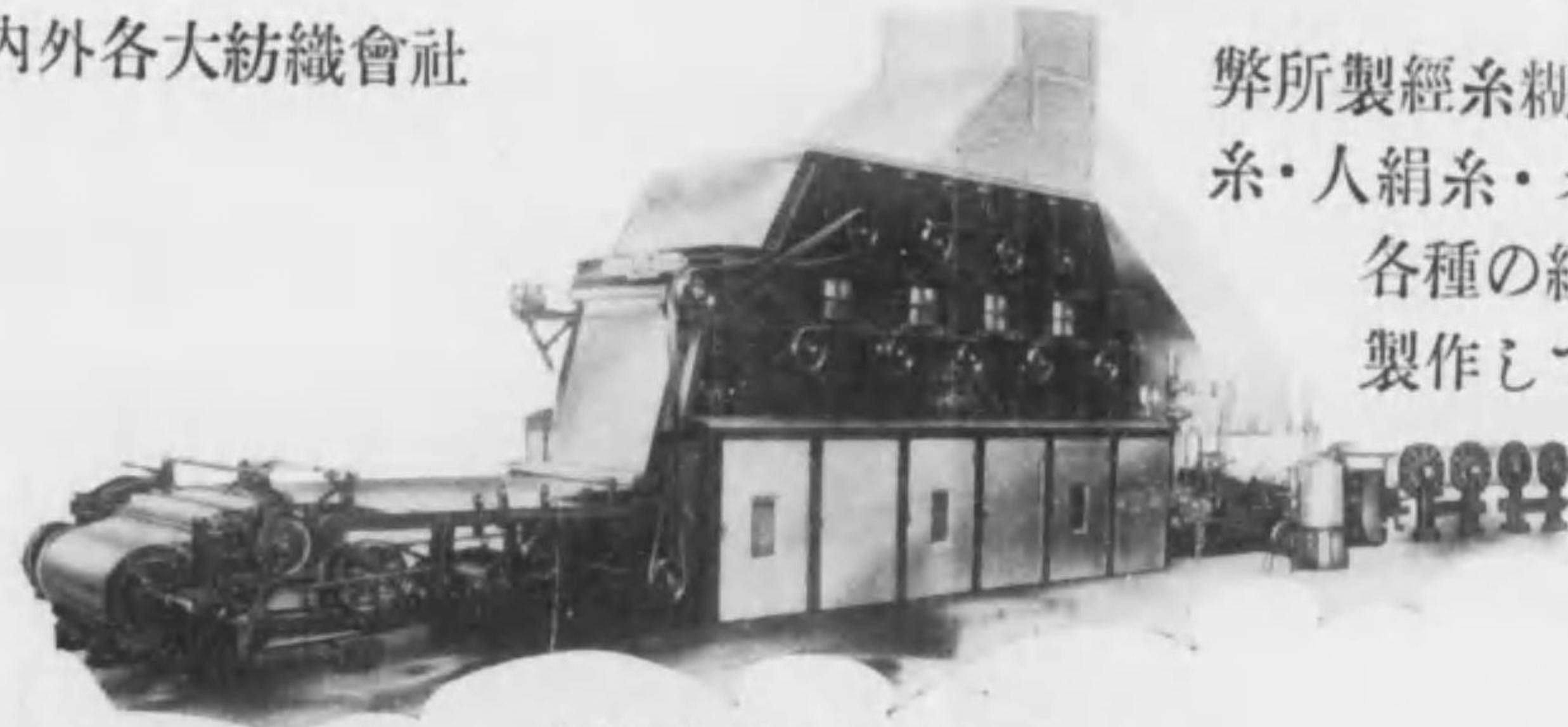
熱風式經糸糊附乾燥機
