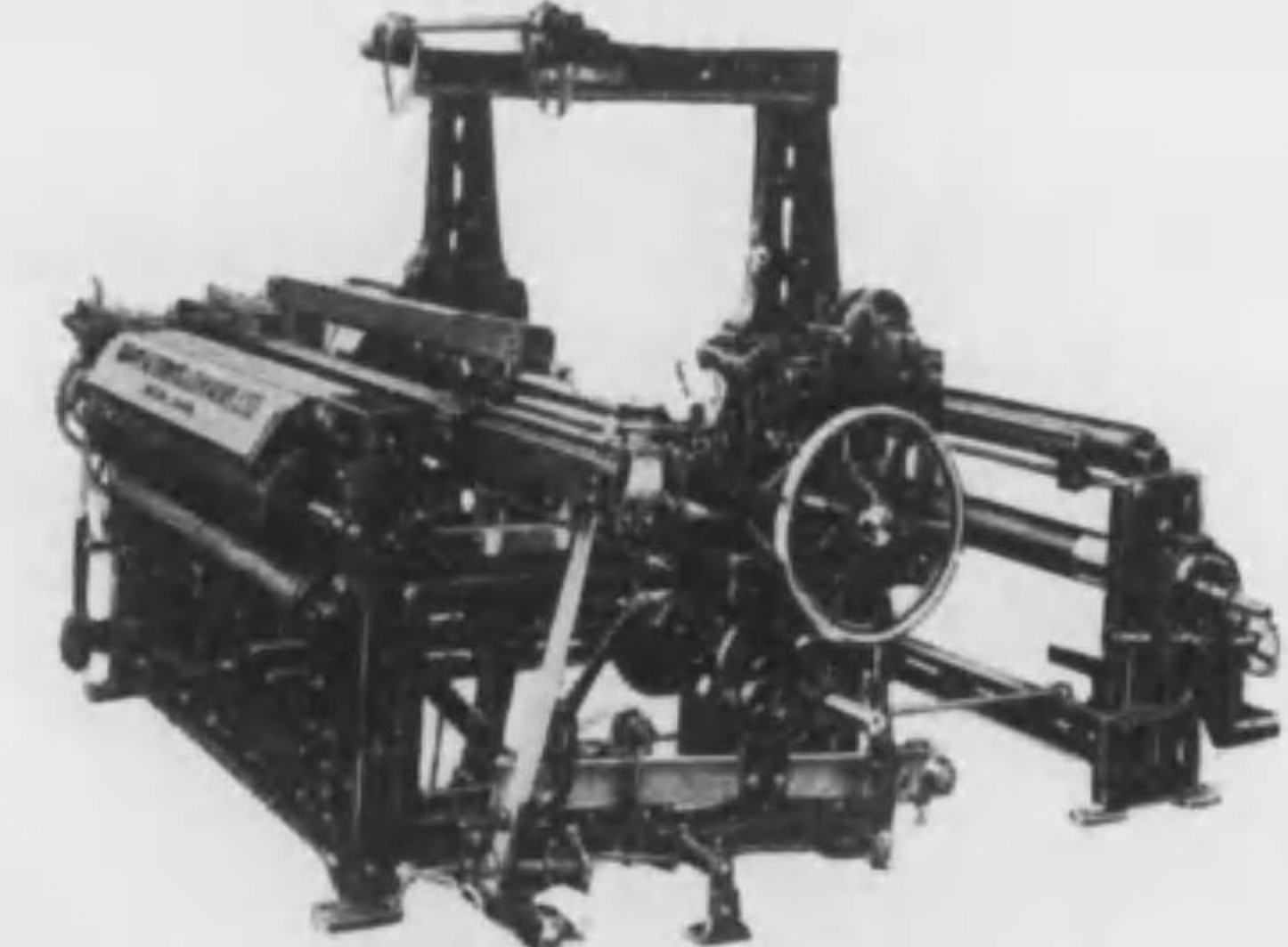
V型片側二丁杼人絹織機
