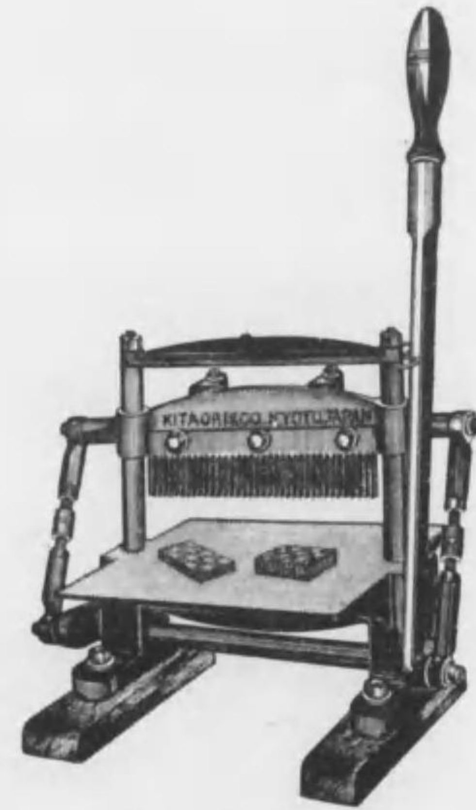
織物見本切斷器
