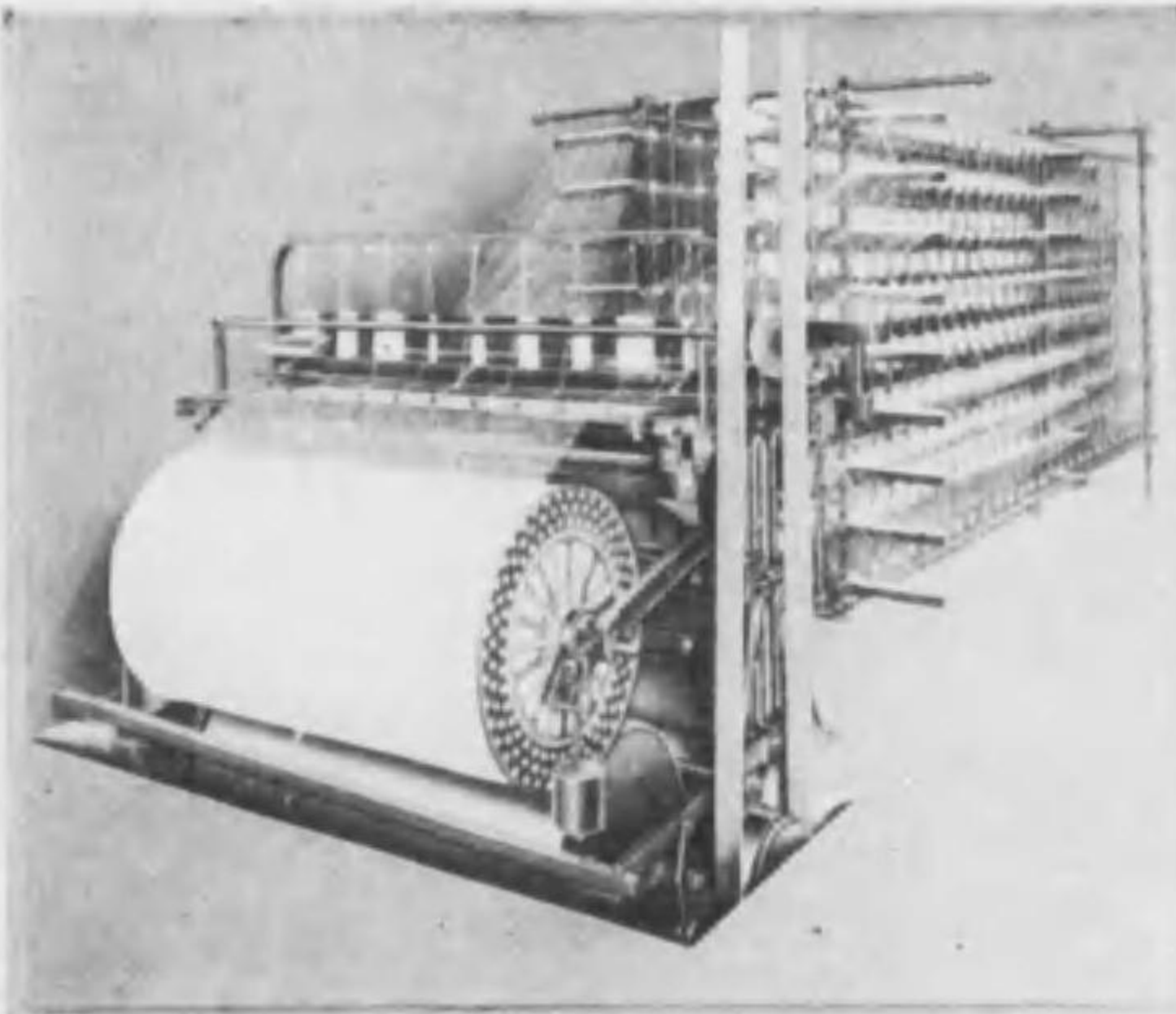
ハイスピード ワーバー
