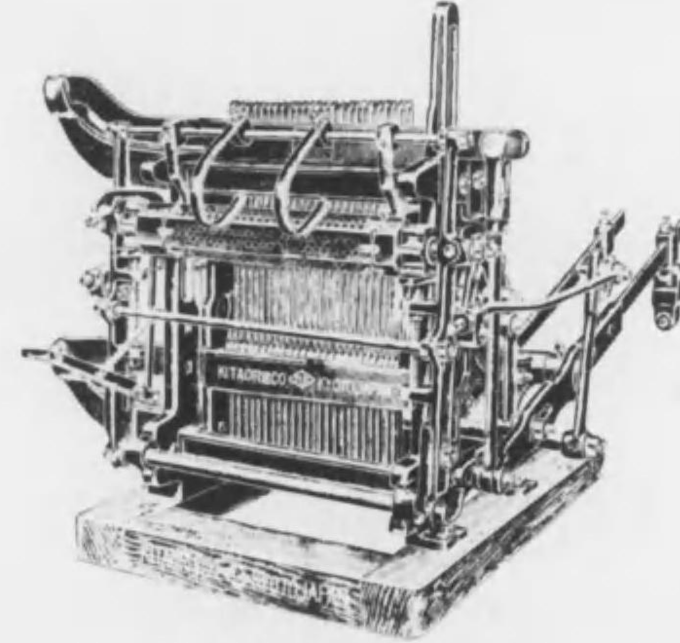
北織式高級ドビー機
