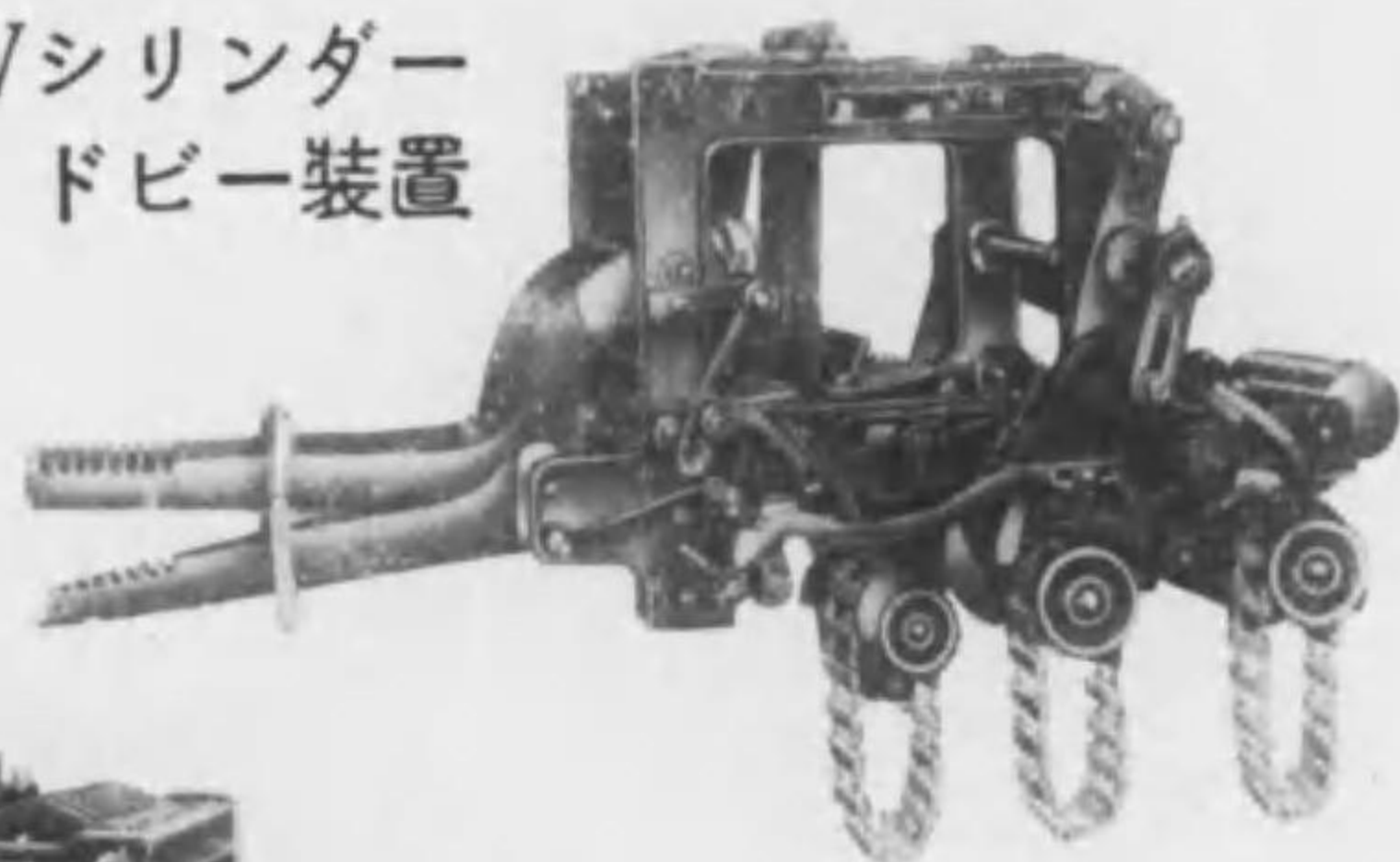
普通ドビー装置
