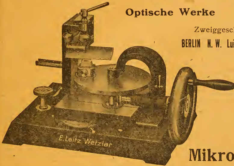
Rotationsmikrotom
