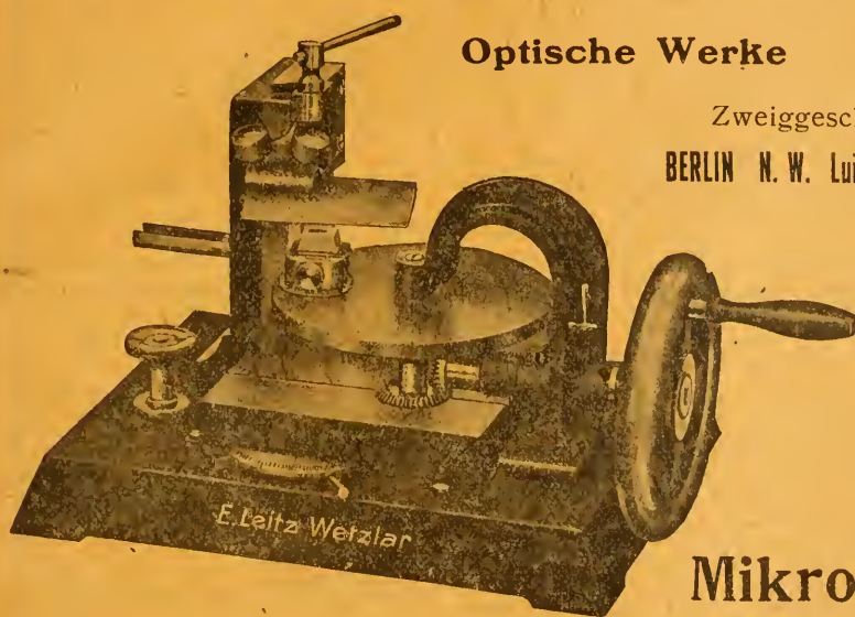
Rotationsmikrotom
