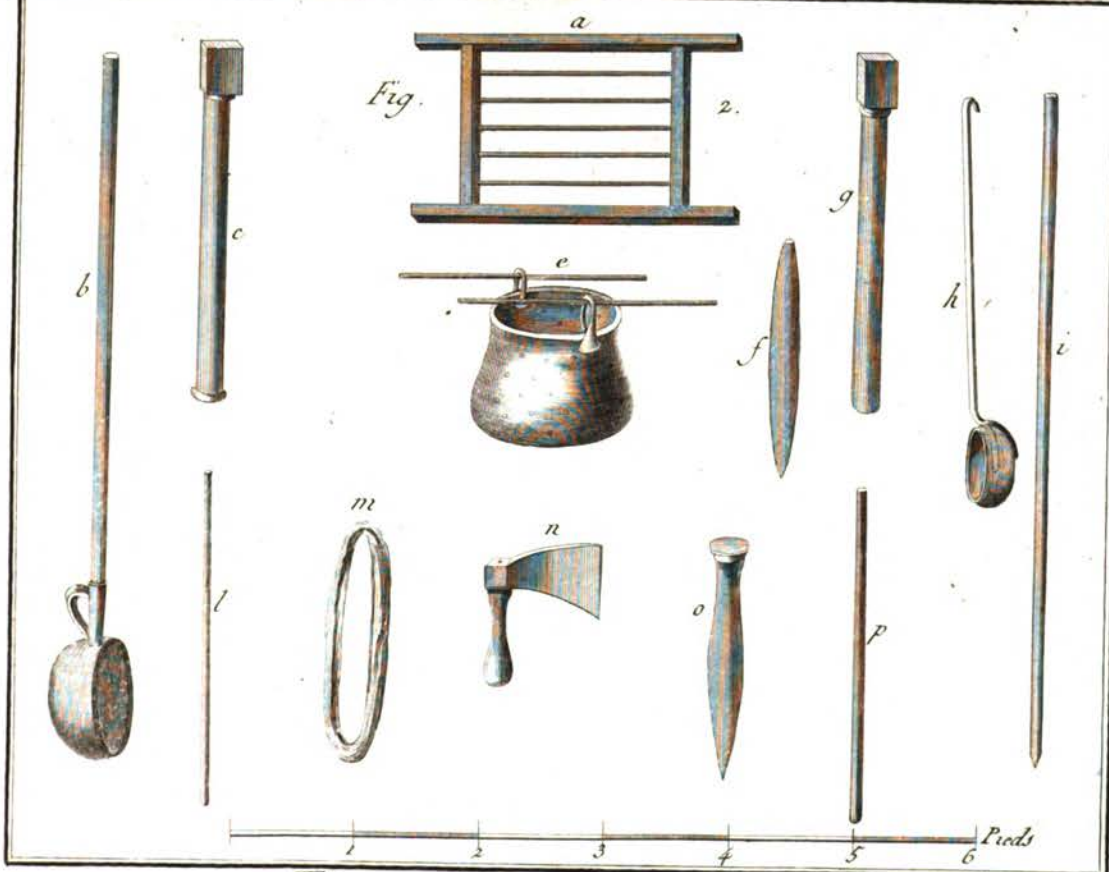
Teinturier, Atelier et Outils.
