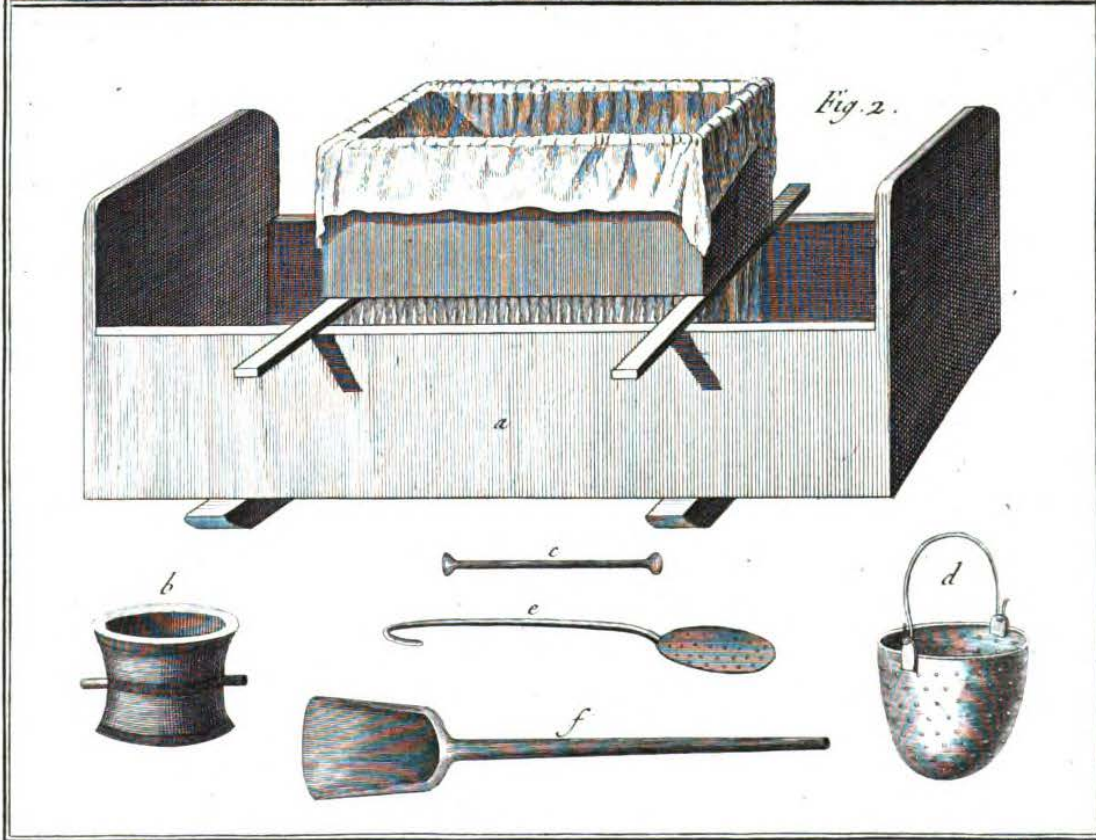
Teinturier, différentes préparations du Safranum et Outils.
