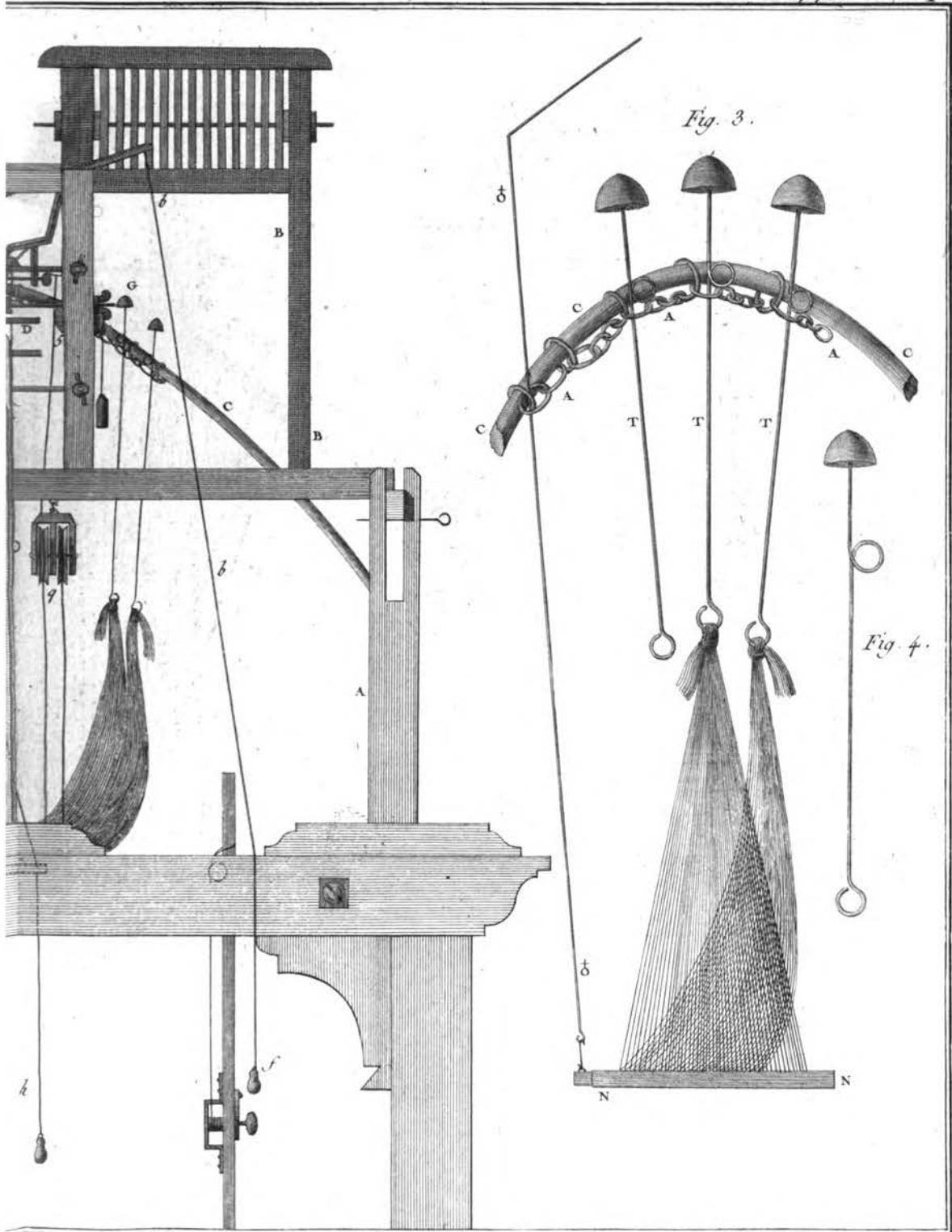
Machine pour dispenser d'un Tireur de Lacs.
