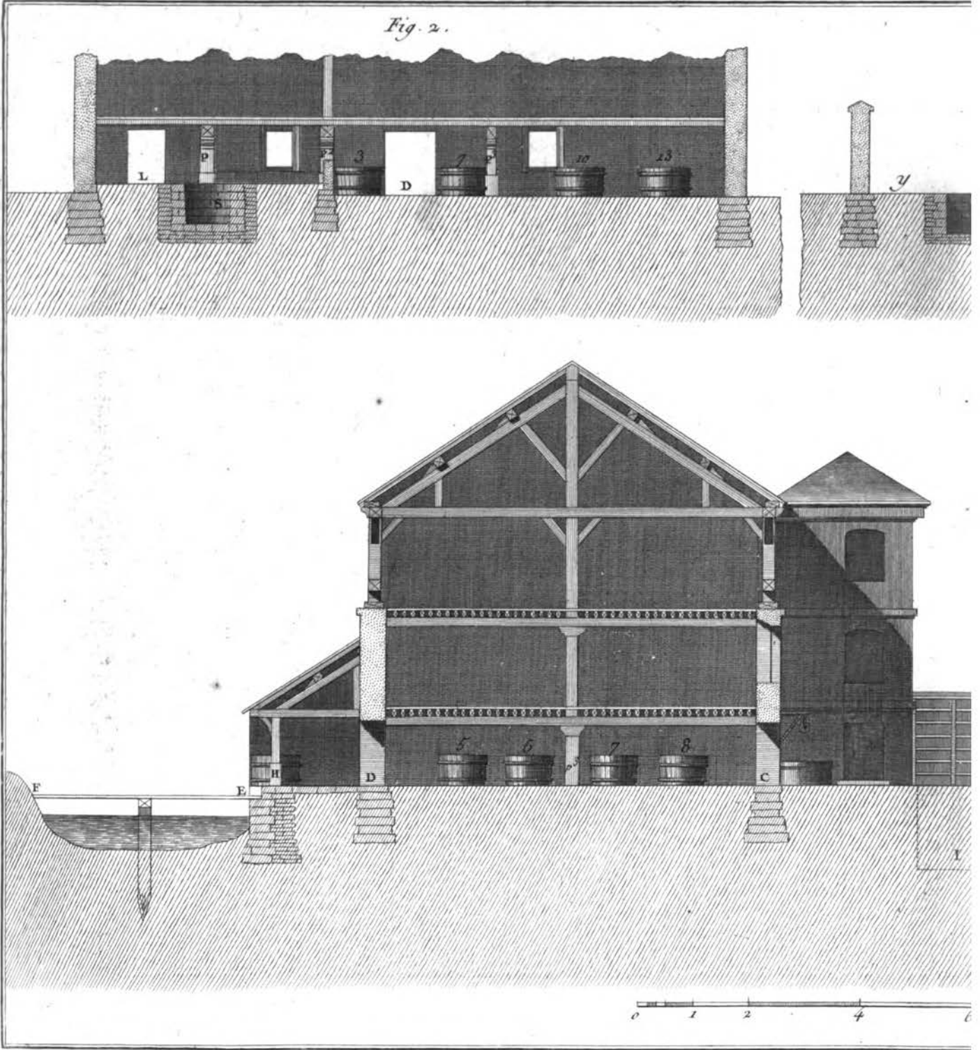
Tanneur, Coupe Longitudin
