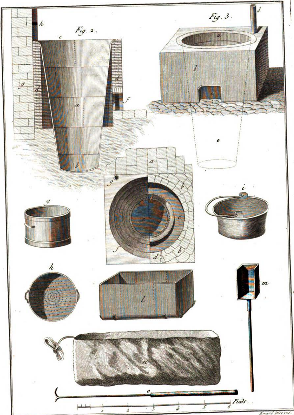
Teinturier de Riviere, Plans, Coupe et Elevation de la Cuve pour l'Indigo.
