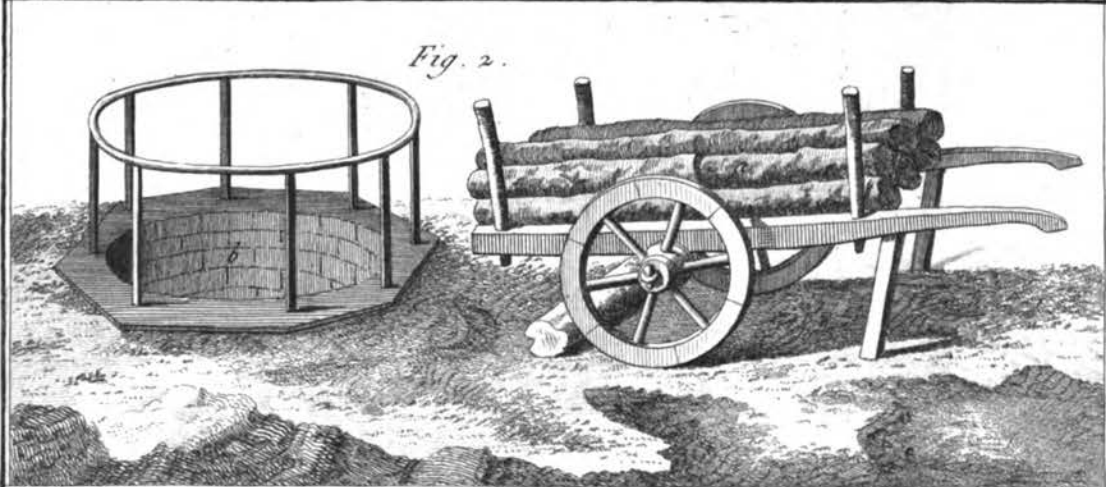
Teinture des Gobelins, Intérieur d'un Fourneau, Outils &c.
