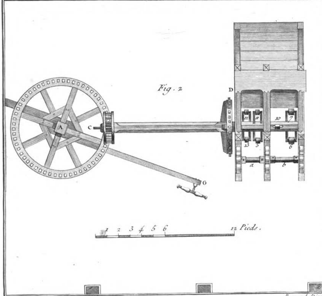
Chamoiseur, Moulin à Foulon.
