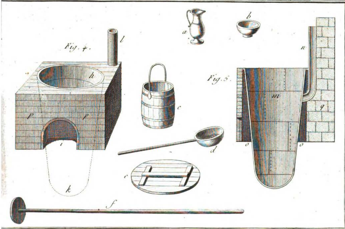
Différens Ateliers et Ustensiles.
