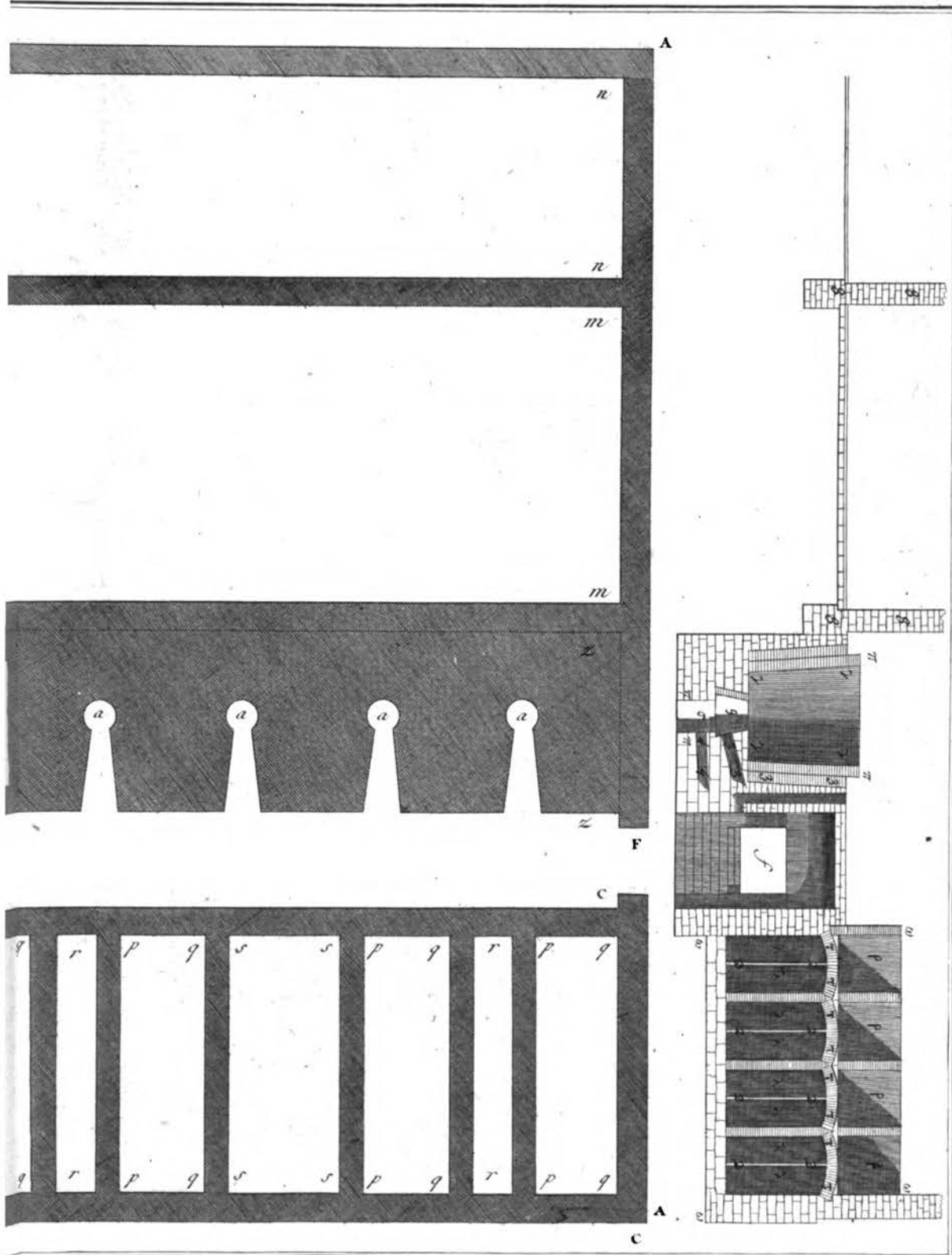
d'une grande Manufacture de Savon
