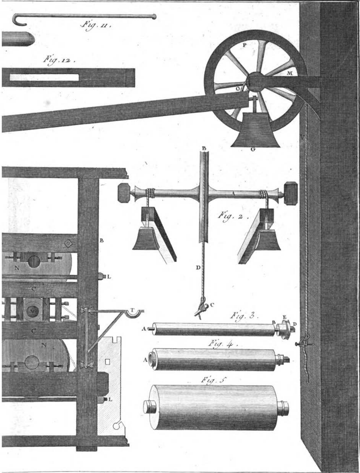
Cylindre à Bascule et développemens .
