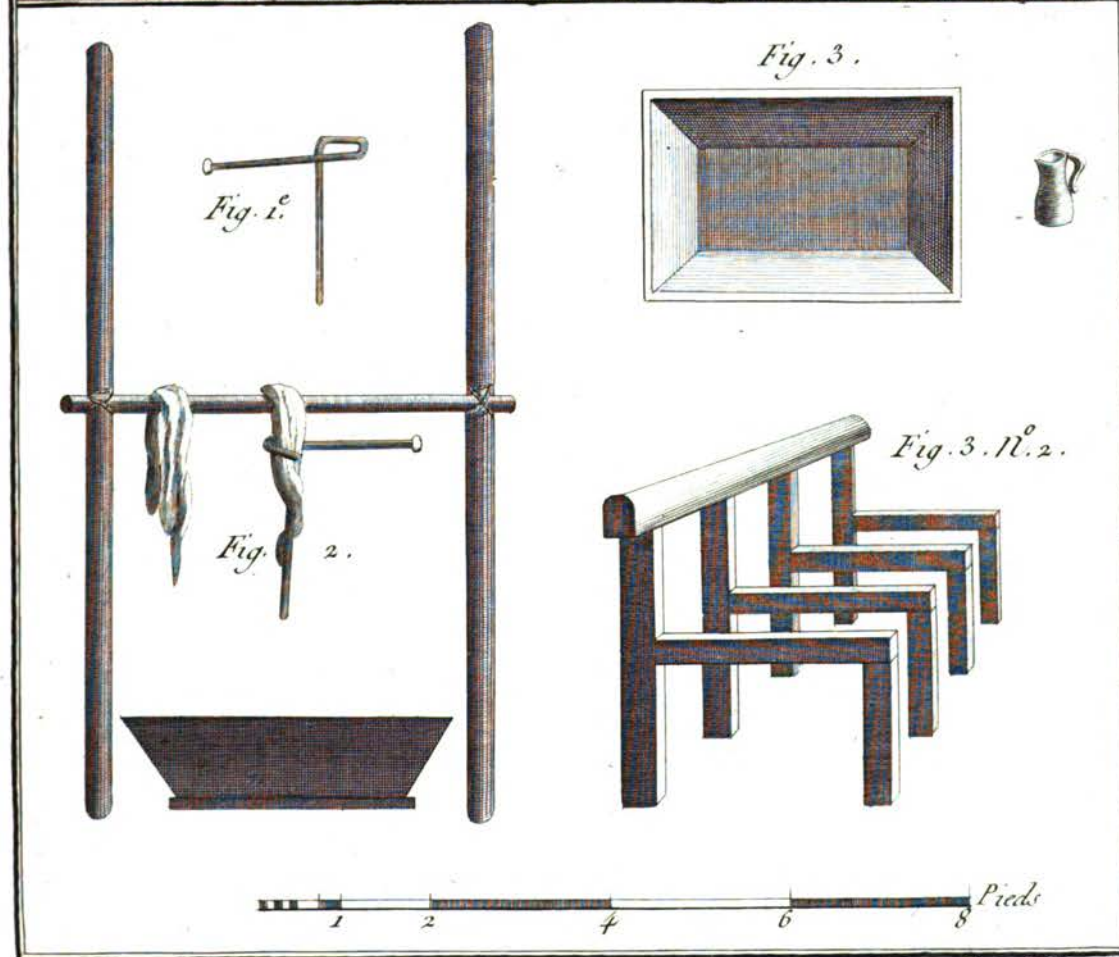
Maroquinier, l'opération de Teindre les Paux. Bernard Duvet.
