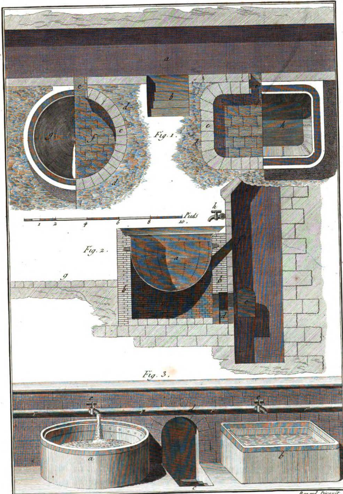
Teinturier de Riviere, Plans, Coupe et Elevations de différentes Chaudieres. 60.
