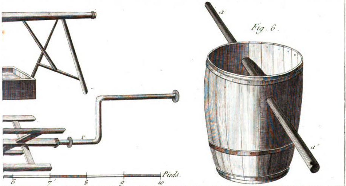
Chaudieres, Entrée des Fourneaux et Ustensiles.
