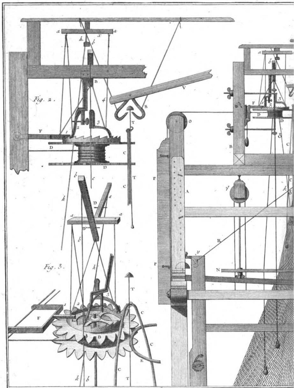
Élévation de la Machine pour dispens
