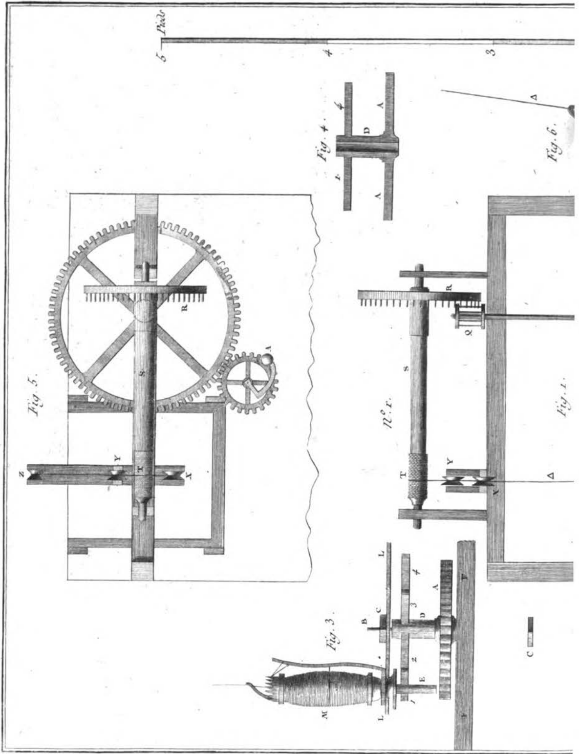
Machine à faire des Liacs
