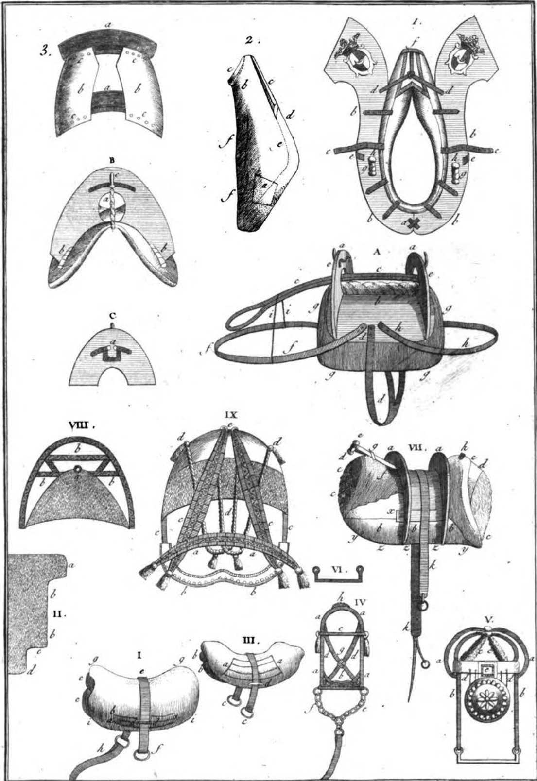
Sellier, suite du Travail du Bourrelier pour le Collier monté, le Bât, le Pannau &c.
