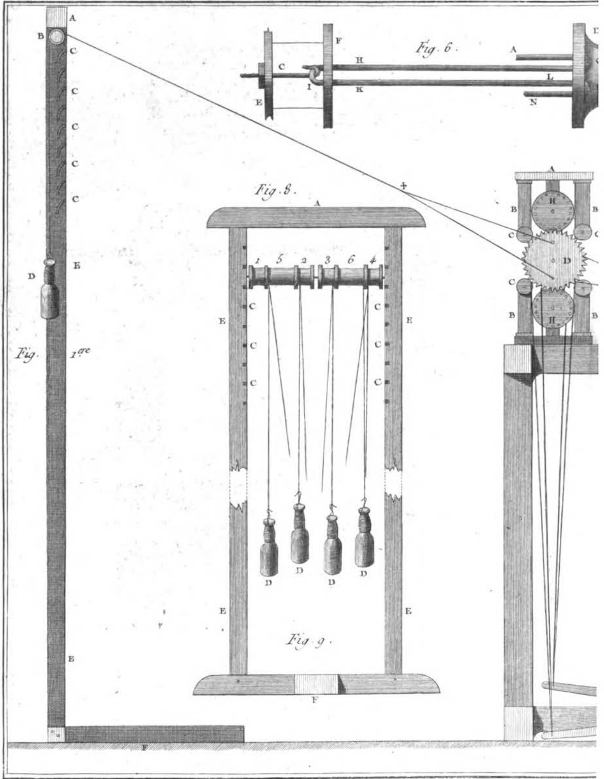
Machine nommée la Rave
