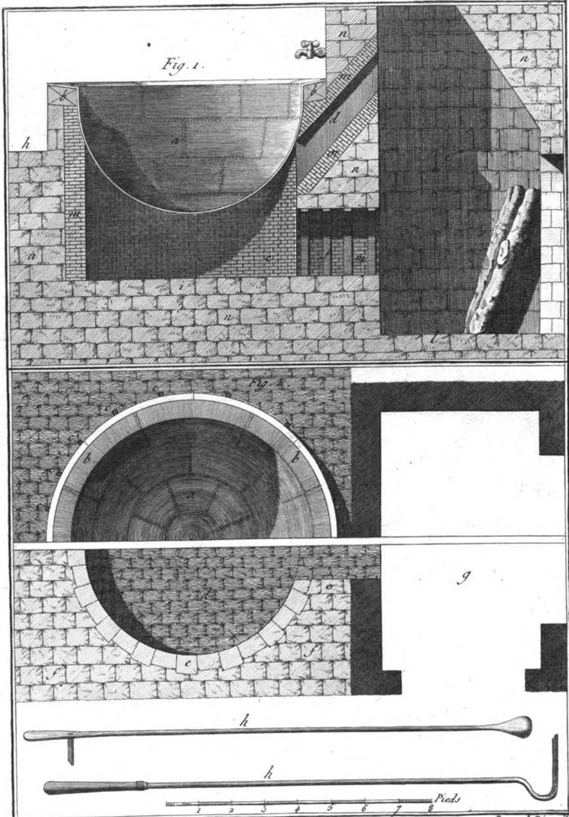
Teinture des Gobelins, Plans et Coupe d'un Fourneau, et Outils. 66. Bernard Dorez del.
