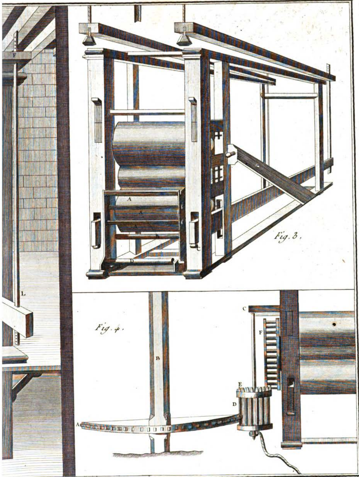
, Différentes Elevations du Cylindre à Bascules.
