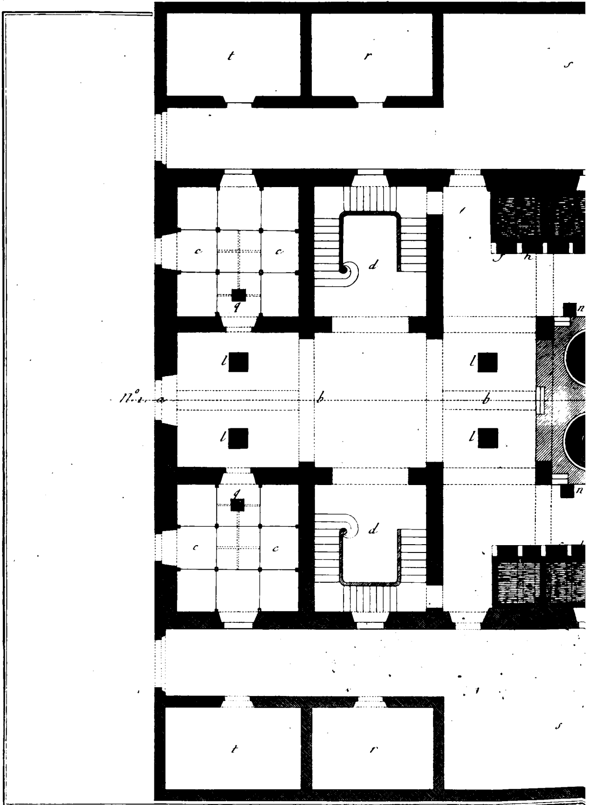
Savonnerie, Plan du Rez de Chaussée
