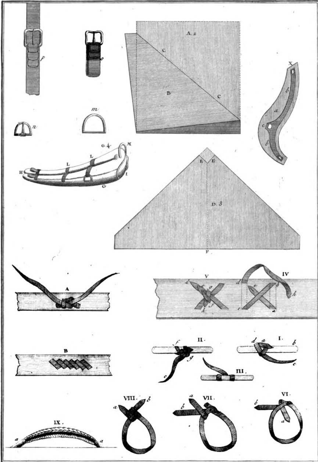
Sellier, suite du Travail du Bourrellier.
