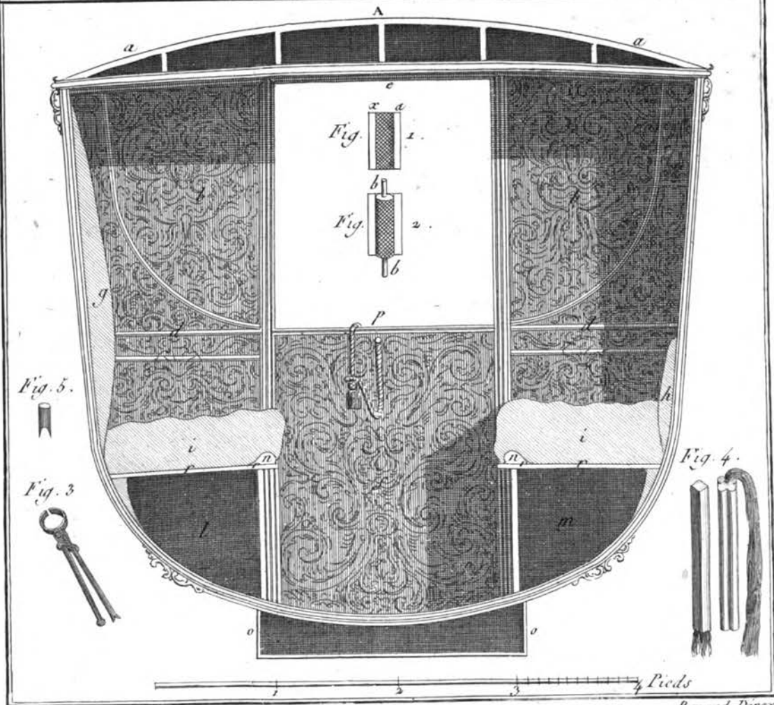
Sellier, Atelier du Sellier - Carrossier, Coupe d'une Berlina, &c.
