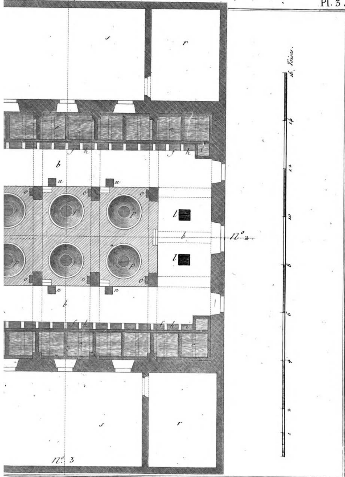
vue d'une Manufactory de Savon.
