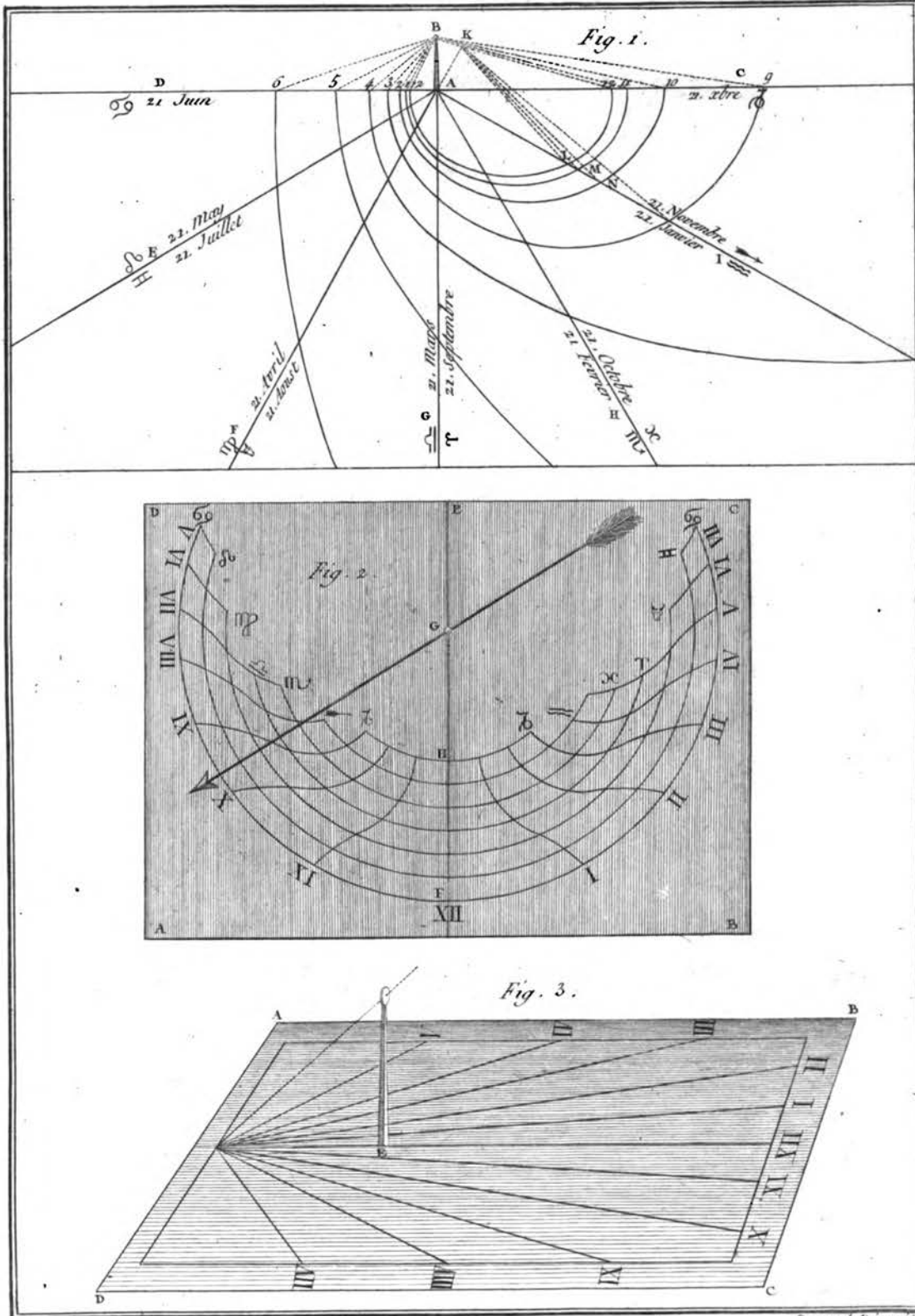
Amusemens de Gnomonique.
