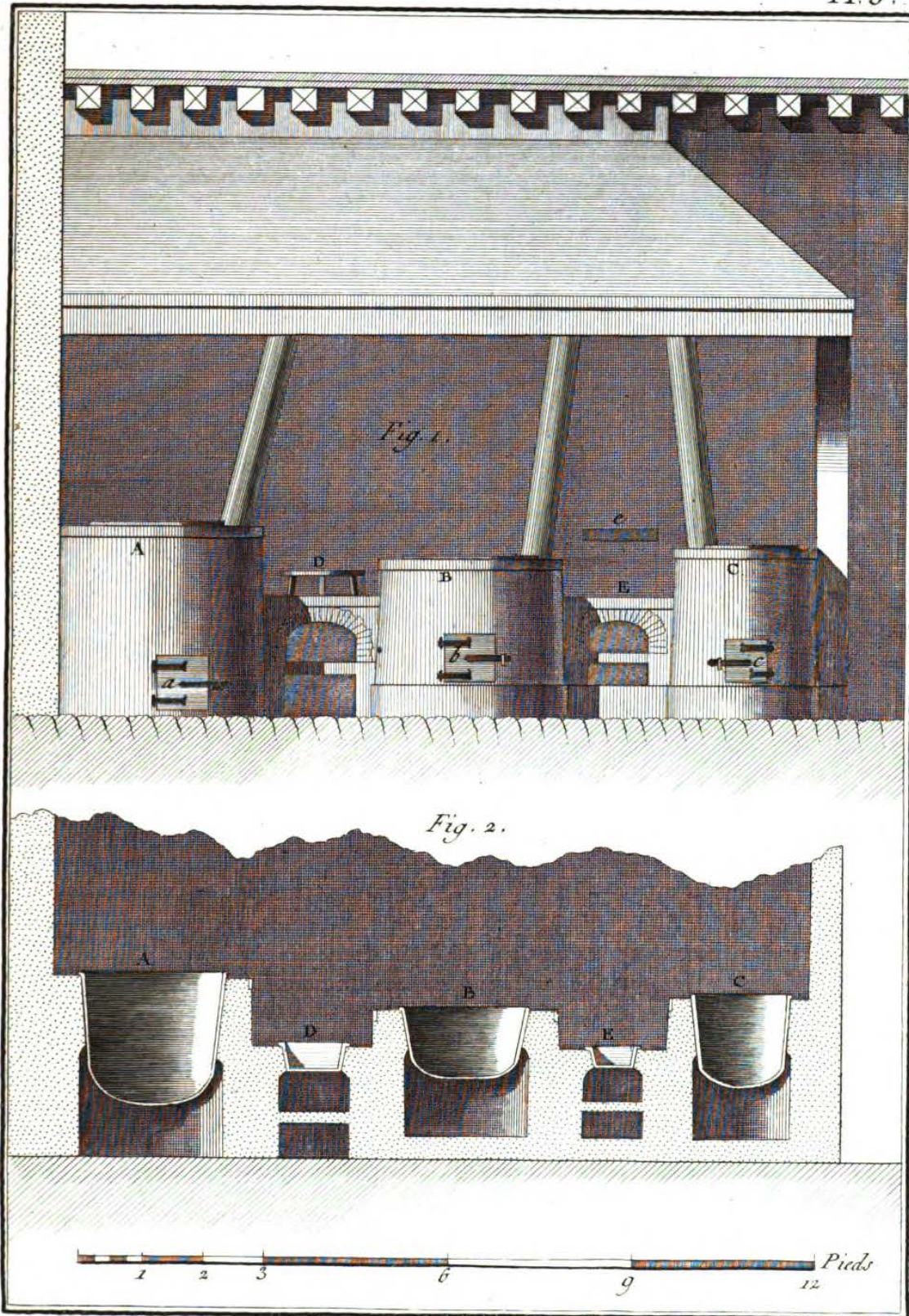
Maroquinier, Elevation et Coupe des Fourneaux.
