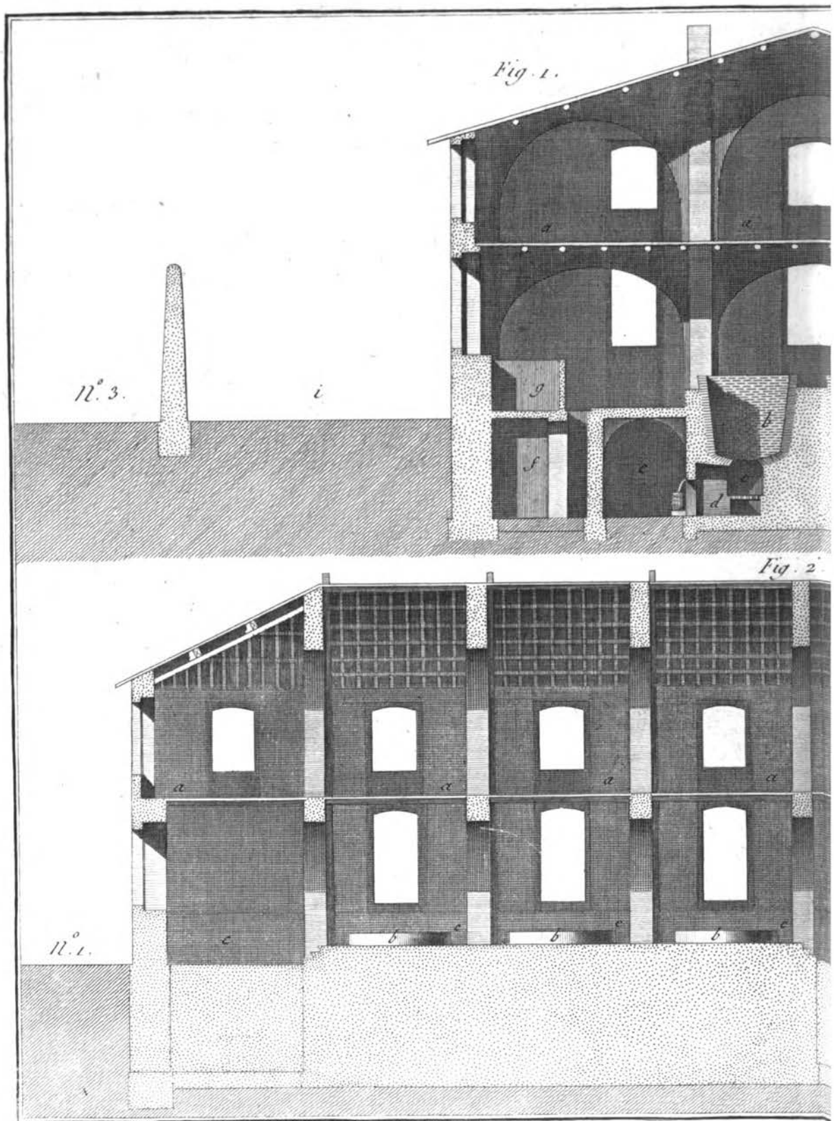
Savonnerie, Coupe sur la longueur et Coupe sur la largeur
