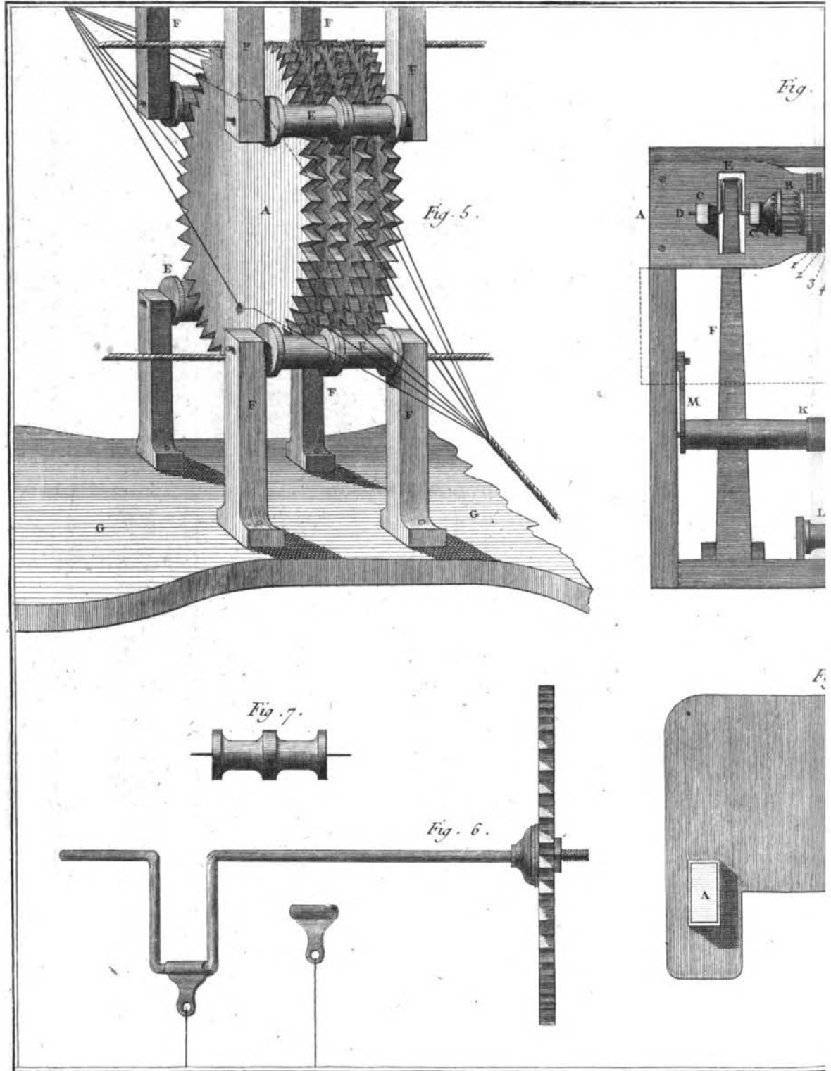
Machine nommée la Rave
