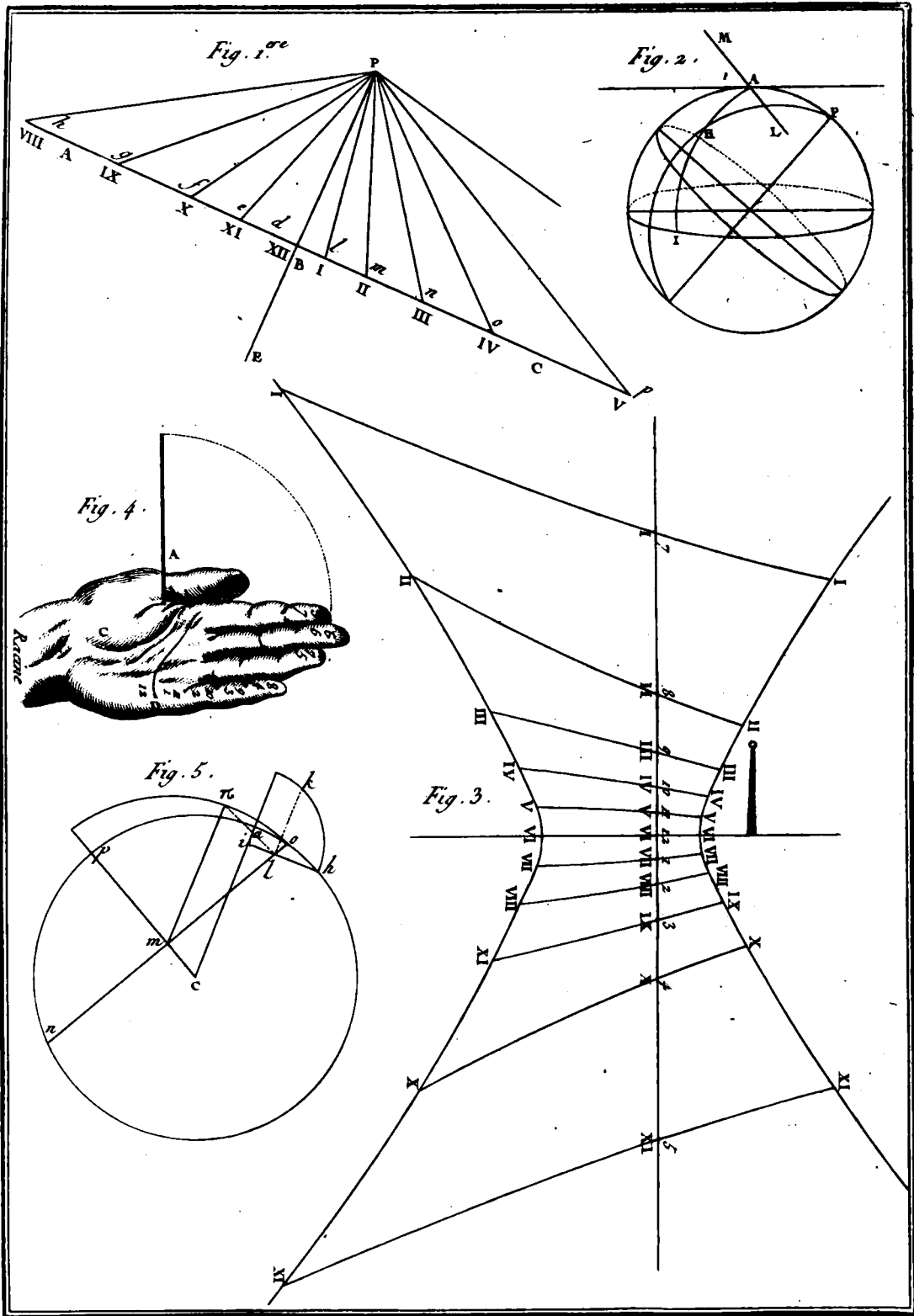
Amusemens de Gnomonique. Bernard Drexel.
