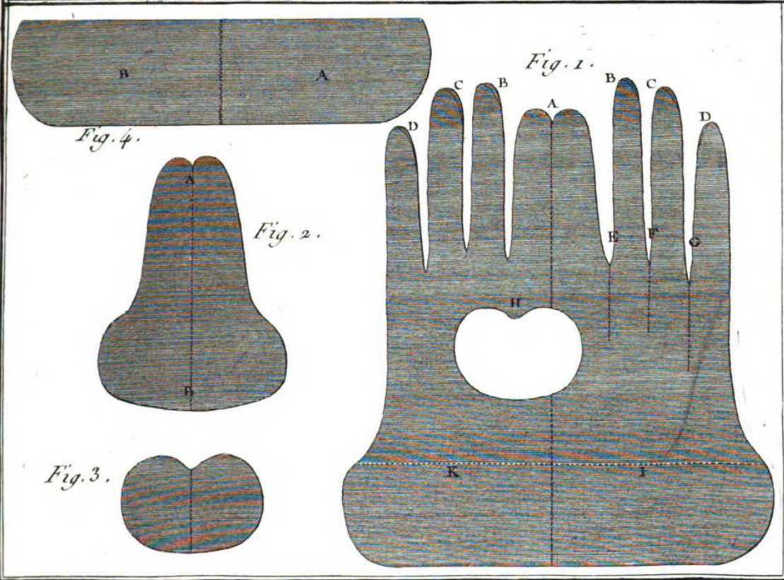
Ganterie, Etavillon et détails de Gants d'Hommes.
