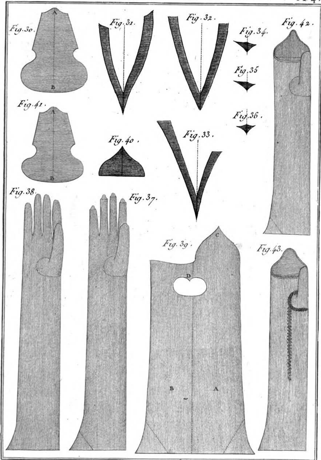
Gantier, Gants et Mitaines de Femmes.
