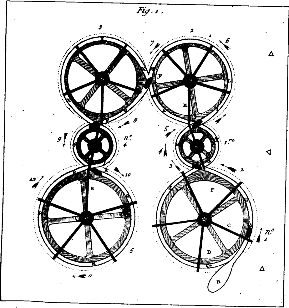
Machine à faire les Lacets.
