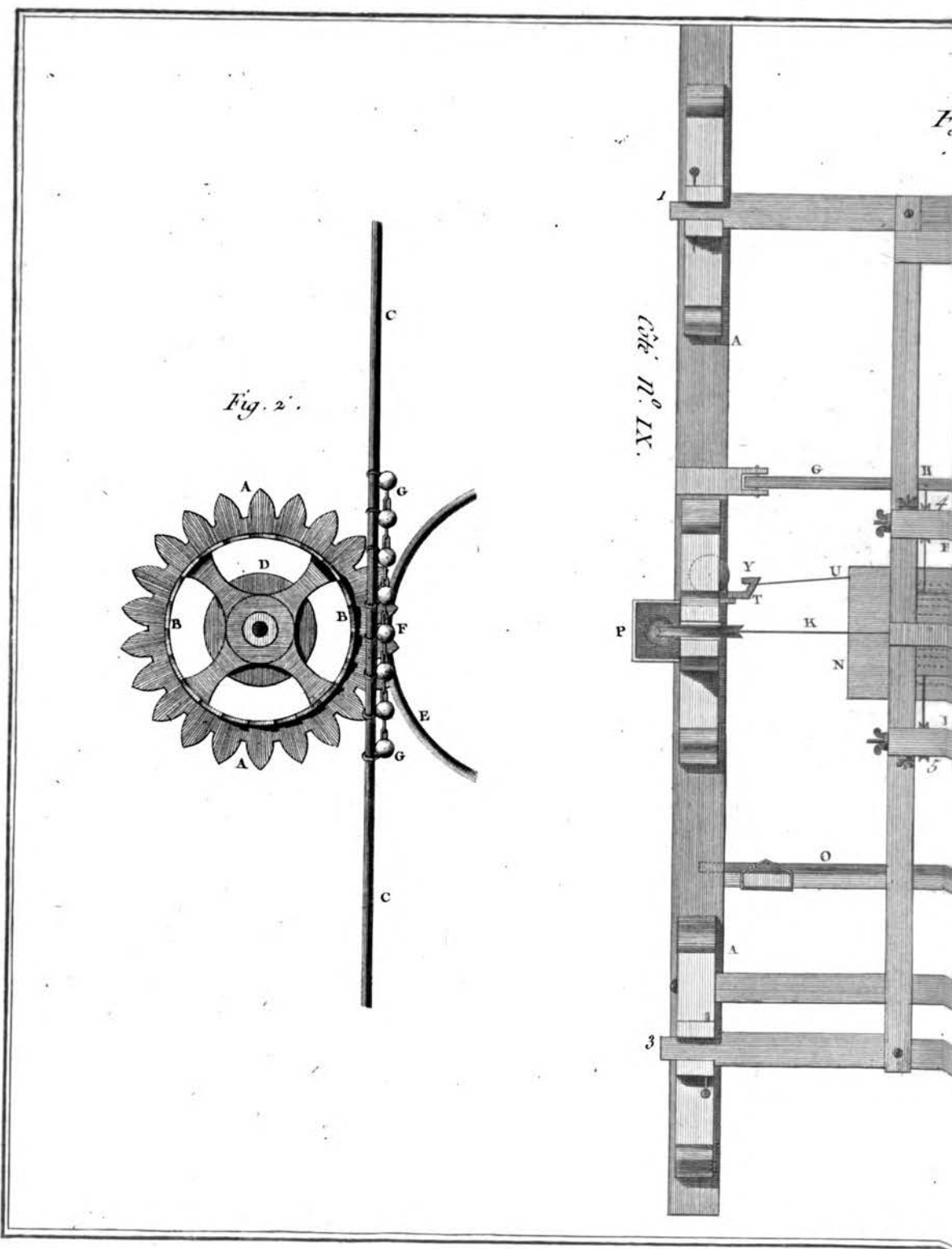
Plan de la Machine pour distiller
