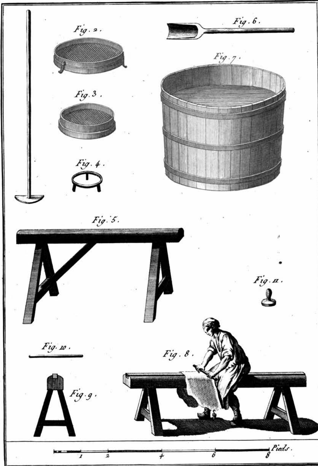
Maroquinier, ustensilles servant à la Teinture, et l'opération de Lisser le Maroquin. Benard Dircct.
