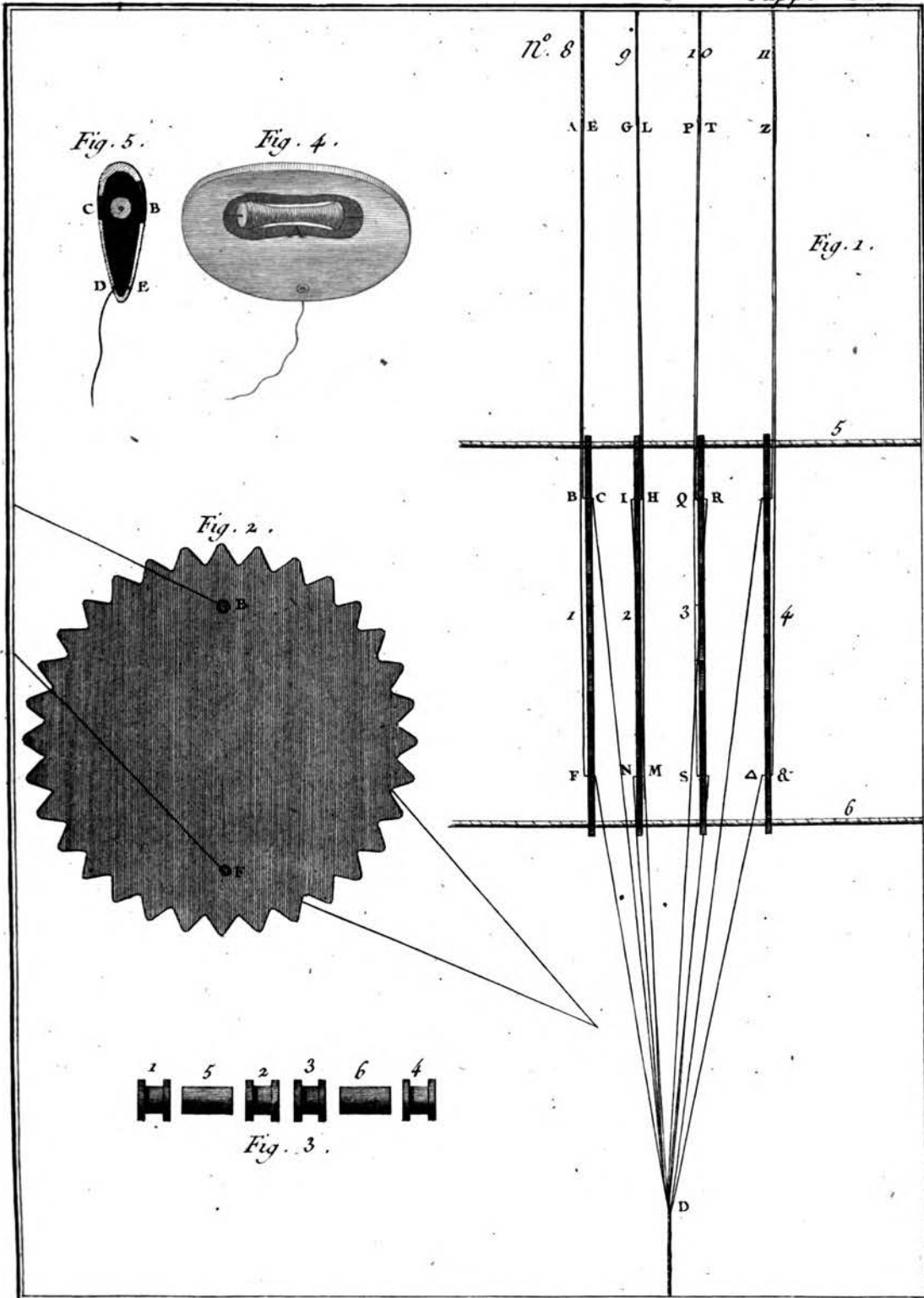
Développemens de la Machine nommée la Ratiere.
