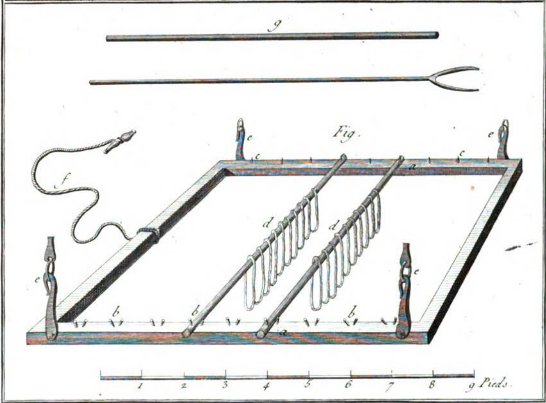
Teinturier, le sechoir pour les Soies &c.
