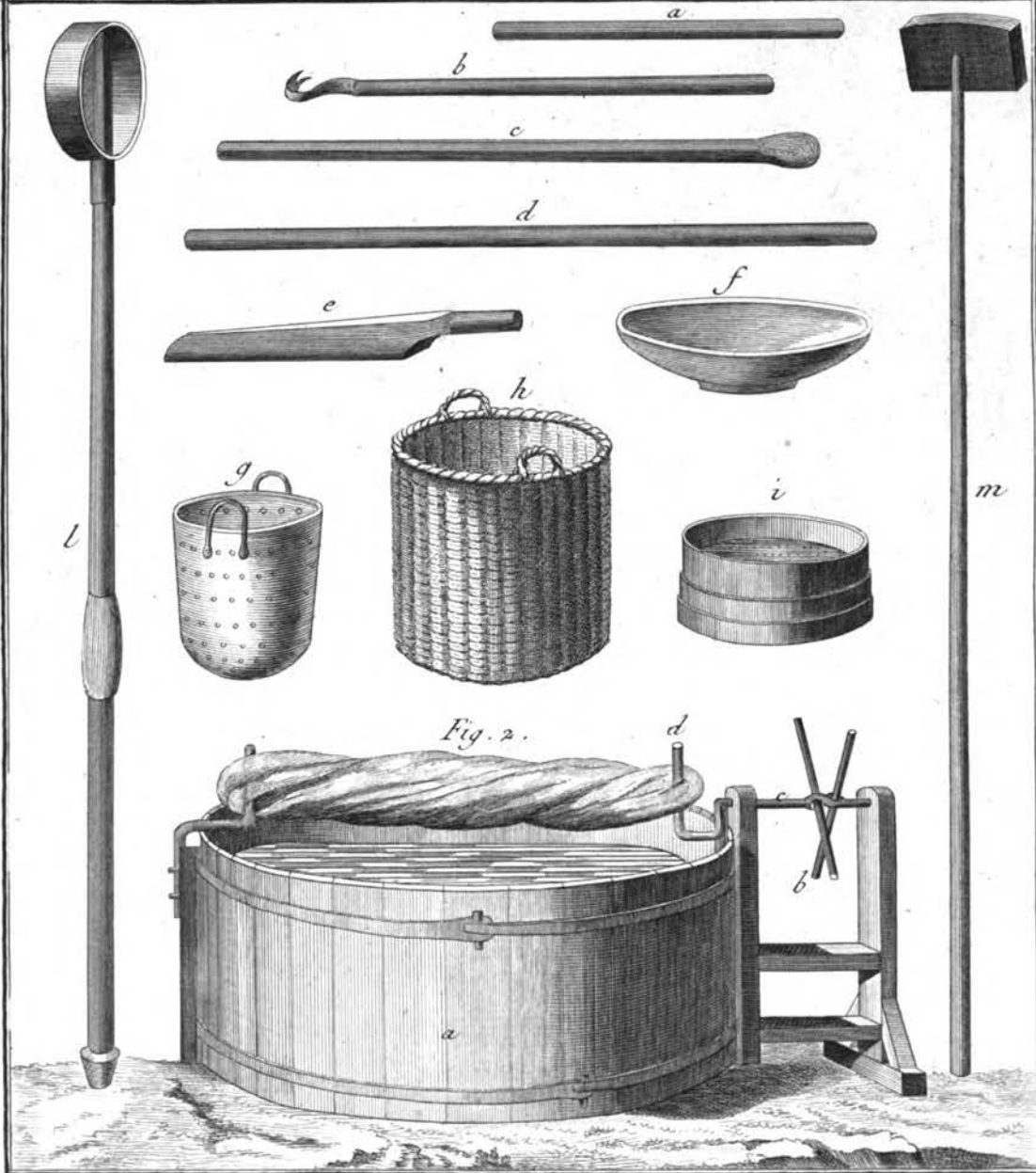
Teinture des Gobelins, Tordoir, Outils et Cuves.
