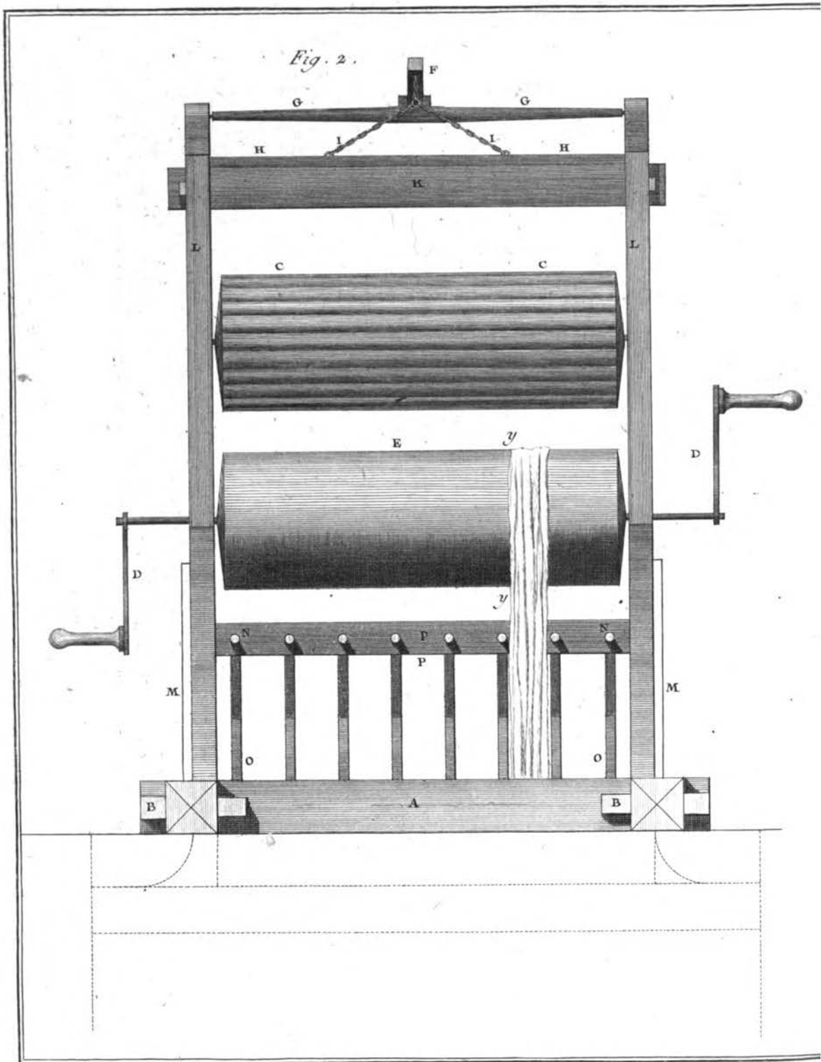
Machine à battre e
