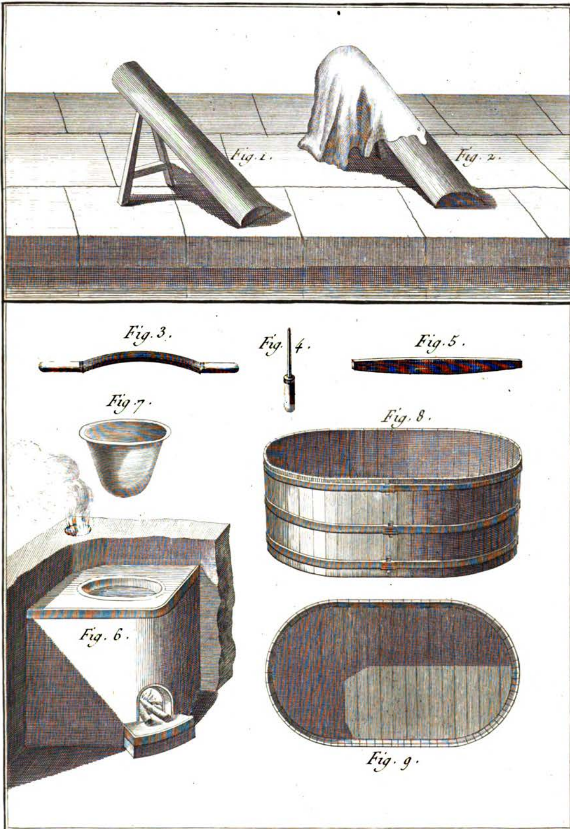
Hongroyeur, Travail de Riviere &c.
