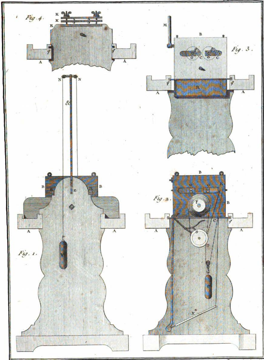
Machine à faire des Peignes.
