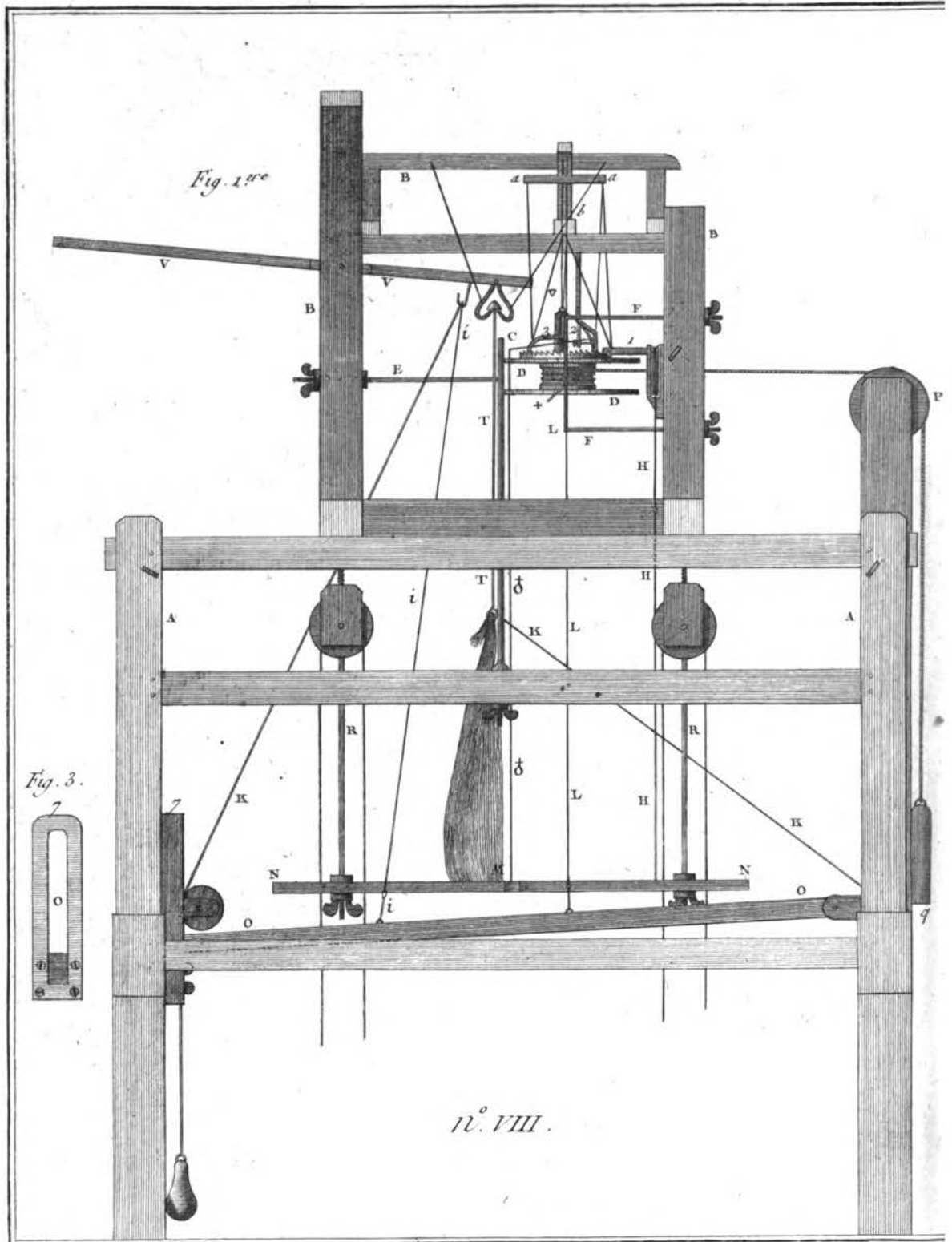
Élévation et Coupe de la Machine po
