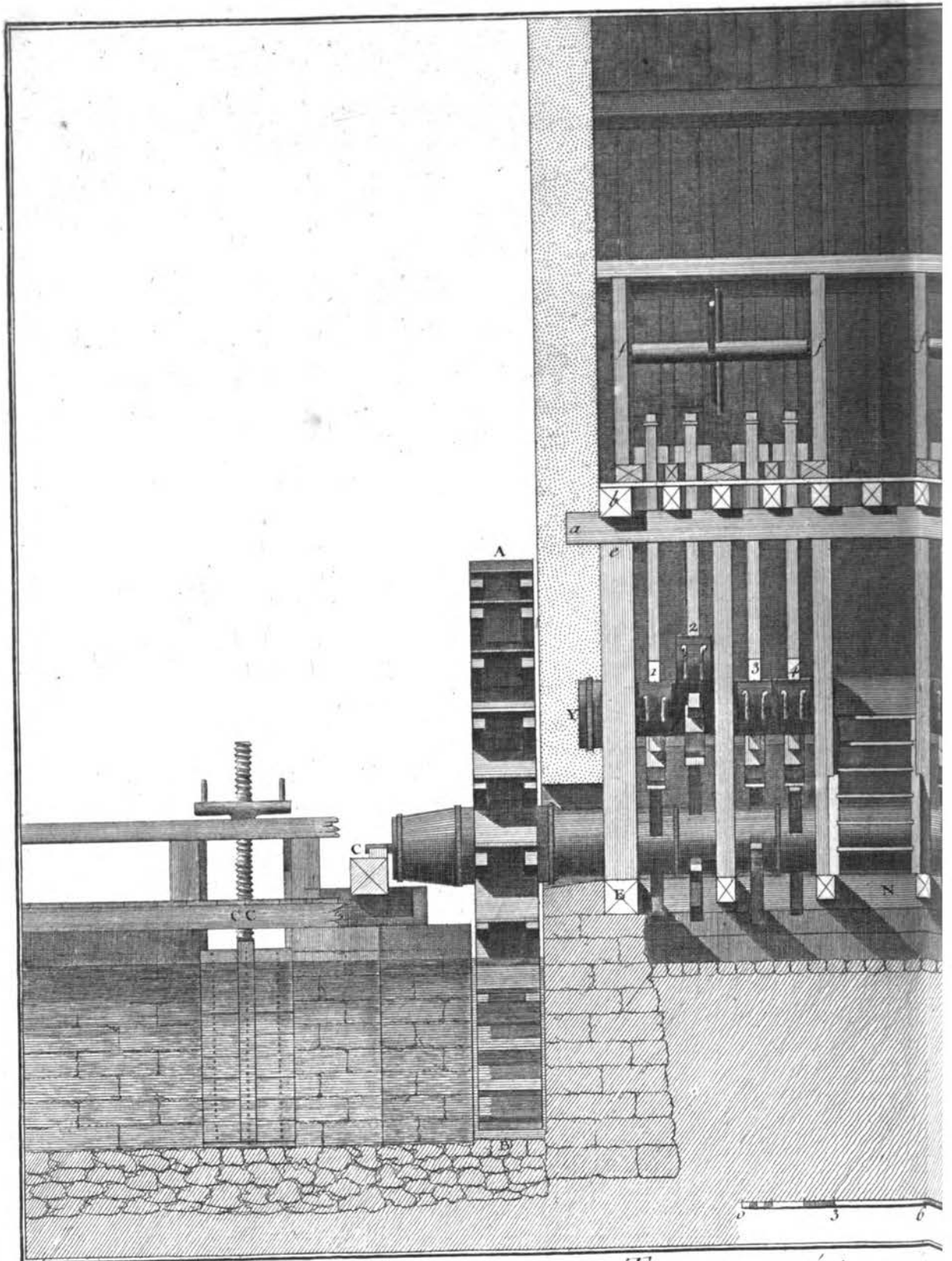
Tanneur, Élévation du
